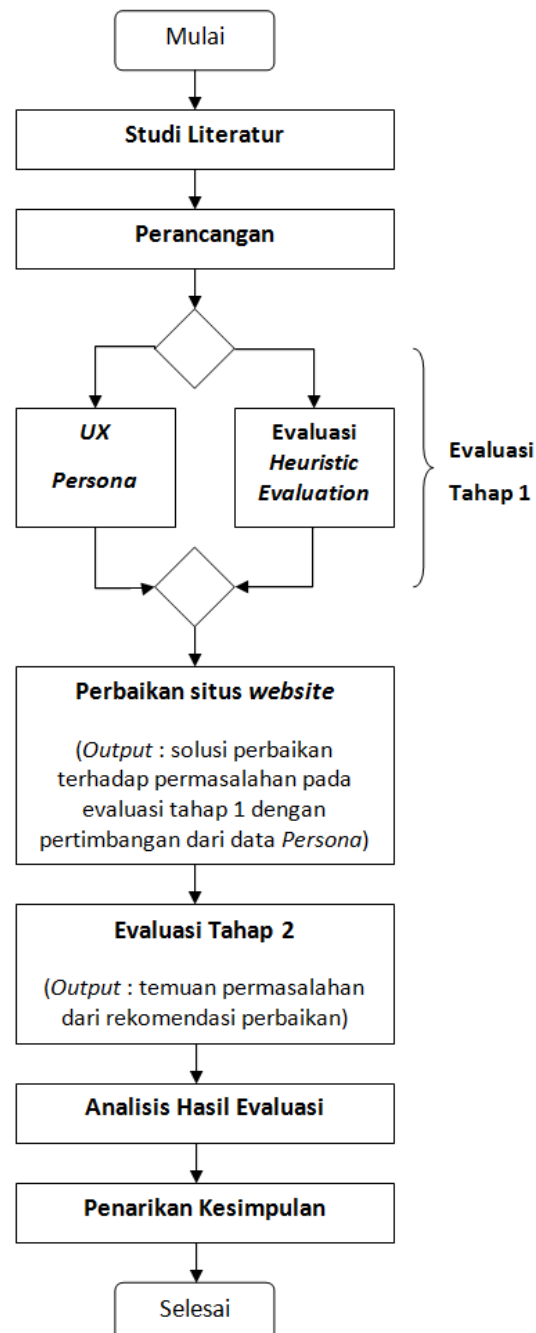
Gambar 3.1 Tahap penelitian
