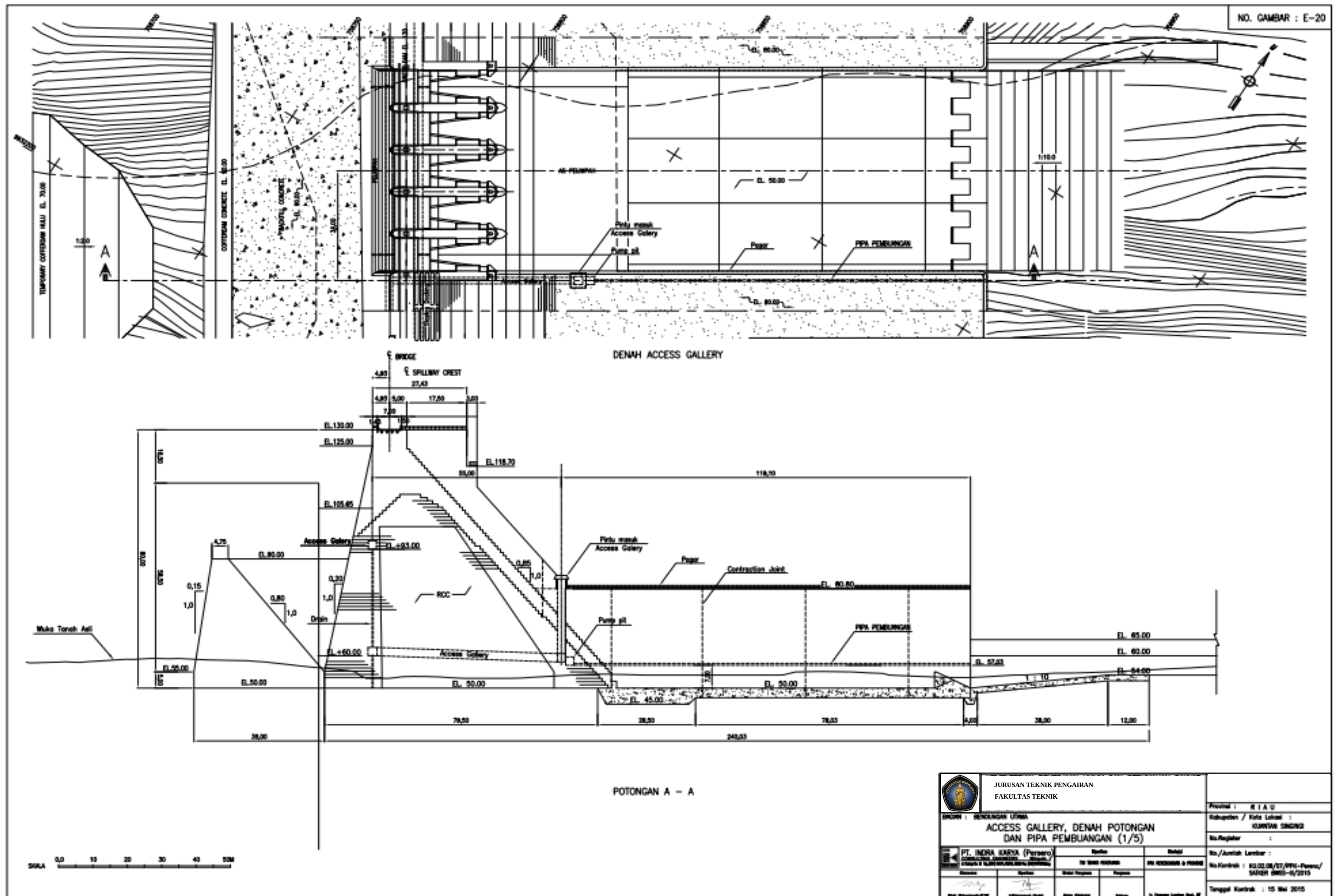
Gambar 3.5. Long Section Bendungan Lubuk Ambacang Sumber : Data PT. Indra Karya
