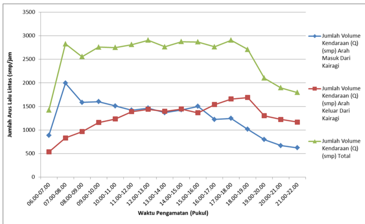
Gambar LI-3. Grafik Fluktuasi Volume Lalu Lintas Arah Masuk dan Keluar Kota Manado di Kairagi Hari Kamis
