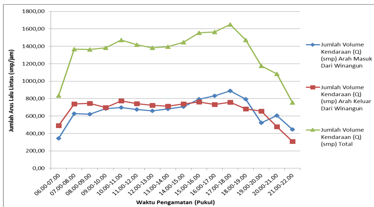
Gambar LI-9. Grafik Fluktuasi Volume Lalu Lintas Arah Masuk dan Keluar Kota Manado di Winangun hari Kamis
