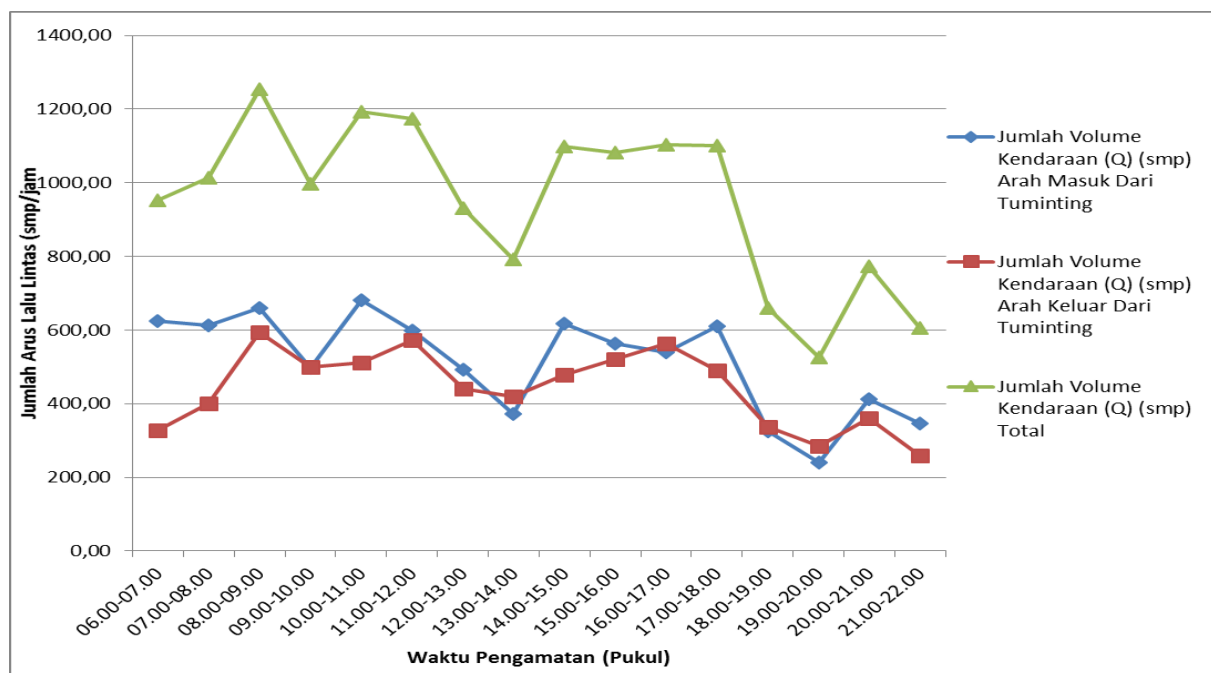
Gambar LI-15. Grafik Fluktuasi Volume Lalu Lintas Arah Masuk dan Keluar Kota Manado di Tuminting Hari Kamis
