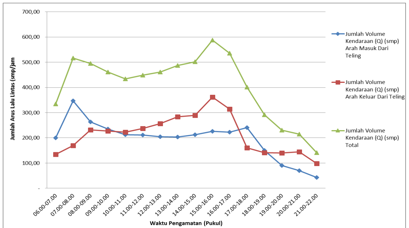
Gambar LI-6. Grafik Fluktuasi Volume Lalu Lintas Arah Masuk dan Keluar Kota Manado di Teling hari Kamis
