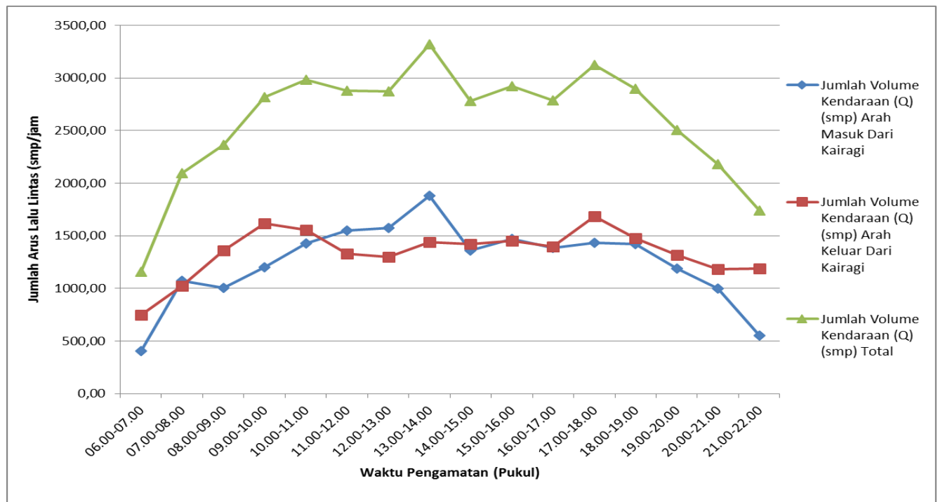
Gambar L 2. Grafik Fluktuasi Volume Lalu Lintas Arah Masuk dan Keluar Kota Manado di Kairagi Hari Rabu
