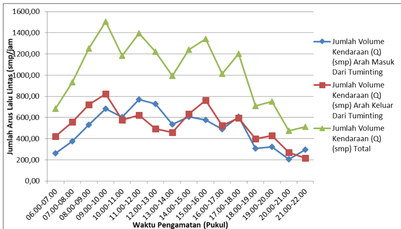
Gambar LI-13. Grafik Fluktuasi Volume Lalu Lintas Arah Masuk dan Keluar Kota Manado di Tuminting Hari Senin
