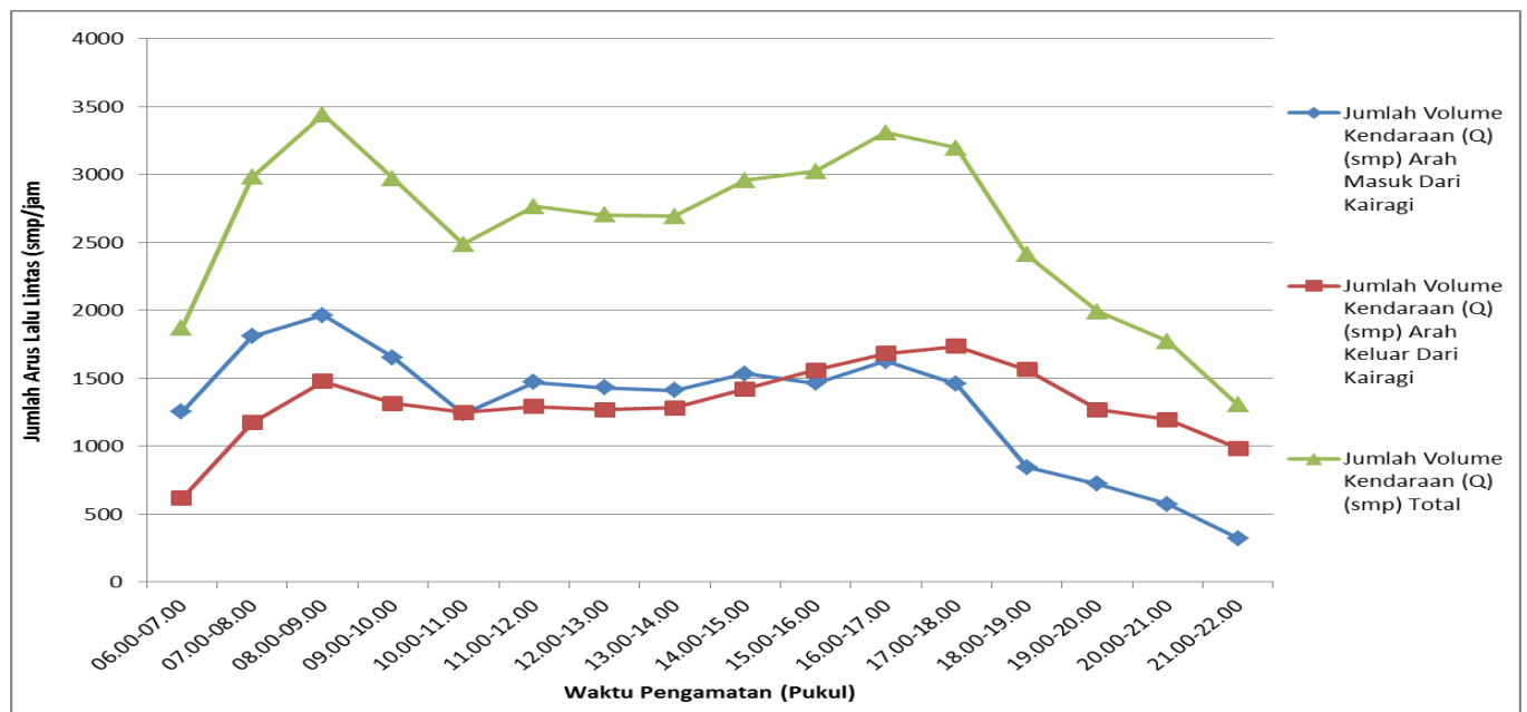
Gambar LI-1 Grafik Fluktuasi Volume Lalu Lintas Arah Masuk dan Keluar Kota Manado di Kairagi Hari Senin
