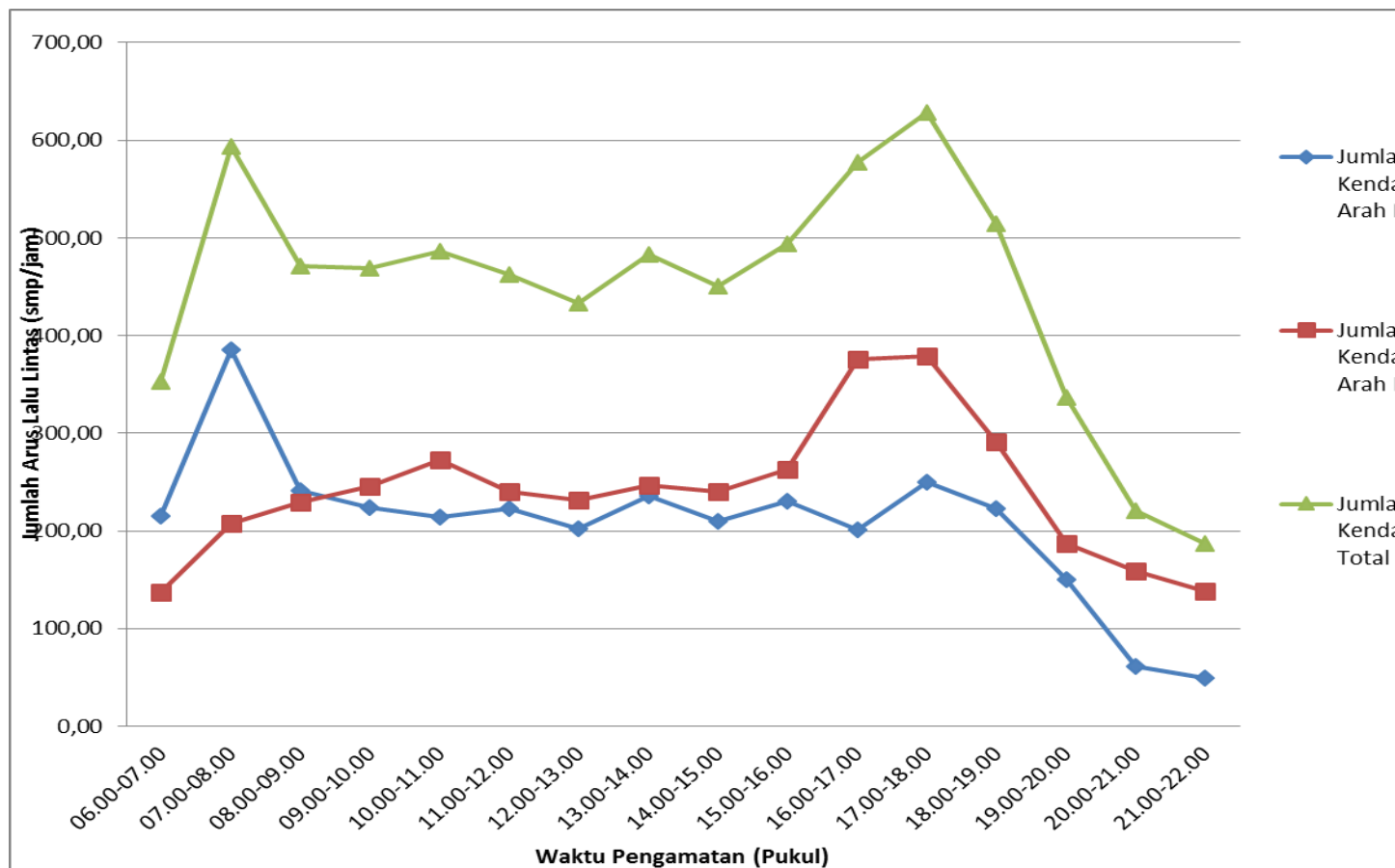
Gambar LI-5. Grafik Fluktuasi Volume Lalu Lintas Arah Masuk dan Keluar Kota Manado di Teling hari Rabu
