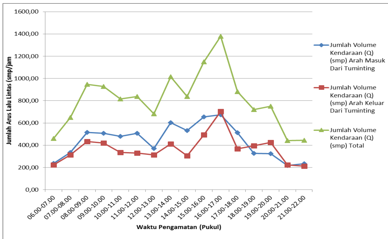
Gambar LI-14. Grafik Fluktuasi Volume Lalu Lintas Arah Masuk dan Keluar Kota Manado di Tuminting Hari Rabu
