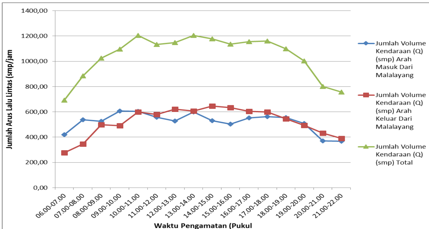
Gambar LI-12. Grafik Fluktuasi Volume Lalu Lintas Arah Masuk dan Keluar Kota Manado di Malalayang Hari Kamis
