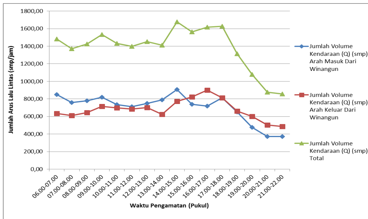
Gambar LI-7. Grafik Fluktuasi Volume Lalu Lintas Arah Masuk dan Keluar Kota Manado di Winangun hari Senin
