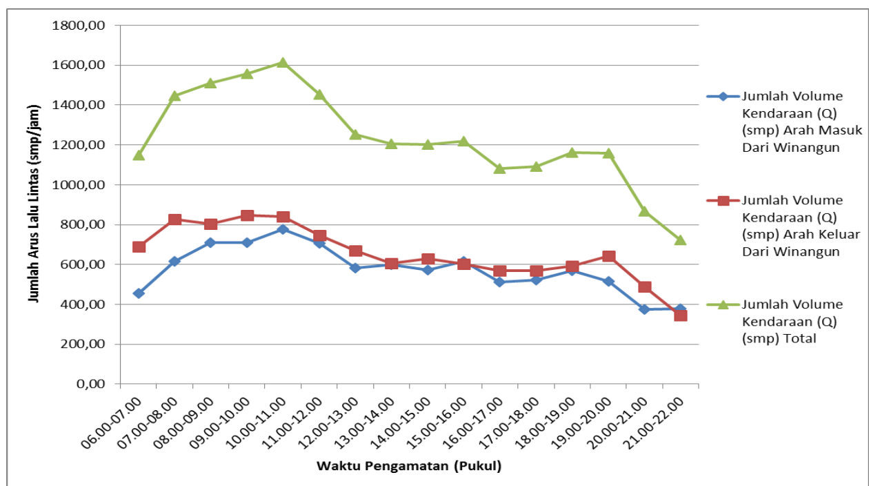
Gambar LI-8. Grafik Fluktuasi Volume Lalu Lintas Arah Masuk dan Keluar Kota Manado di Winangun hari Rabu
