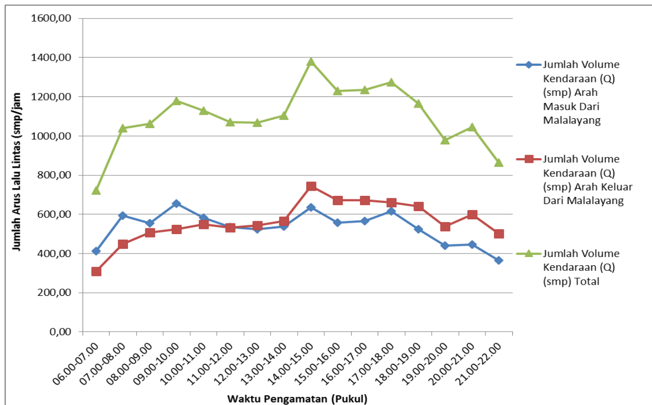
Gambar LI-10. Grafik Fluktuasi Volume Lalu Lintas Arah Masuk dan Keluar Kota Manado di Malalayang Hari Senin
