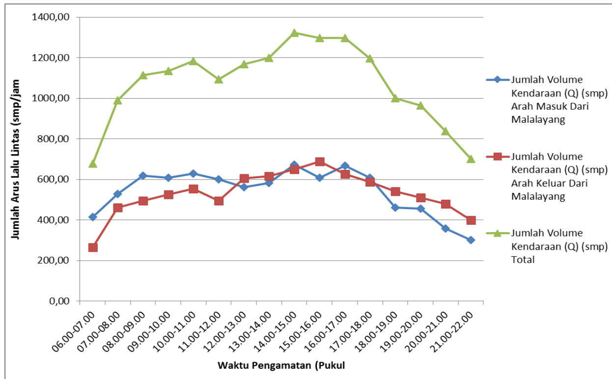
Gambar LI-11. Grafik Fluktuasi Volume Lalu Lintas Arah Masuk dan Keluar Kota Manado di Malalayang Hari Rabu
