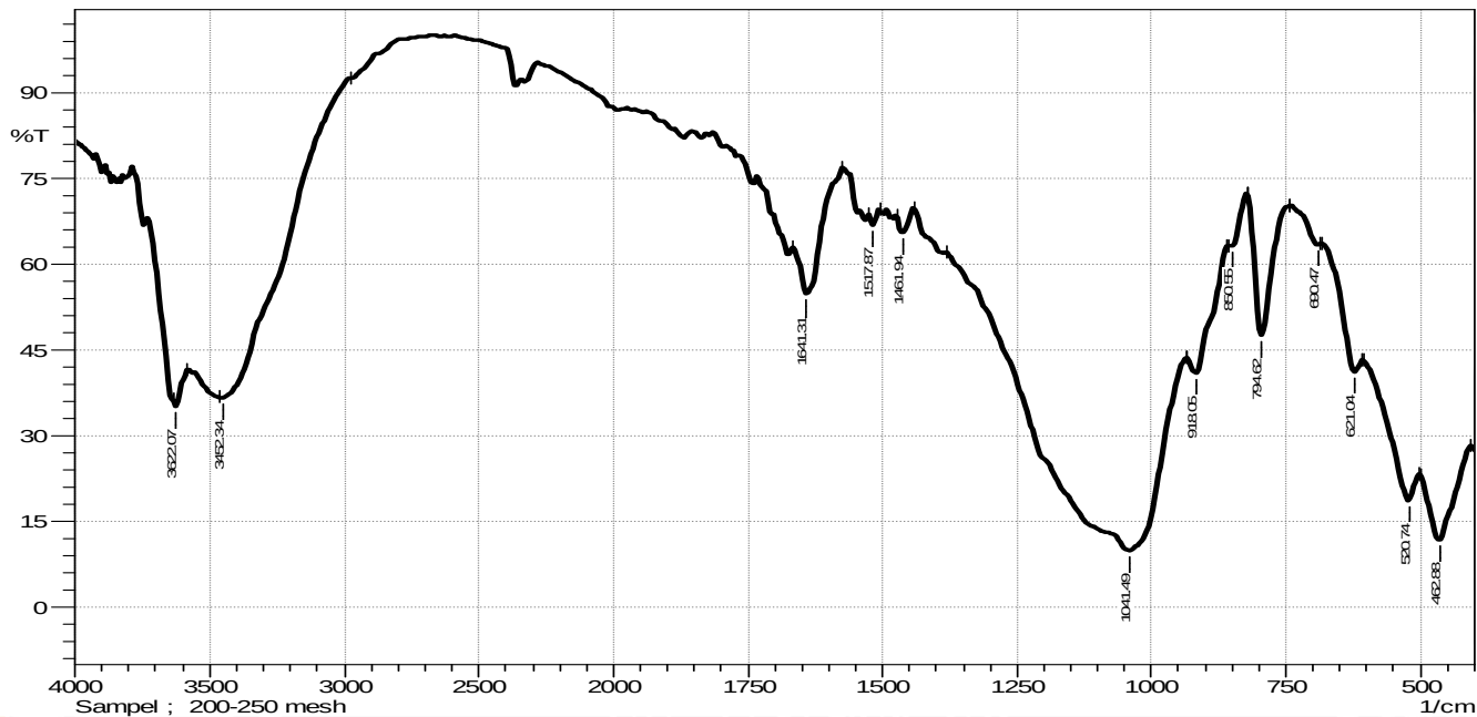
Gambar L.6.1 Spektra Inframerah Bentonit Natrium 200-250 mesh
