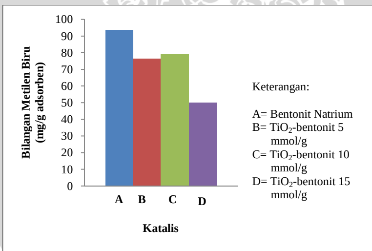
Gambar 4.5 Grafik Bilangan Metilen Biru Akibat Impregnasi dengan TiO 2
