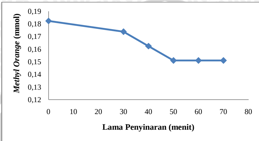
Gambar 4.1 Pengaruh Lama Penyinaran UV terhadap Konsentrasi Methyl Orange pada Konsentrasi Awal Zat Warna Methyl Orange 60 ppm
