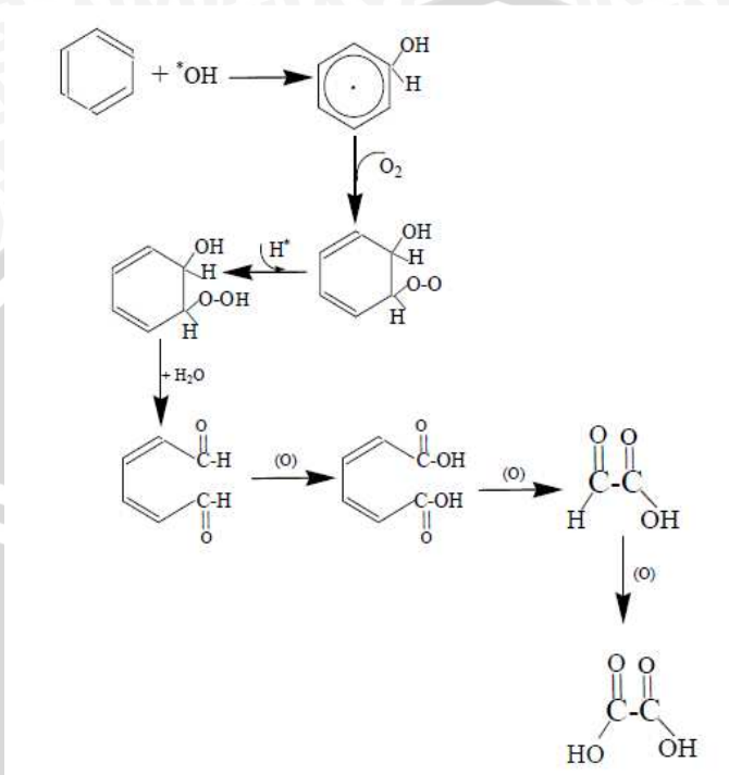
Gambar 2.8 Tahap Reaksi Degradasi Gugus Benzene (Getoff, 1996)
