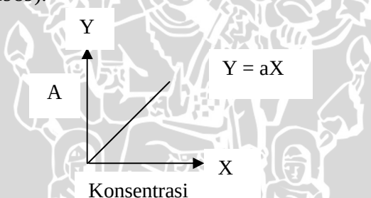
Gambar 2.9 Kurva Hubungan Absorbansi dengan Konsentrasi
