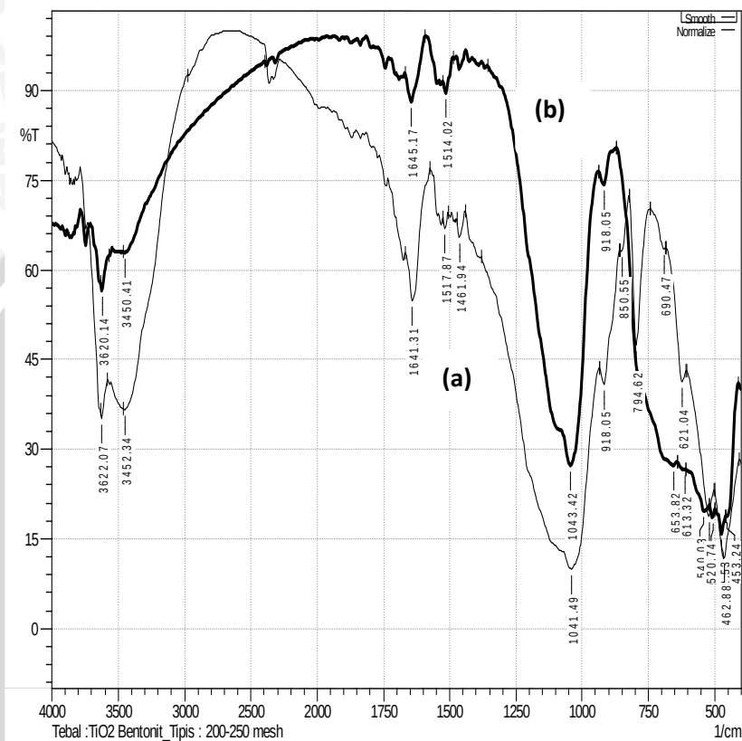
Gambar 4.6 Spektra Inframerah (a) Bentonit Natrium (b) \text{TiO}_2 -Bentonit 10 mmol/katalis optimum
