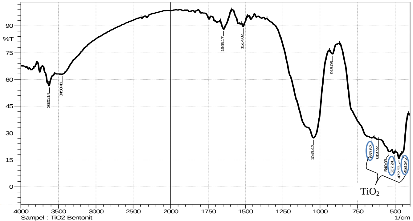
Gambar L.6.2 Spektra Inframerah TiO 2 -Bentonit 10 mmol/g (Katalis Optimum)
