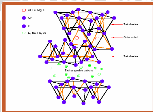
Gambar 2.3 Struktur Bentonit (Syuhada dkk. , 2009)
