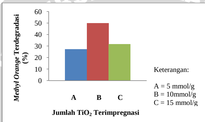
Gambar 4.3 Pengaruh Jumlah Konsentrasi \text{TiO}_2 yang Terimpregnasi terhadap Persen Methyl Orange Terdegradasi pada Konsentrasi Larutan Methyl Orange 20 ppm dan Lama Penyinaran 50 Menit
