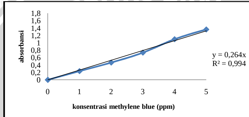
Gambar L.5.2 Kurva Baku Larutan Metilen Biru
