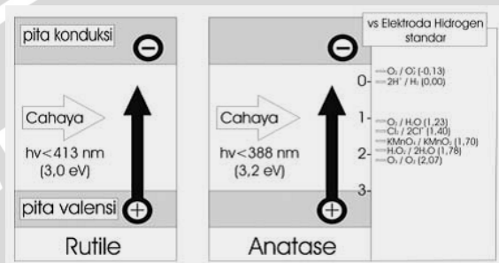
Gambar 2.2 Celah Pita Energi \text{TiO}_2 Rutil dan Anatase serta Hubungannya dengan Potensial Redoks (Gunadi, 2008)
