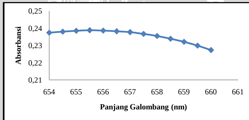
L.5.1 Grafik Penentuan Panjang Gelombang Maksimum Metilen Biru
