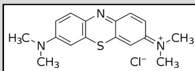
Gambar 2.10 Struktur Molekul Metilen Biru
