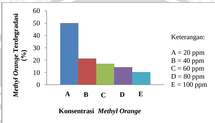
Gambar 4.2 Persen Methyl Orange Terdegradasi terhadap Konsentrasi Larutan Methyl Orange pada Lama Penyinaran Sinar UV 50 Menit
