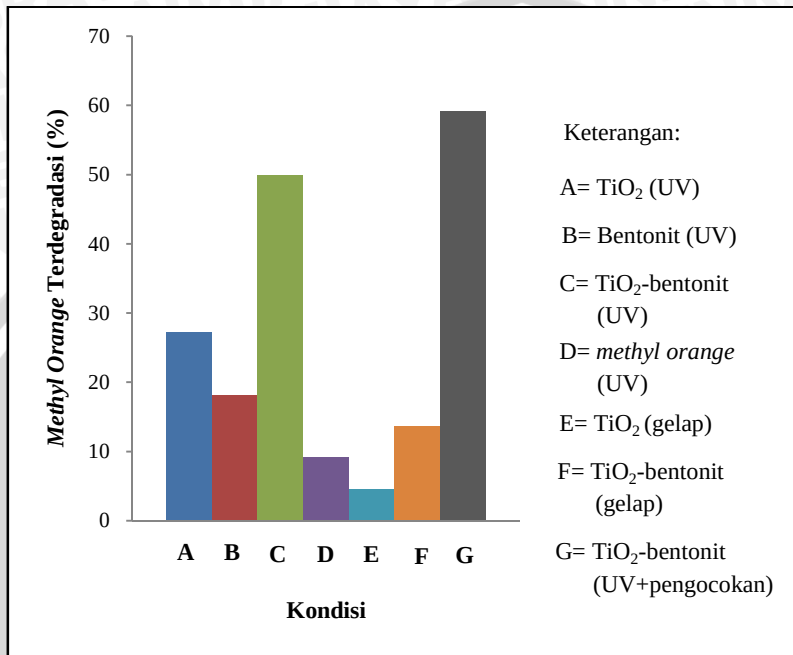
Gambar 4.4 Perbandingan Kemampuan Degradasi Zat Warna Methyl Orange 20 ppm pada Lama Penyinaran 50 Menit
