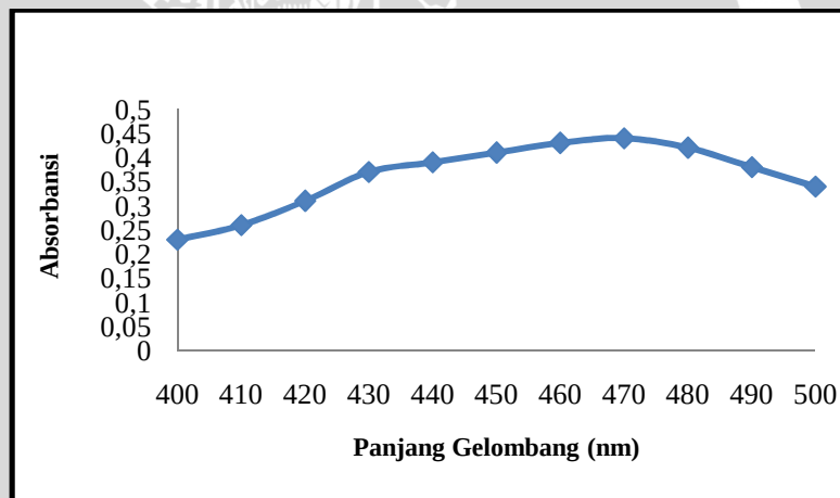
Gambar L.3.1 Grafik Penentuan Panjang Gelombang Maksimum Methyl Orange
