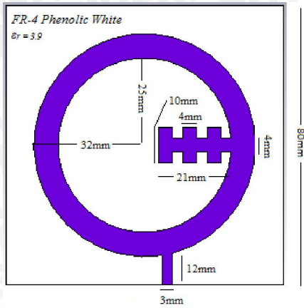
Gambar 1. Bentuk Geometri Antena Mikrostrip: Sumber: Simulasi
