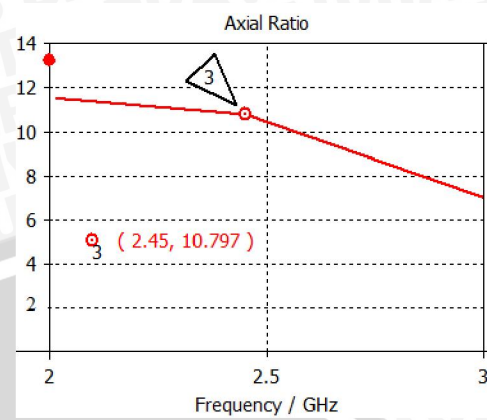
Grafik 2. Nilai Axial Ratio terhadap frekuensi pada antena
