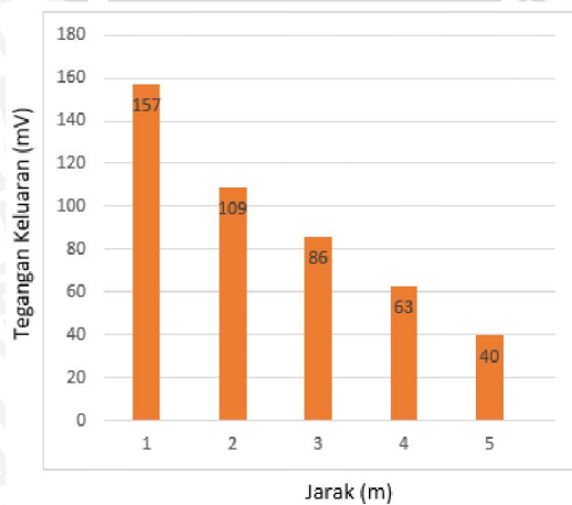
Grafik 5. Hasil Tegangan Keluaran Switch Rectenna Sumber : Hasil Pengujian
