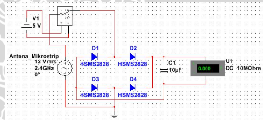
Gambar 2. Rancangan switch rectifier
