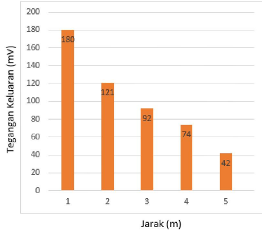
Grafik 4. Hasil Tegangan Keluaran Rectenna Sumber : Hasil Pengukuran
