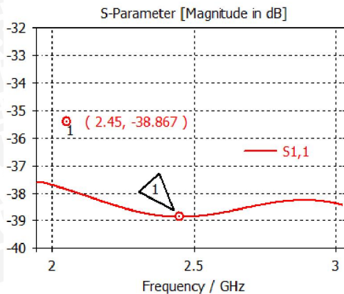
Grafik 1. Nilai Return Loss terhadap frekuensi pada antena
