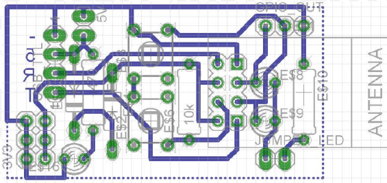
Gambar 4. Jalur kaki rancangan modul ESP8266
