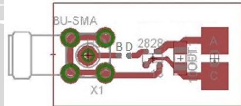
Gambar 3. Jalur kaki rancangan rectifier
