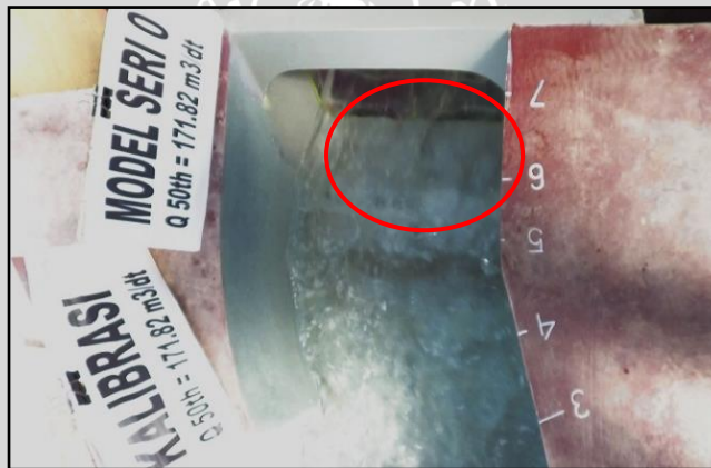
Kondisi aliran debit Q_{50} pada saluran transisi menuju ke saluran peluncur
