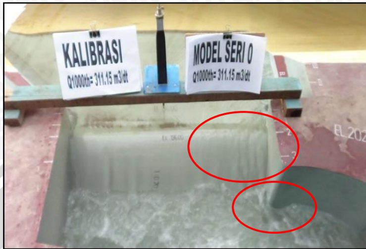
Kondisi aliran debit Q_{1000} pada pelimpah tampak depan
