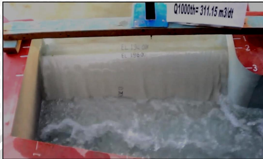
Kondisi aliran debit Q_{1000} pada pelimpah tampak depan seri 1
