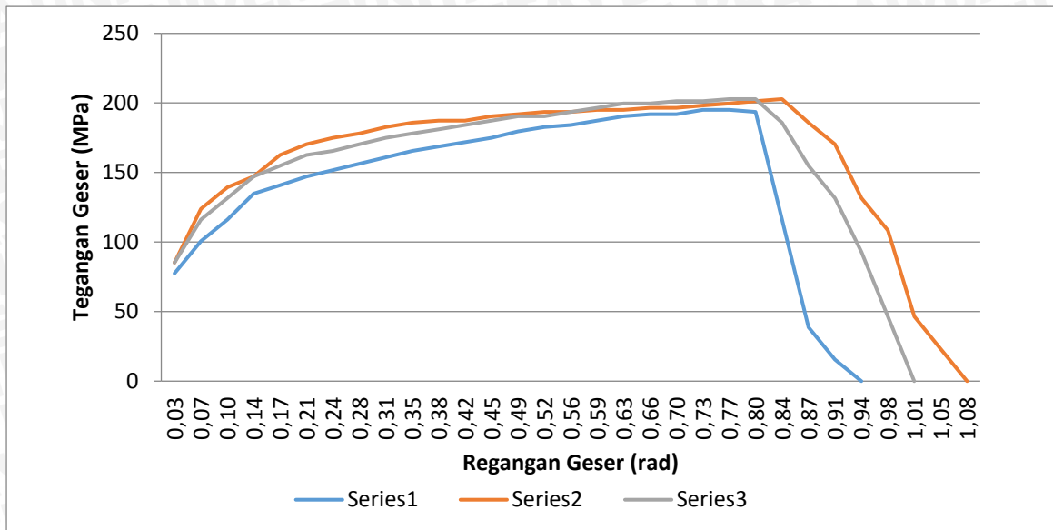
Spesimen sudut chamfer 30° BOL 15 mm
