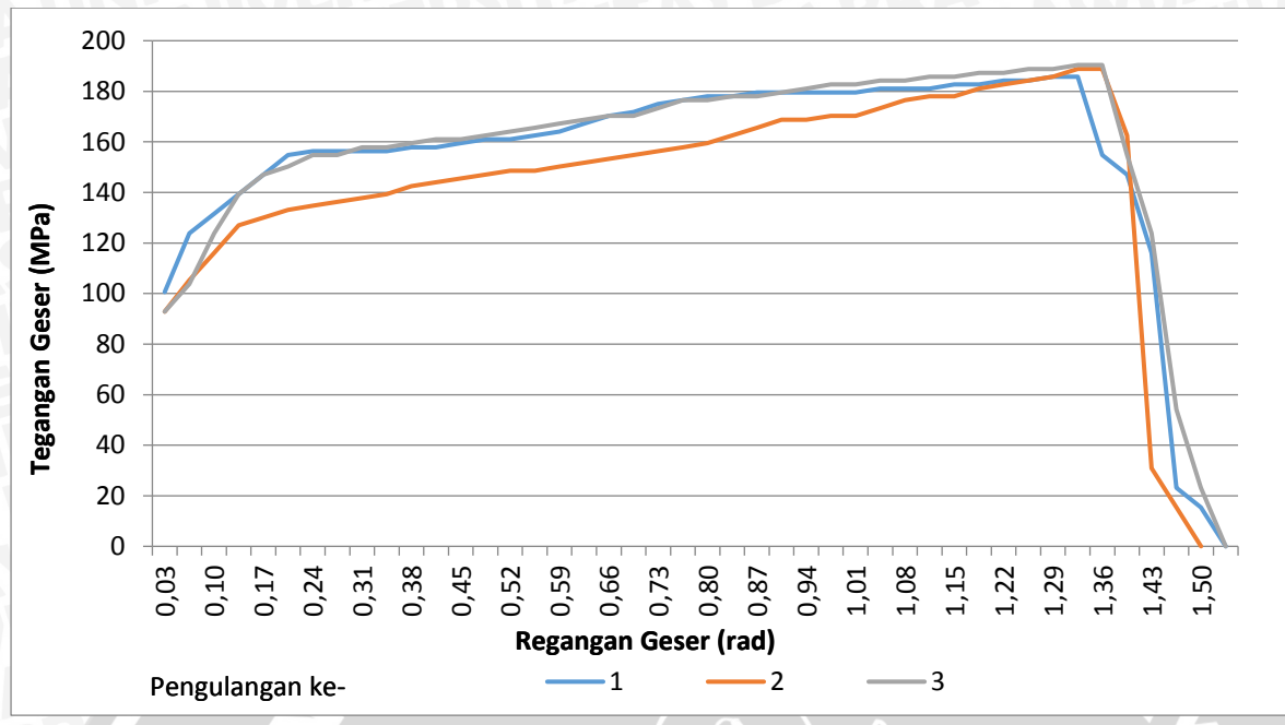
Spesimen sudut chamfer 0° BOL 20 mm
