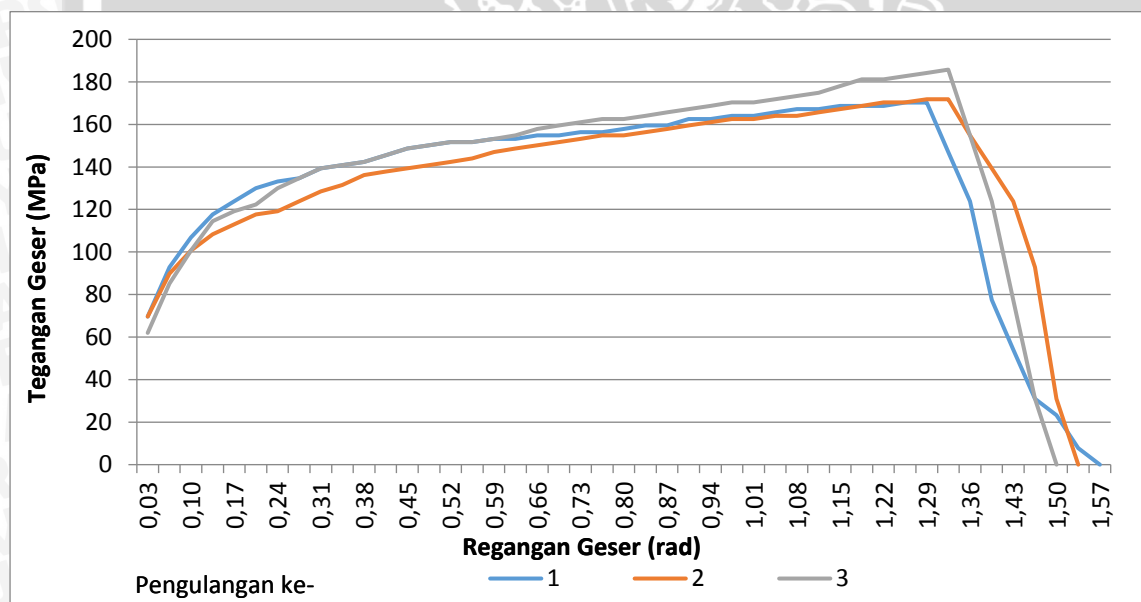
Spesimen sudut chamfer 0° BOL 15 mm
