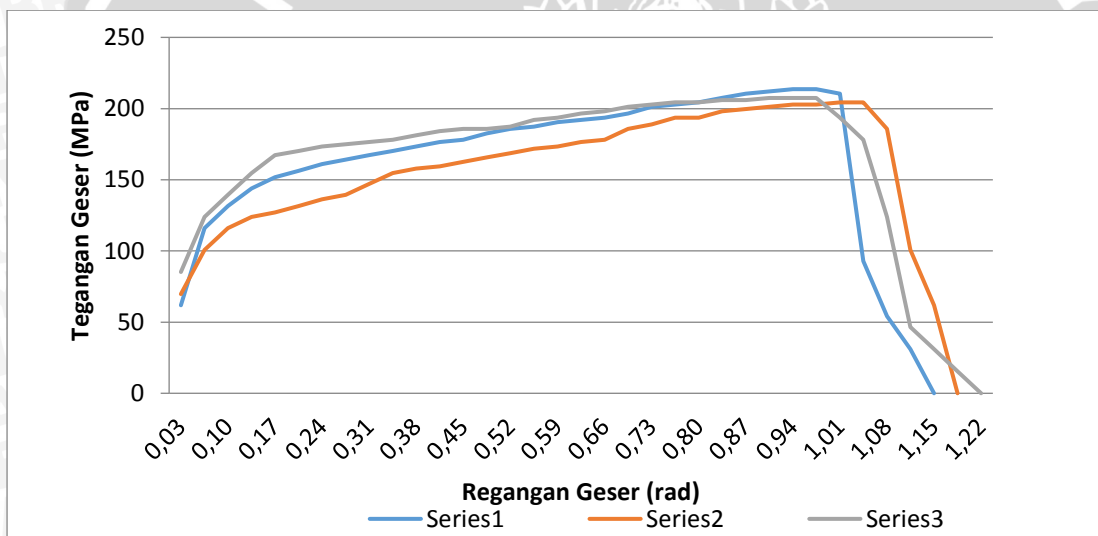
Spesimen sudut chamfer 30° BOL 20 mm
