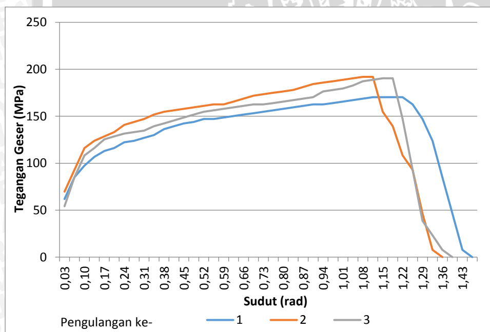
Spesimen sudut chamfer 60° BOL 20 mm
