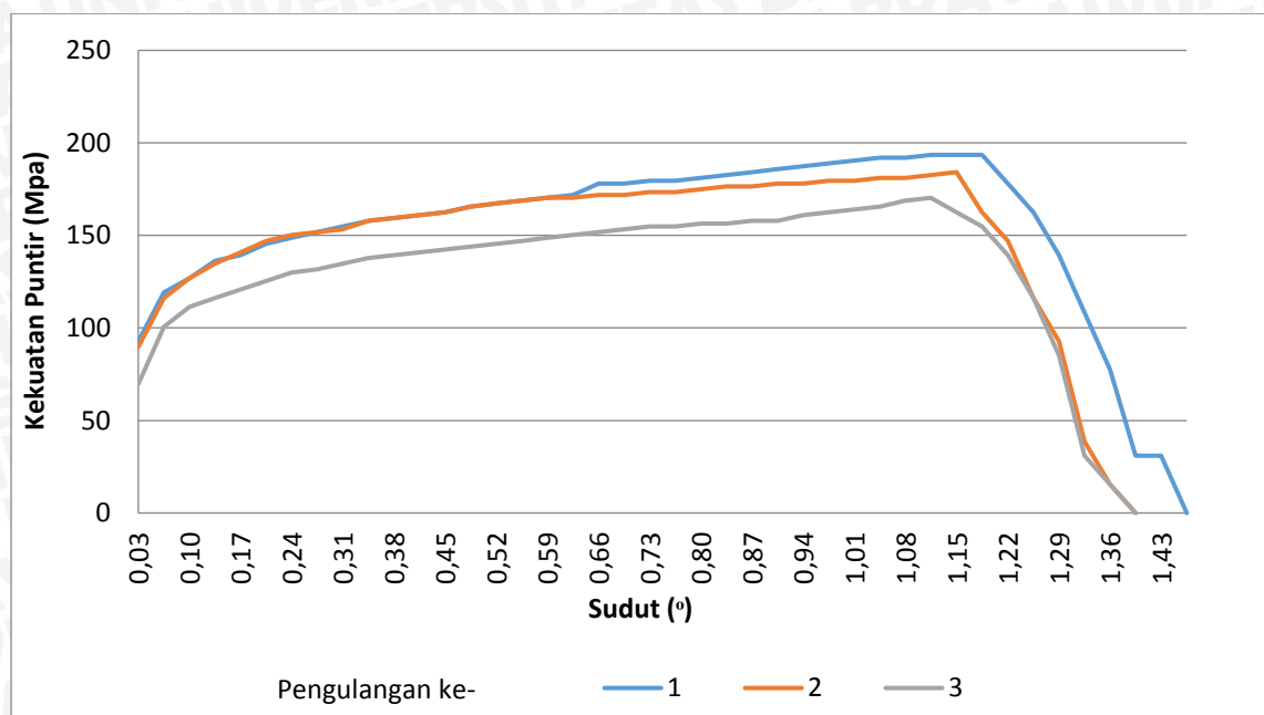
Spesimen sudut chamfer 0° BOL 10 mm
