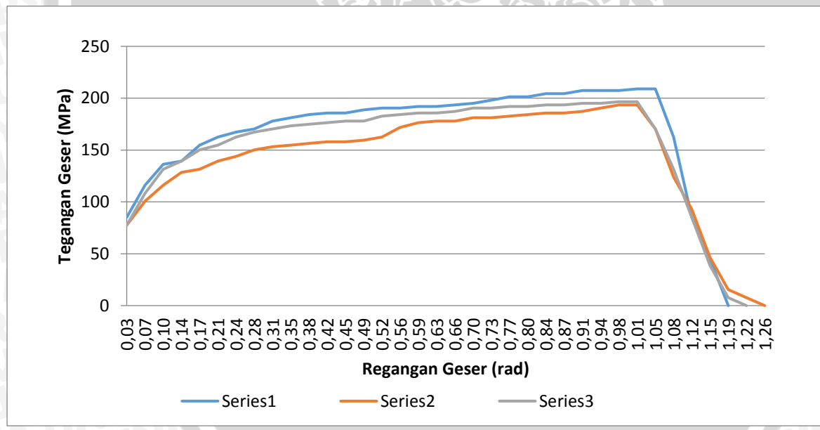
Spesimen sudut chamfer 30° BOL 10 mm
