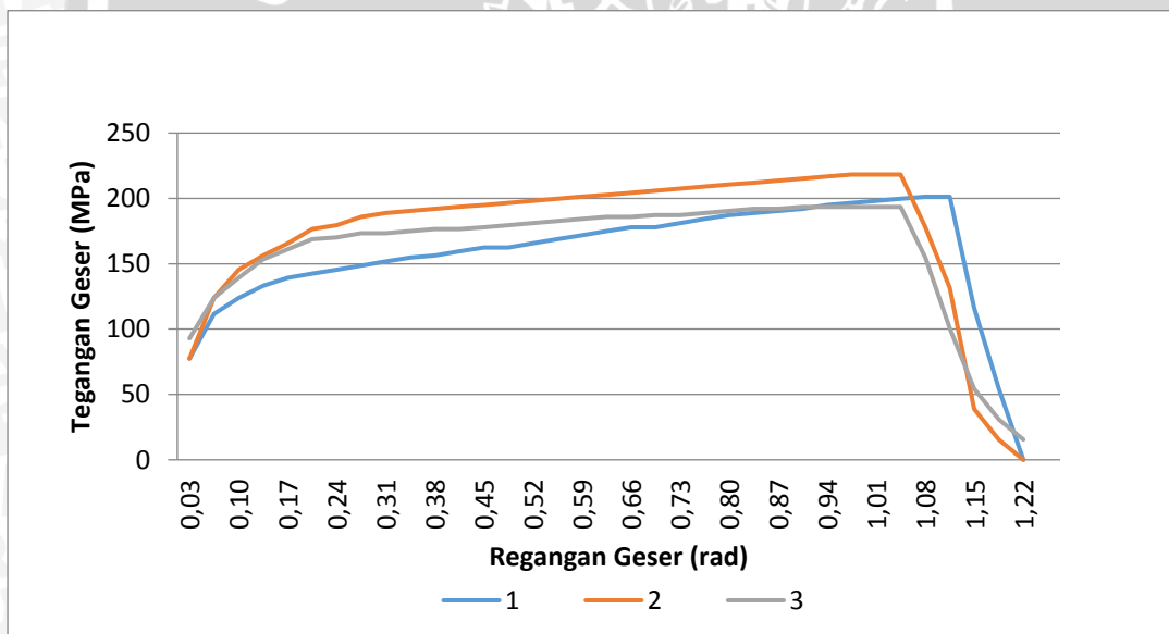
Spesimen sudut chamfer 45° BOL 15 mm
