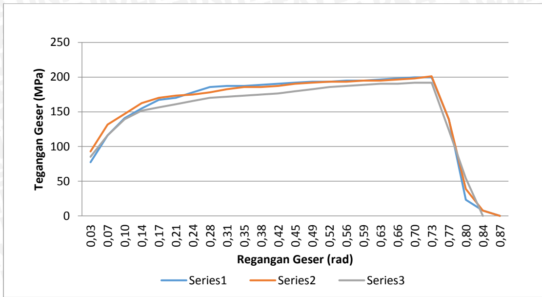
Spesimen sudut chamfer 45° BOL 10 mm
