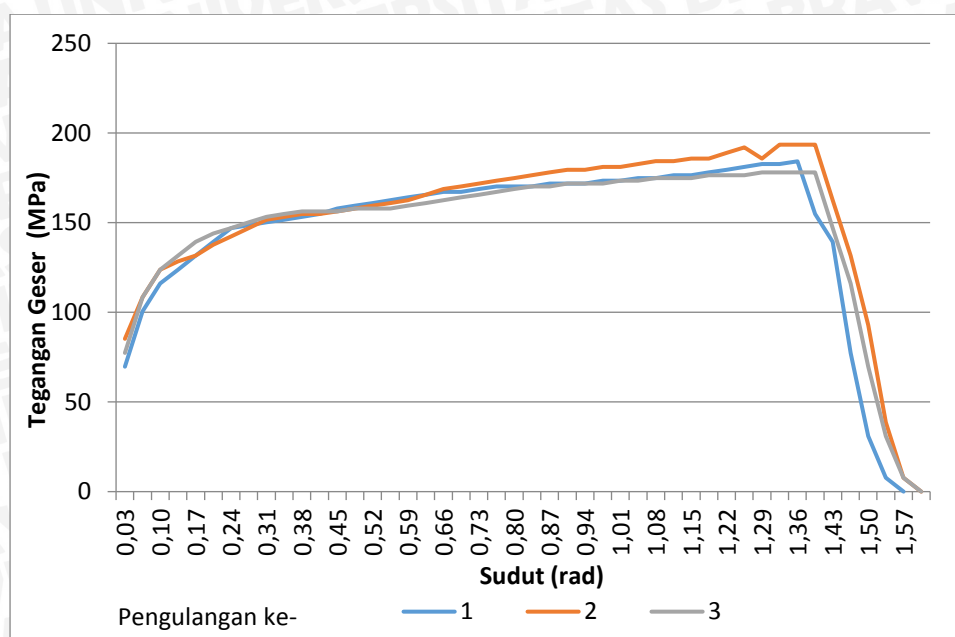
Spesimen sudut chamfer 60° BOL 15 mm
