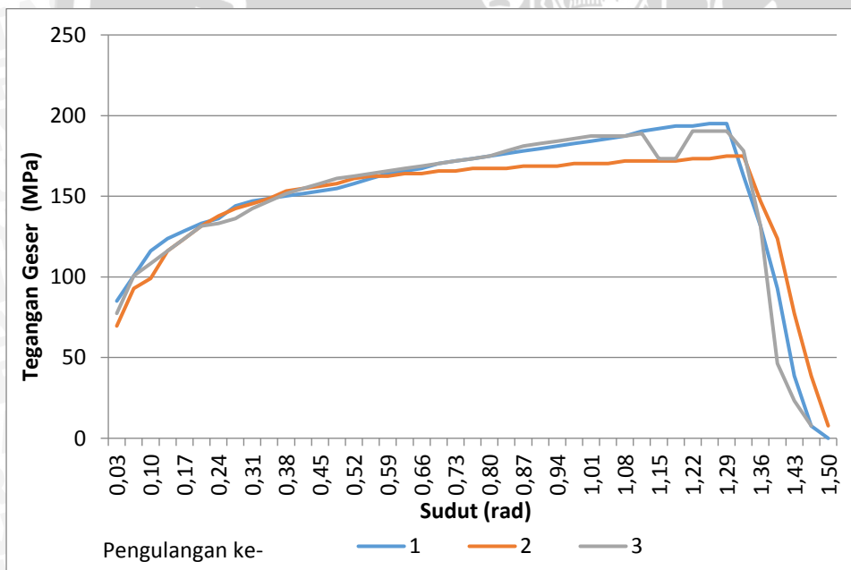
Spesimen sudut chamfer 60° BOL 10 mm
