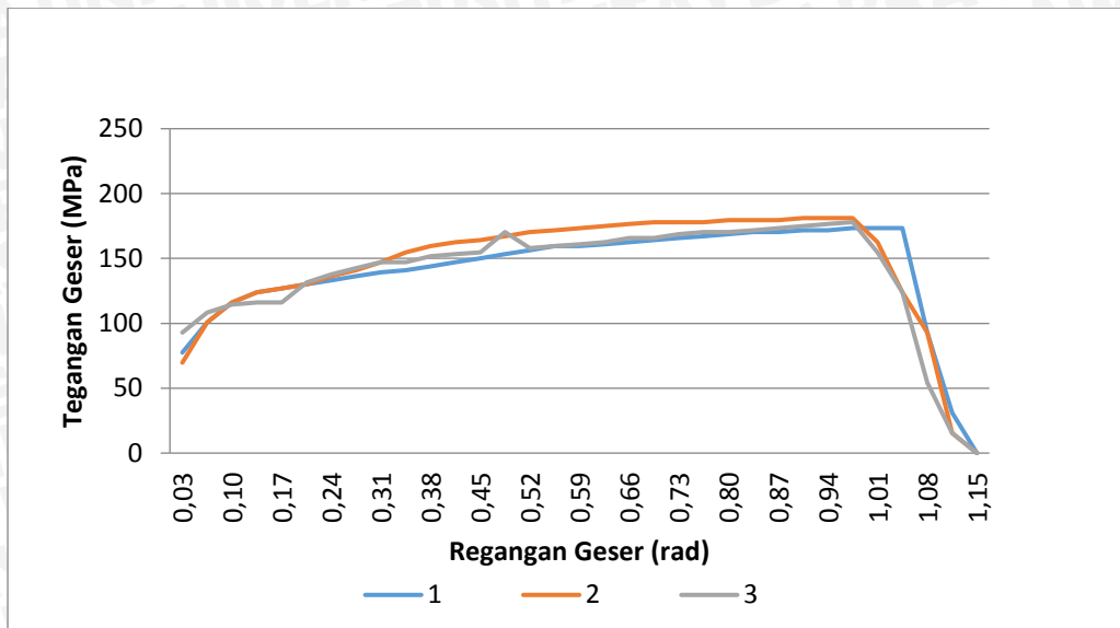
Spesimen sudut chamfer 45° BOL 20 mm
