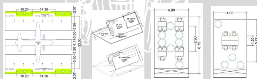
Gambar 9. Ruang-ruang utama hasil sintesa
