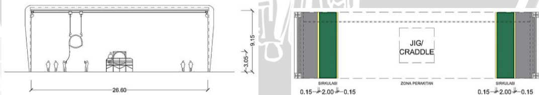
Gambar 1. Kondisi hanggar minimum
