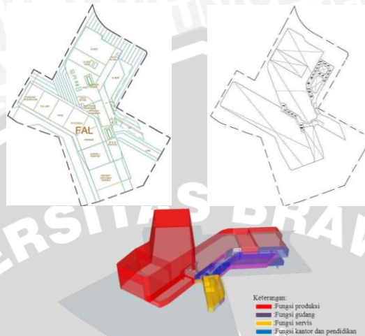
Gambar 8. Konsep tata ruang awal secara horizontal dan perspektif massa
