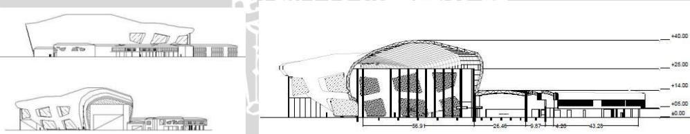
Gambar 13. Hasil Tampak (kanan) dan potongan bangunan (kiri)
