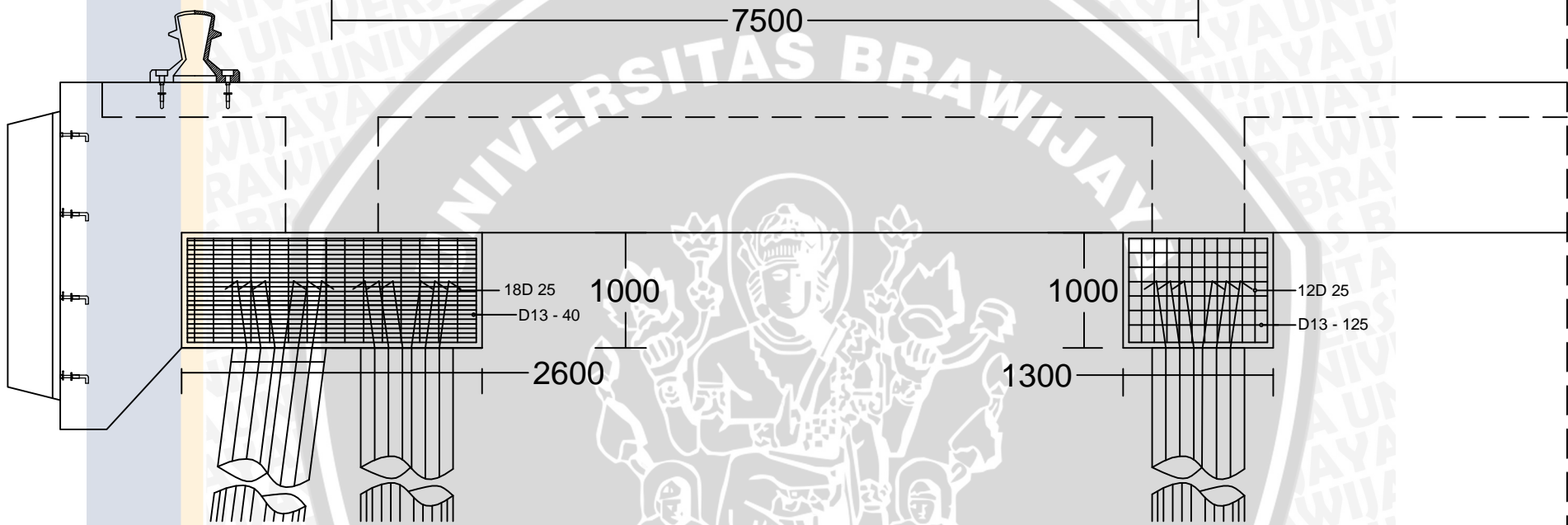
DETAIL PENULANGAN KEPALA TIANG SKALA 1 : 192
