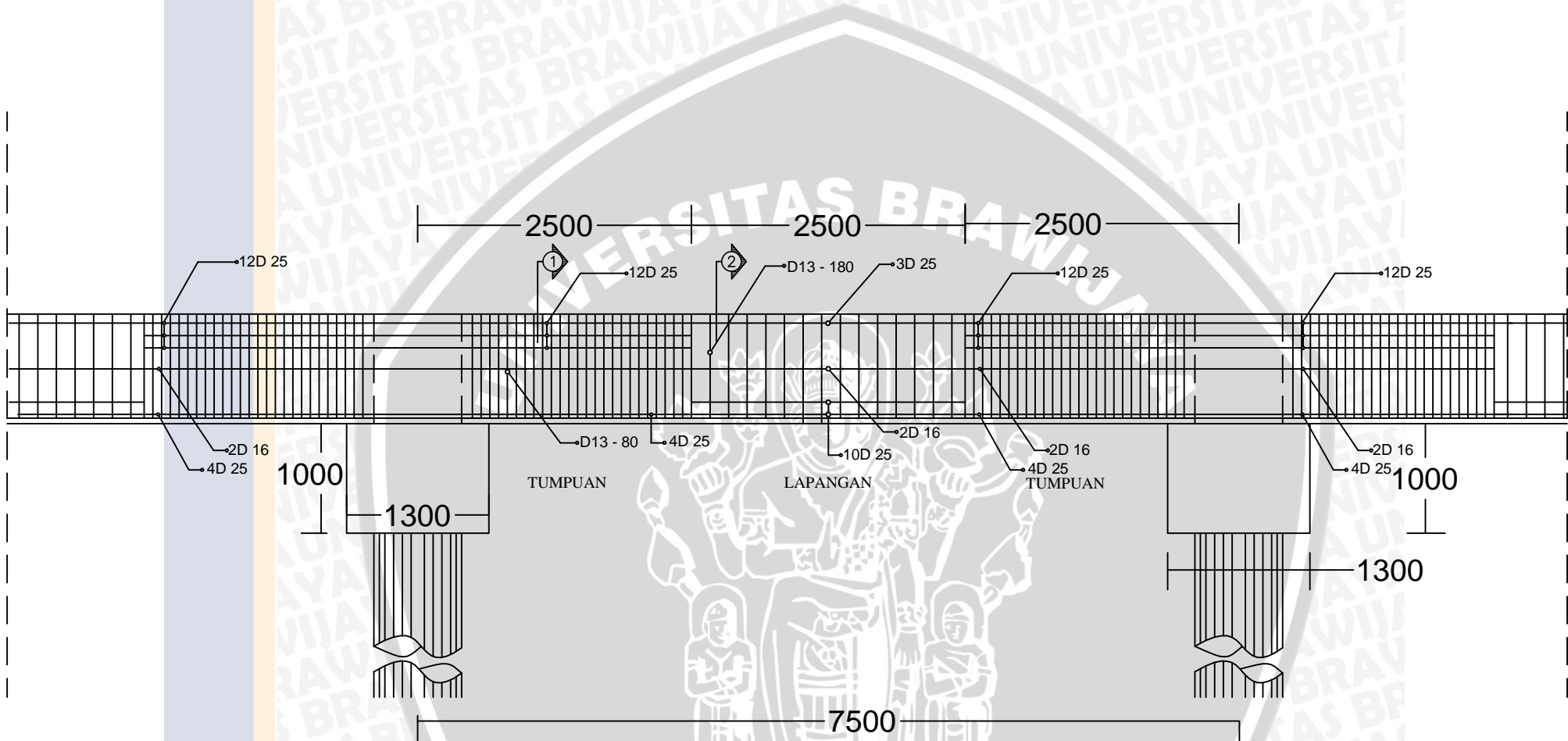
DETAIL PENULANGAN BALOK MELINTANG DERMAGA SKALA 1 : 192
