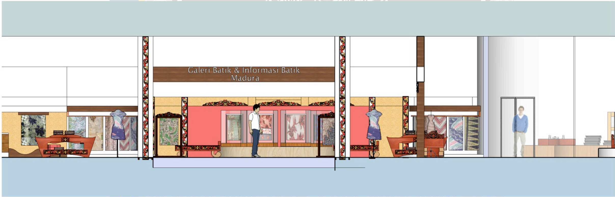
Gambar 4.55 Potongan B-B' Skala 1:50
