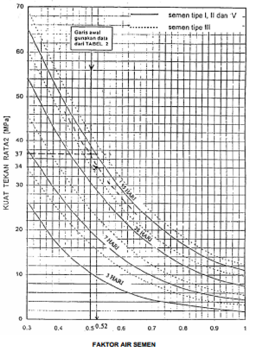
Grafik 1. Hubungan tekanan dan faktor air semen (benda uji berbentuk silinder diameter 150 mm, tinggi 300 mm)
