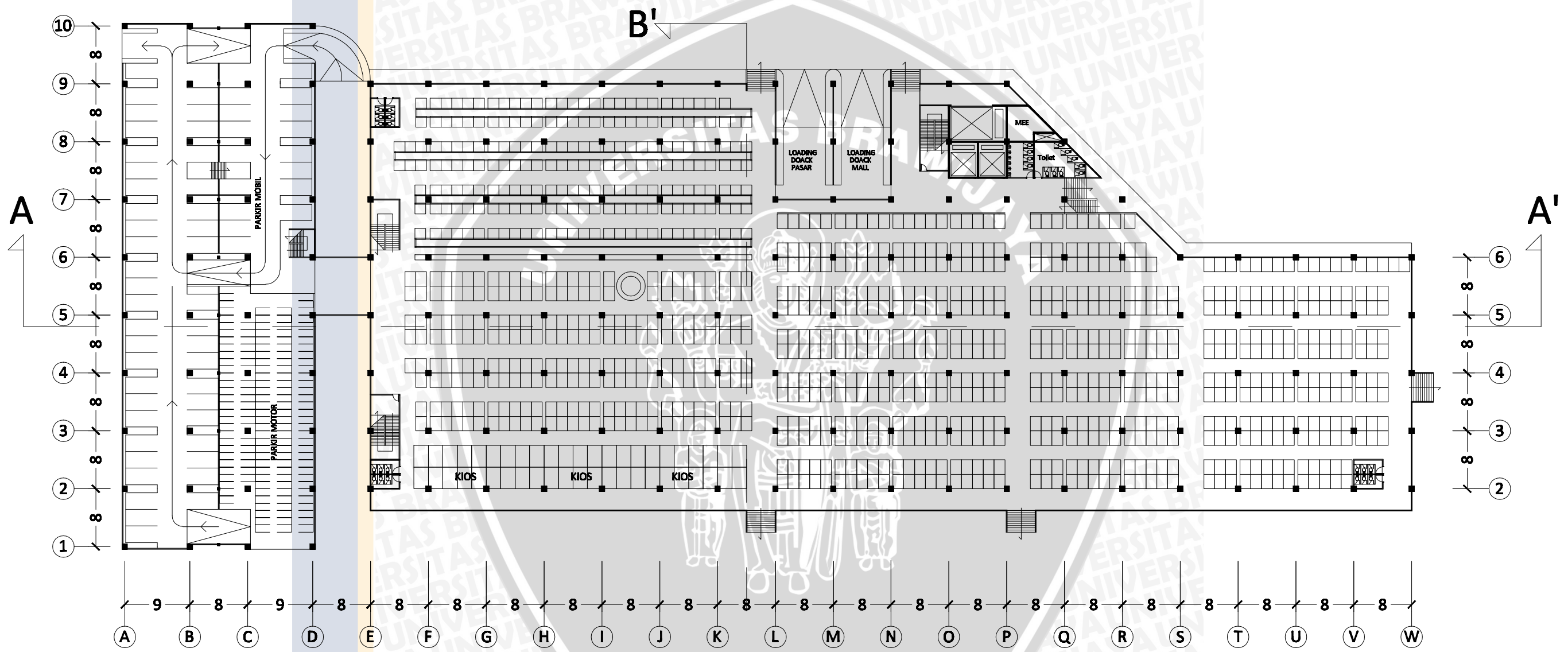
DENAH LANTAI 1 SKALA: 1:600
