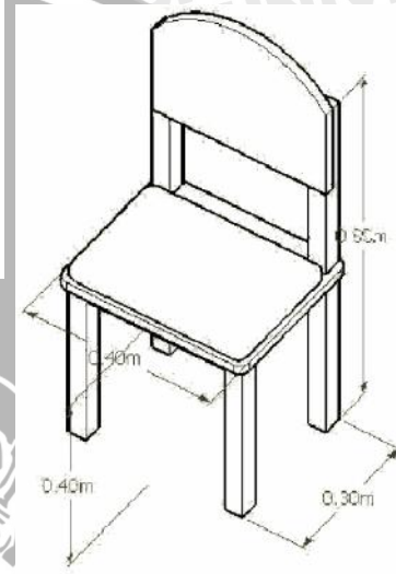
Gambar 4.21 Perspektif Kursi Kelas 1B Sumber : Hasil Desain,2008
