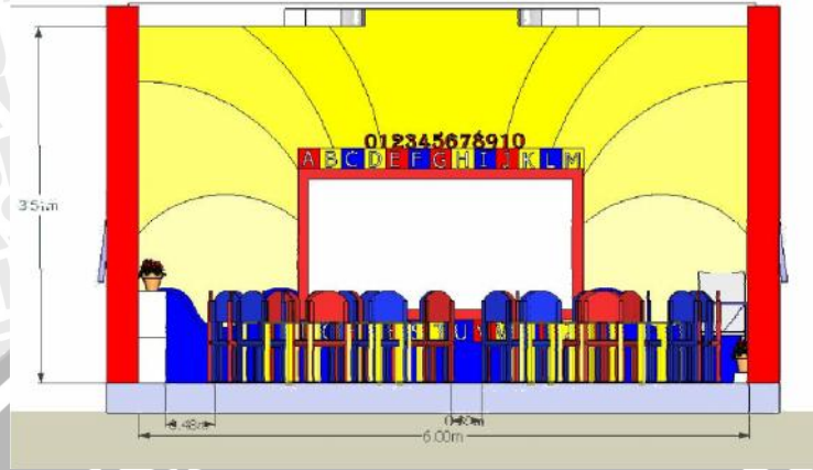
Gambar 4.14 Potongan BB Sumber : Hasil Desain,2008
