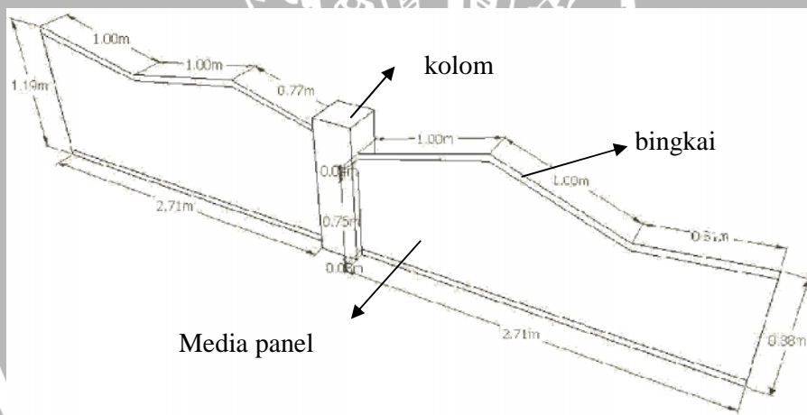
Gambar 4.37 Perspektif Panel Sumber : Hasil Desain,2008
