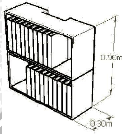
Gambar 4.23 Perspektif Rak Buku Kelas 1B Sumber : Hasil Desain,2008
