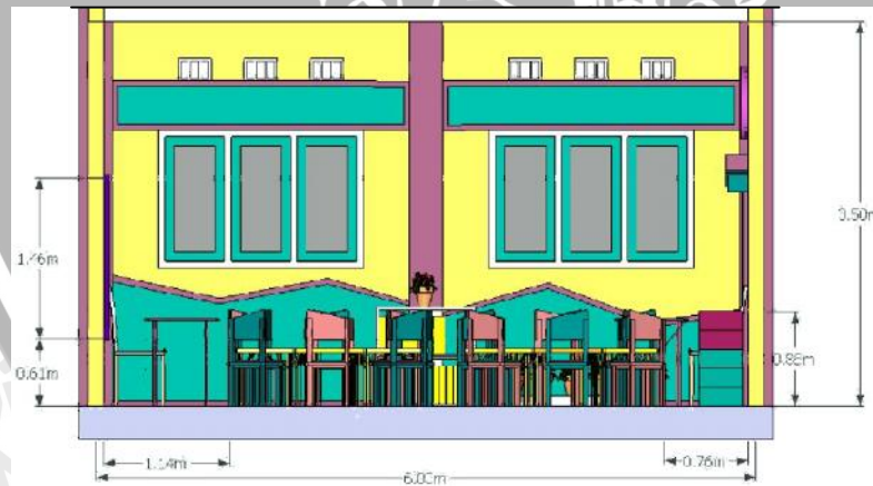
Gambar 4.26 Potongan AA Sumber : Hasil Desain,2008
