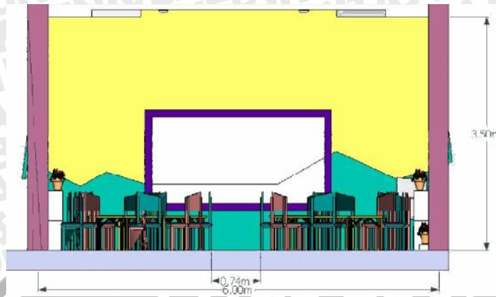
Gambar 4.27 Potongan BB Sumber : Hasil Desain,2008
