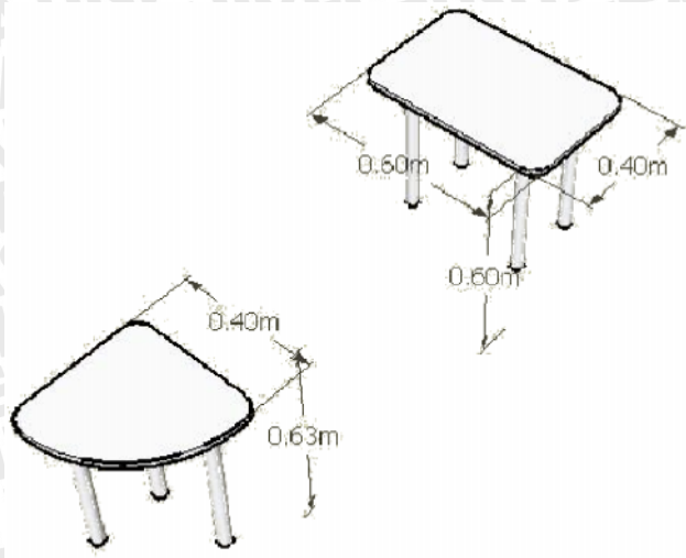
Gambar 4.20 Perspektif Meja Kelas 1B Sumber : Hasil Desain,2008
