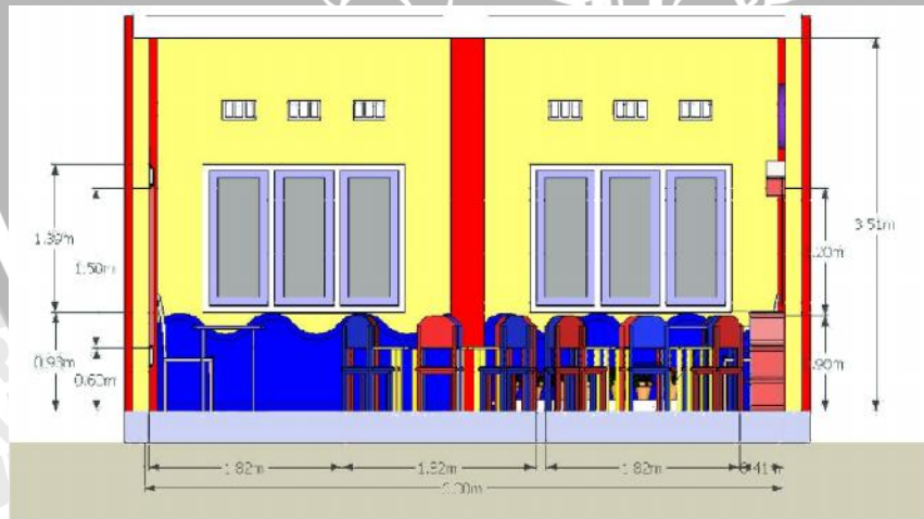
Gambar 4.13 Potongan AA Sumber : Hasil Desain,2008
