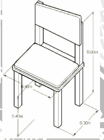
Gambar 4.34 Perspektif Kursi Kelas 3B Sumber : Hasil Desain,2008
