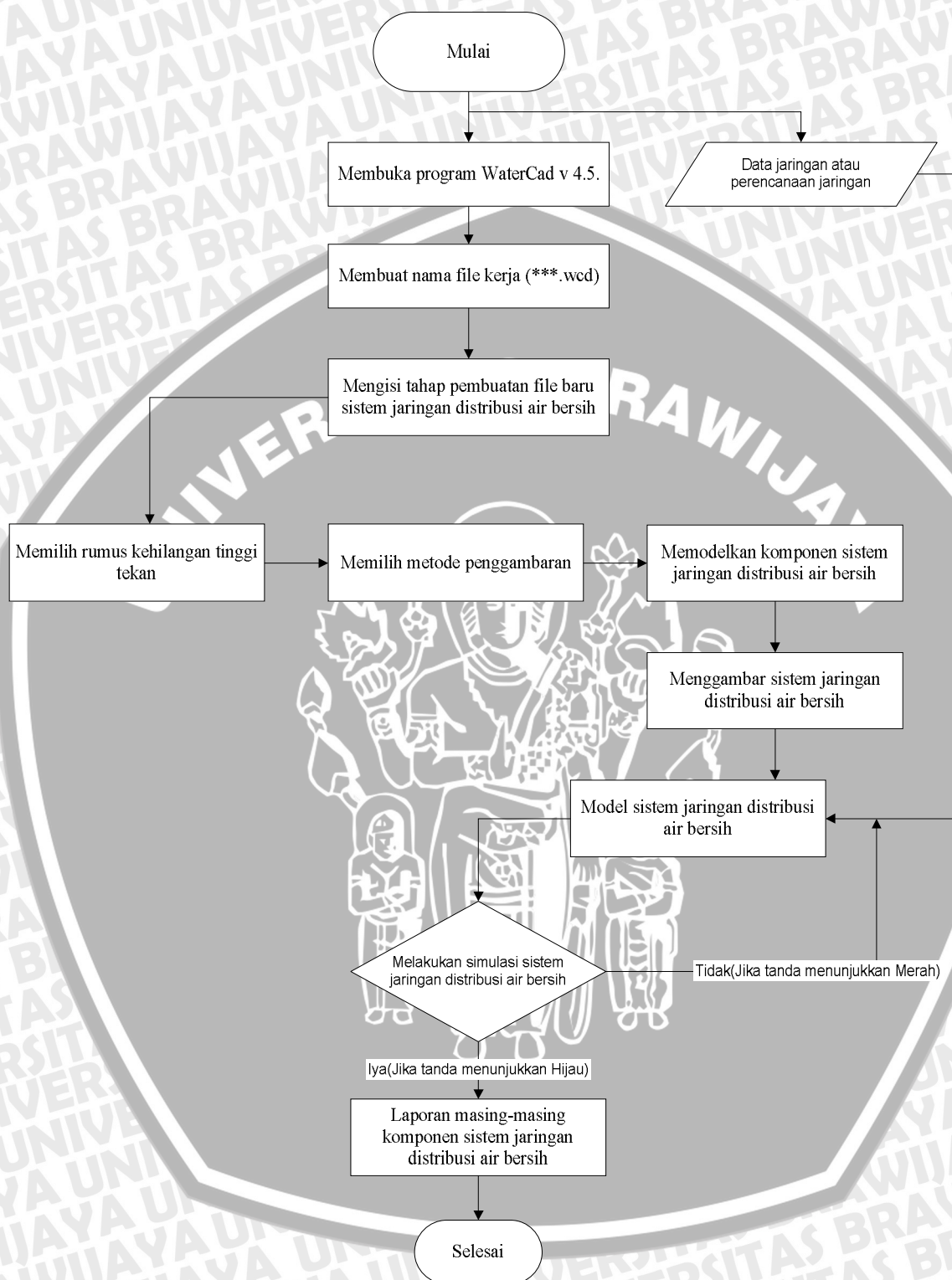
Gambar 3.2. Diagram Alir Proses simulasi sistem jaringan distribusi air bersih dengan menggunakan WaterCad v 4.5.
