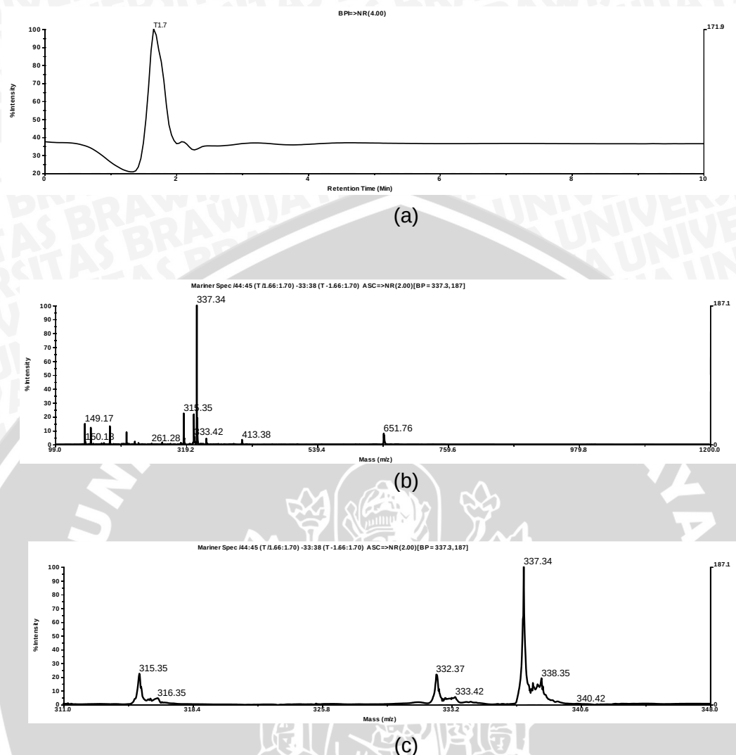
Gambar 10. (a) Spektrum LC (b,c) Spektrum MS, Mikroenkapsul ekstrak kasar teh sargassum cristaefolium pada pH 3. (LIPI Jakarta, 2016)
