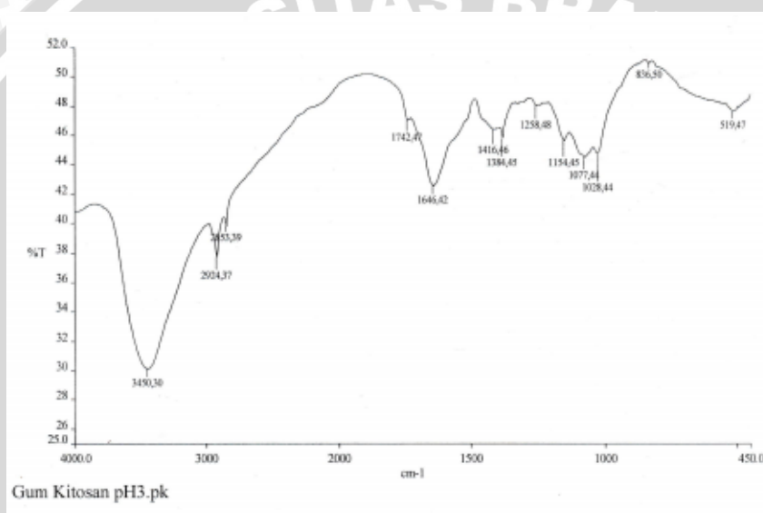
Gambar 9. Hasil Uji FTIR mikroenkapsul ekstrak kasar teh S. cristaefolium (Labolatorium Farmasi Unair, 2016)
