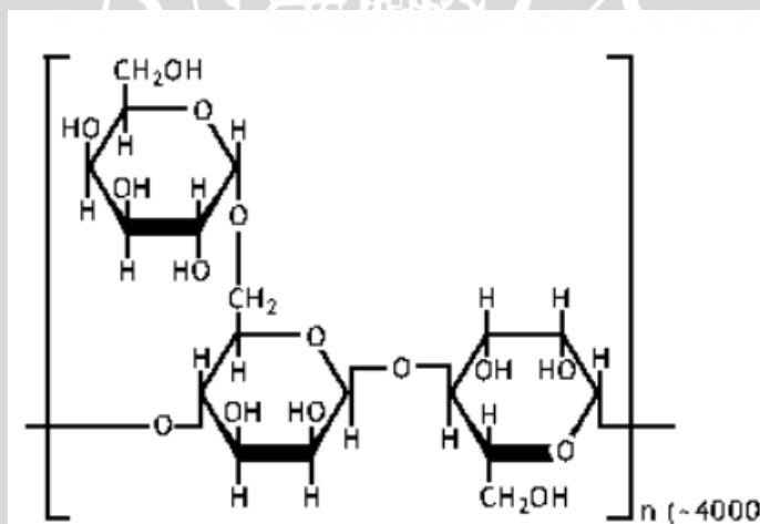
Gambar 5. Struktur Primer Gum Arab (Rini et al., 2012)
