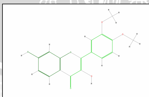
Gambar 11. Senyawa 3,7-Dihidroksi-3',4'-dimetoksiflavin (massbank, 2016)
