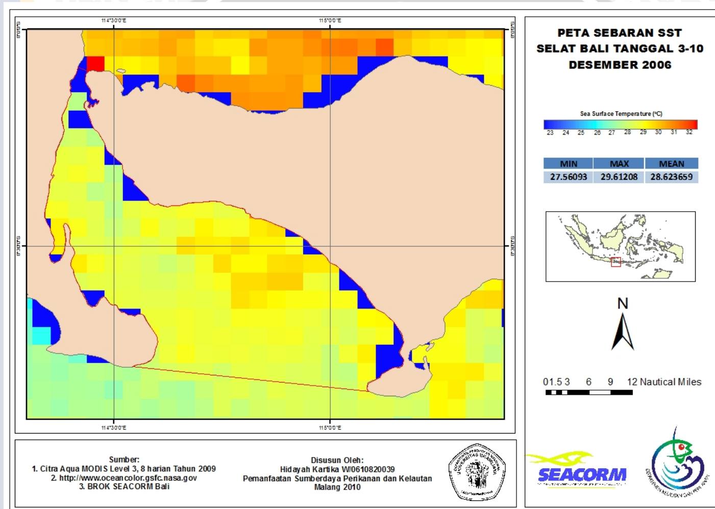
Lampiran 18. Peta Sebaran Suhu Permukaan Laut Tanggal 3-10 Desember Tahun 2006
