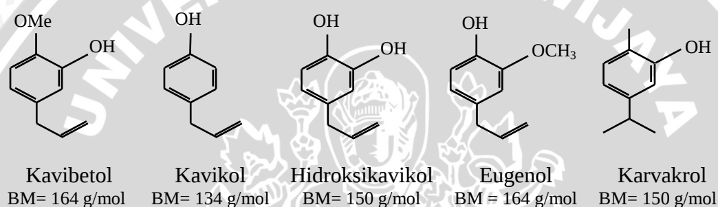
Gambar 5. Struktur senyawa kimia yang terkandung dalam daun sirih
