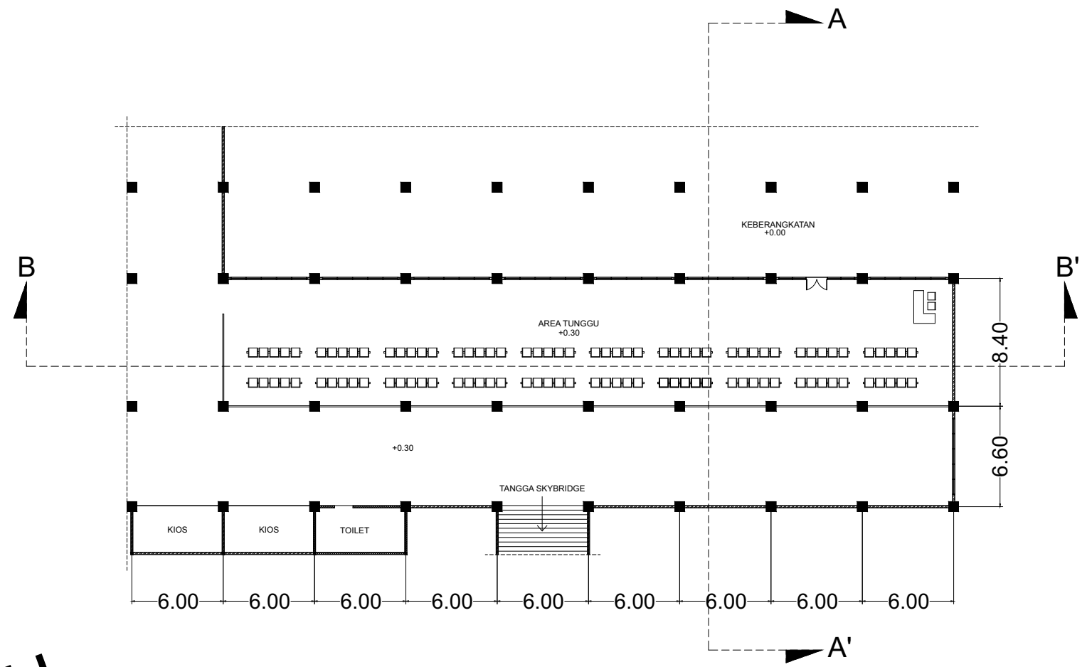
DENAH EKSISTING RUANG TUNGGU TIMUR SKALA 1:500
