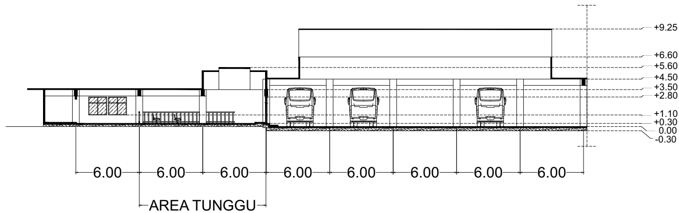
POTONGAN B-B' RUANG TUNGGU BARAT (EKSISTING) SKALA 1:500
