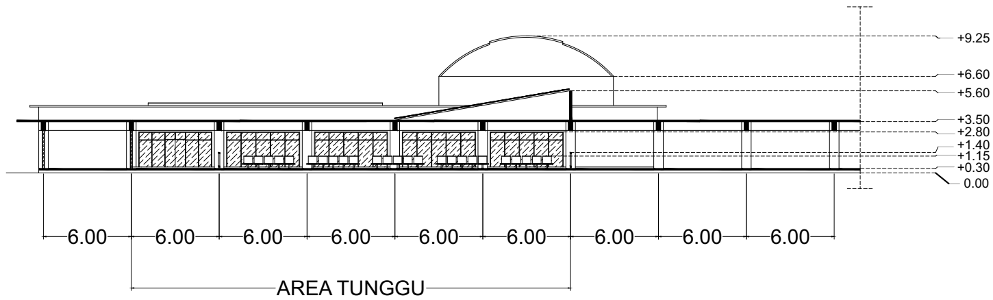
POTONGAN A-A' RUANG TUNGGU BARAT (HASIL AKHIR) SKALA 1:500
