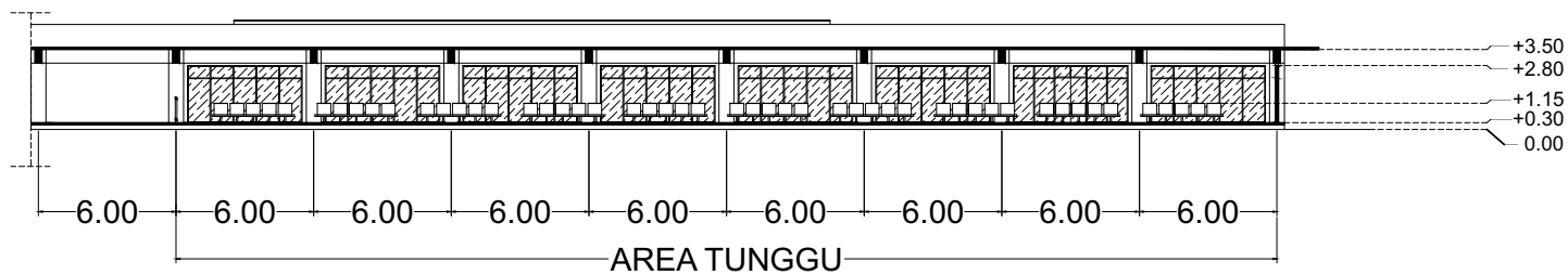
POTONGAN B-B' RUANG TUNGGU TIMUR (HASIL AKHIR) SKALA 1:500
