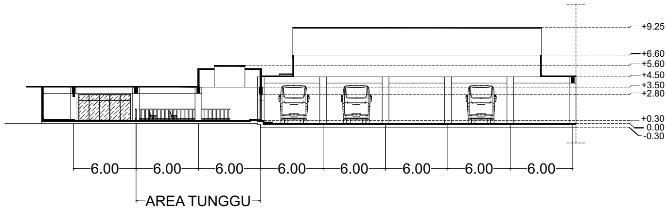
POTONGAN B-B' RUANG TUNGGU BARAT (HASIL AKHIR) SKALA 1:500
