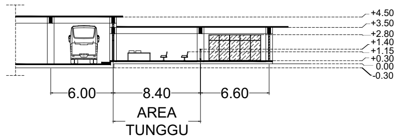
POTONGAN A-A' RUANG TUNGGU TIMUR (EKSISTING) SKALA 1:500
