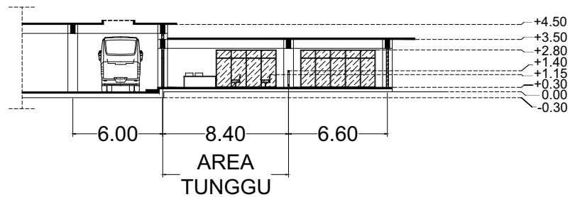
POTONGAN A-A' RUANG TUNGGU TIMUR (HASIL AKHIR) SKALA 1:500
