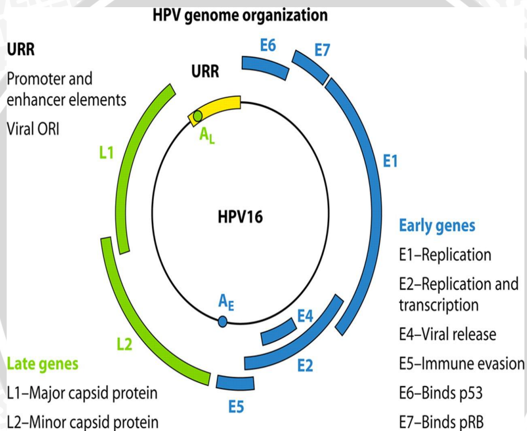
Gambar 2.4 Skema genom HPV beserta fungsinya (Lukman , 2010)
