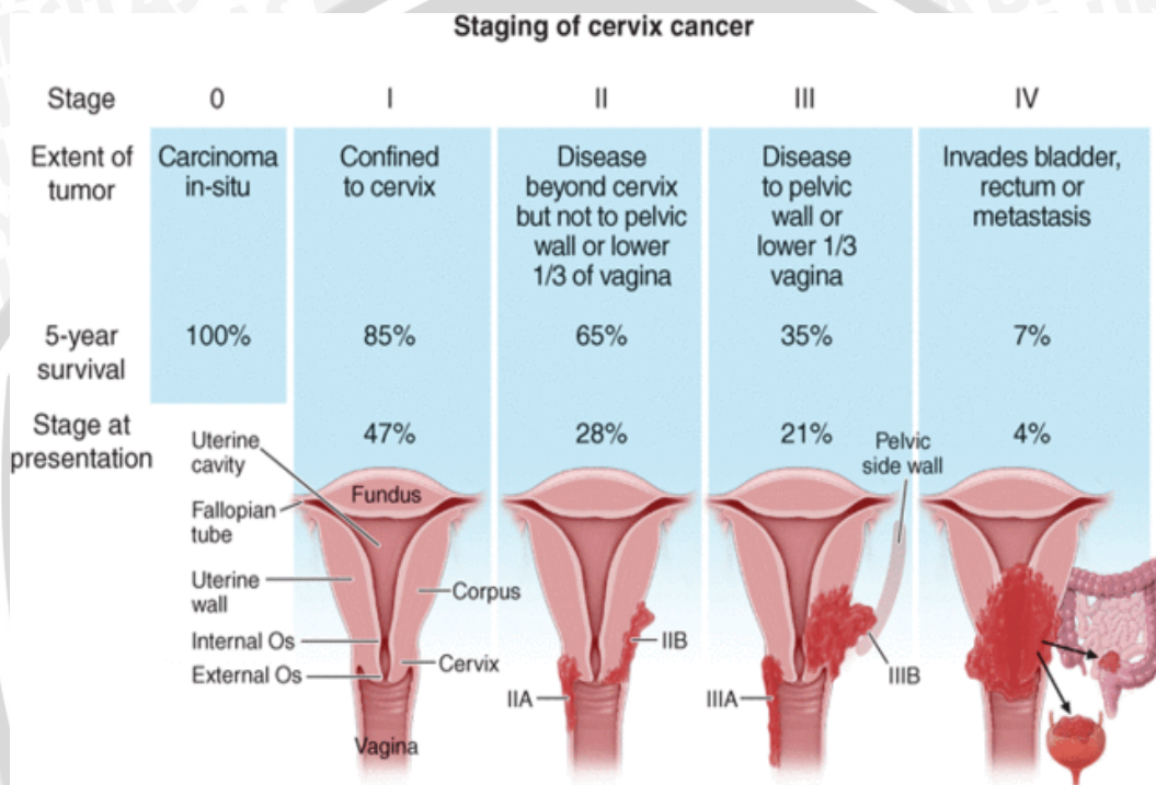
Gambar 2.6 Stadium Kanker Serviks Menurut FIGO dan AJCC (ACS,2014)
