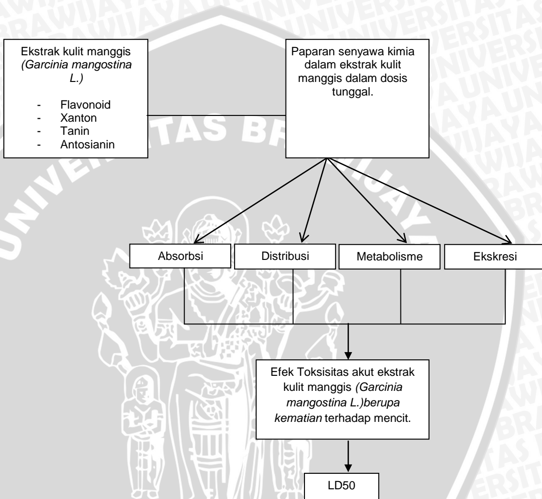
Gambar 3.1. Kerangka Konsep
