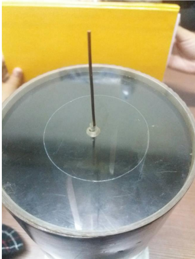
Gambar 4. Objek uji berupa susunan elektroda koaksial
