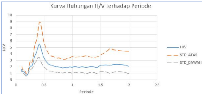
Gambar Lampiran 4.11 Kurva hubungan A_0 dan T_0 di titik KA11.
