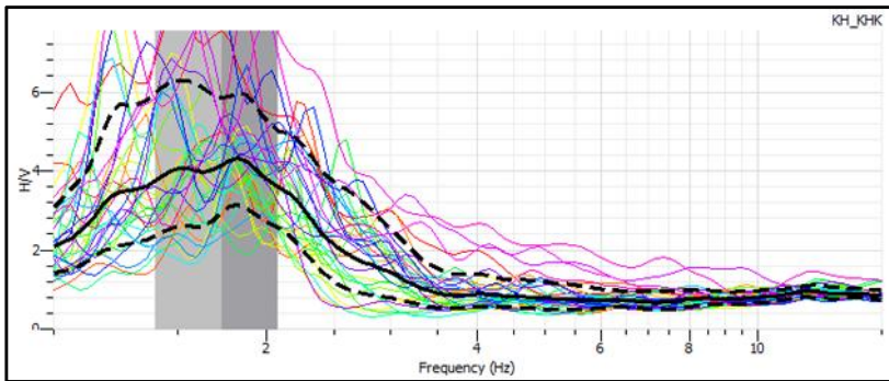
Gambar Lampiran 3.17 Kurva HVSR di titik KA17.
