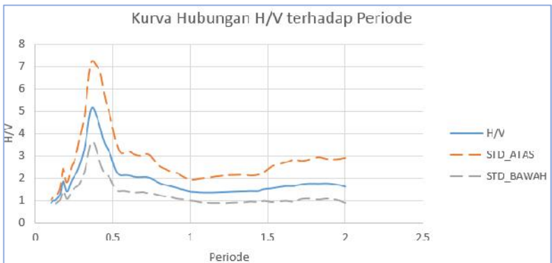
Gambar Lampiran 4.9 Kurva hubungan A_0 dan T_0 di titik KA9.
