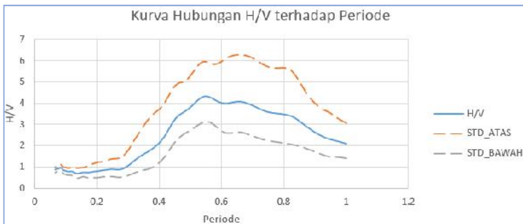
Gambar Lampiran 4.17 Kurva hubungan A_0 dan T_0 di titik KA17.
