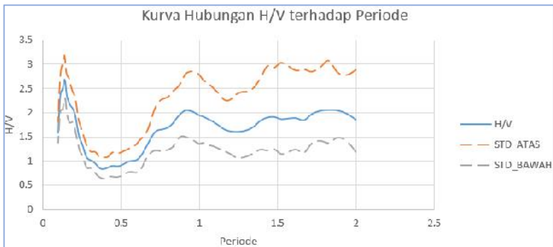
Gambar Lampiran 4.16 Kurva hubungan A_0 dan T_0 di titik KA16.
