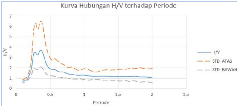
Gambar Lampiran 4.10 Kurva hubungan A_0 dan T_0 di titik KA10.
