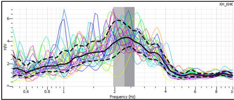
Gambar Lampiran 3.23 Kurva HVSR di titik KA23.
