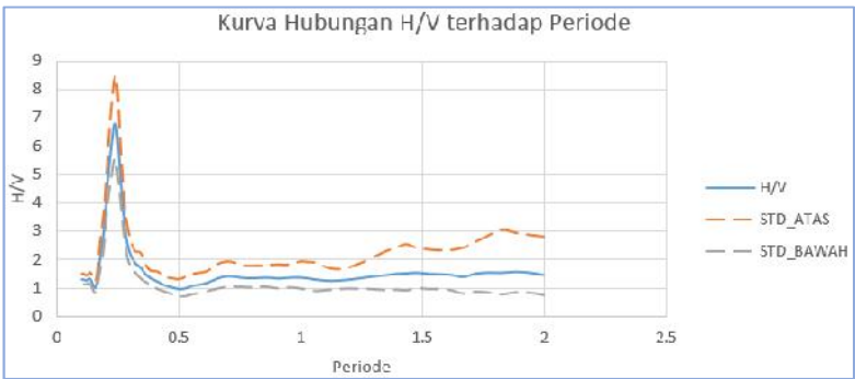
Gambar Lampiran 4.24 Kurva hubungan A_0 dan T_0 di titik KA24.
