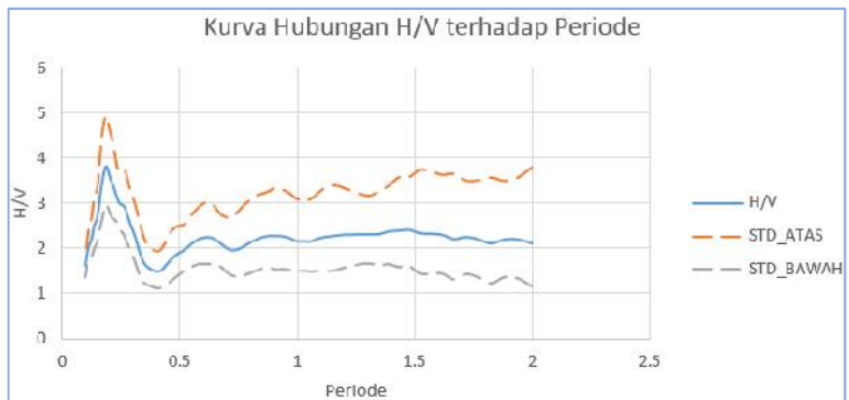
Gambar Lampiran 4.20 Kurva hubungan A_0 dan T_0 di titik KA20.
