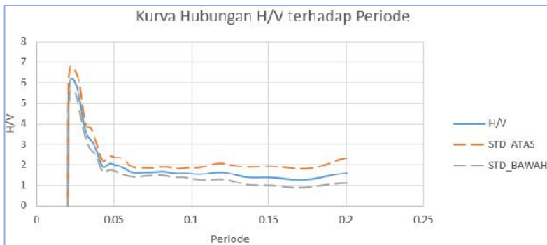
Gambar Lampiran 4.5 Kurva hubungan A_0 dan T_0 di titik KA5.
