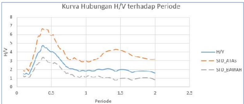
Gambar Lampiran 4.8 Kurva hubungan A_0 dan T_0 di titik KA8.
