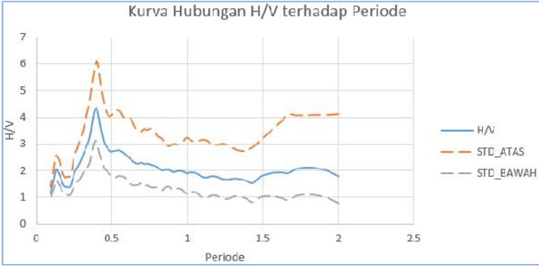
Gambar Lampiran 4.22 Kurva hubungan A_0 dan T_0 di titik KA22.
