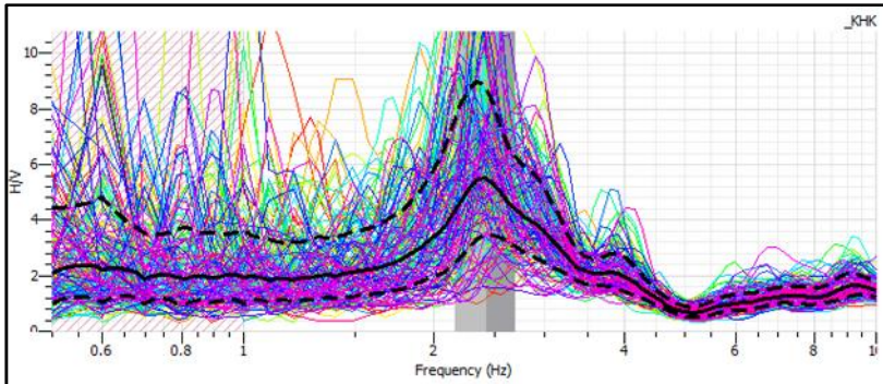
Gambar Lampiran 3.11 Kurva HVSR di titik KA11.
