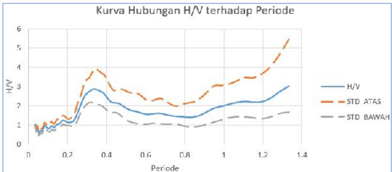
Gambar Lampiran 4.15 Kurva hubungan A_0 dan T_0 di titik KA15.
