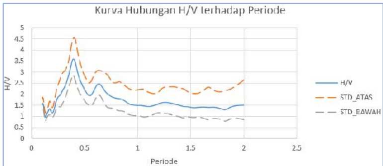
Gambar Lampiran 4.14 Kurva hubungan A_0 dan T_0 di titik KA14.
