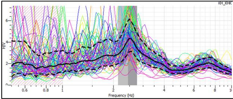
Gambar Lampiran 3.22 Kurva HVSR di titik KA22.
