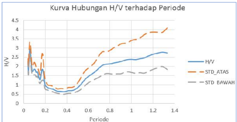
Gambar Lampiran 4.21 Kurva hubungan A_0 dan T_0 di titik KA21.
