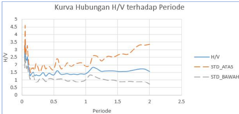
Gambar Lampiran 4.4 Kurva hubungan A_0 dan T_0 di titik KA4.
