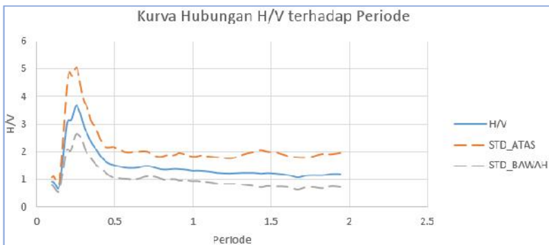
Gambar Lampiran 4.12 Kurva hubungan A_0 dan T_0 di titik KA12.
