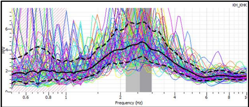
Gambar Lampiran 3.8 Kurva HVSR di titik KA8.
