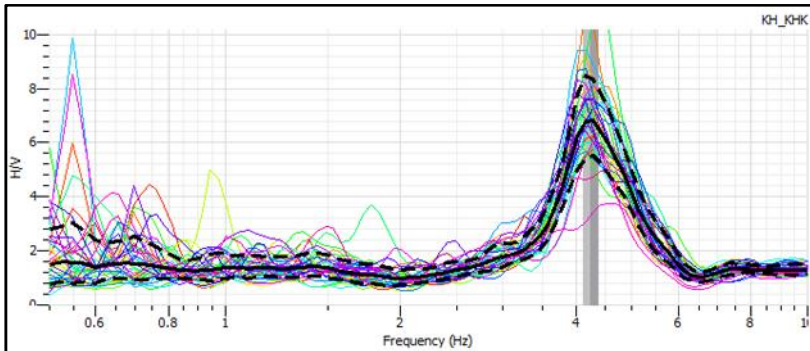
Gambar Lampiran 3.24 Kurva HVSR di titik KA24.
