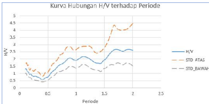
Gambar Lampiran 4.3 Kurva hubungan A_0 dan T_0 di titik KA3.
