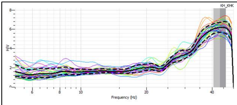
Gambar Lampiran 3.5 Kurva HVSR di titik KA5.
