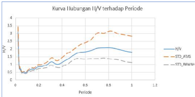
Gambar Lampiran 4.1 Kurva hubungan A_0 dan T_0 di titik KA1.
