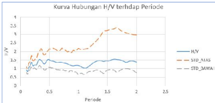
Gambar Lampiran 4.2 Kurva hubungan A_0 dan T_0 di titik KA2.
