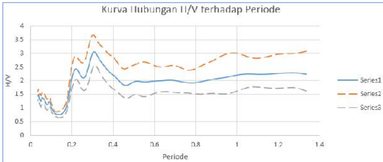
Gambar Lampiran 4.19 Kurva hubungan A_0 dan T_0 di titik KA19.
