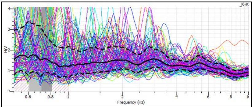
Gambar Lampiran 3.2 Kurva HVSR di titik KA2.
