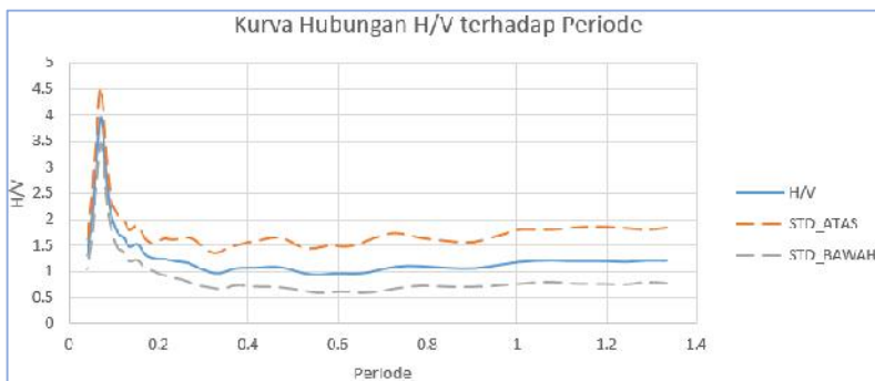
Gambar Lampiran 4.6 Kurva hubungan A_0 dan T_0 di titik KA6.
