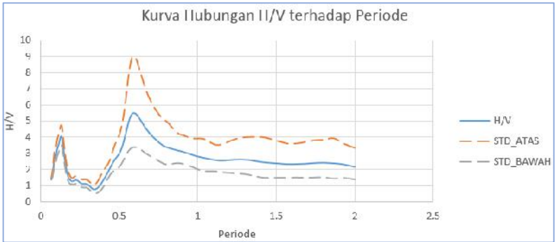
Gambar Lampiran 4.13 Kurva hubungan A_0 dan T_0 di titik KA13.
