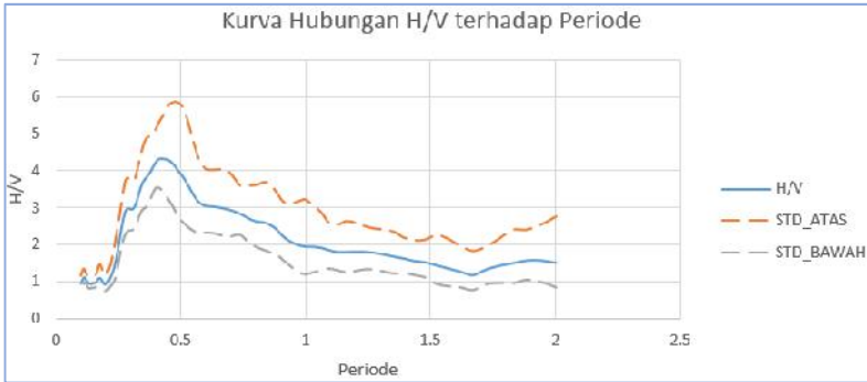
Gambar Lampiran 4.23 Kurva hubungan A_0 dan T_0 di titik KA23.
