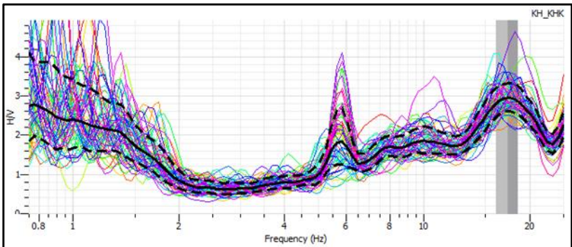
Gambar Lampiran 3.21 Kurva HVSr di titik KA21.
