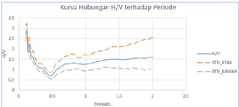
Gambar Lampiran 4.7 Kurva hubungan A_0 dan T_0 di titik KA7.
