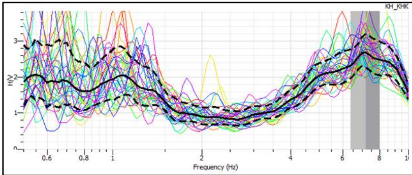
Gambar Lampiran 3.16 Kurva HVSR di titik KA16.
