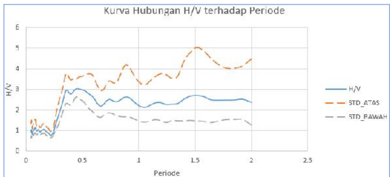
Gambar Lampiran 4.18 Kurva hubungan A_0 dan T_0 di titik KA18.
