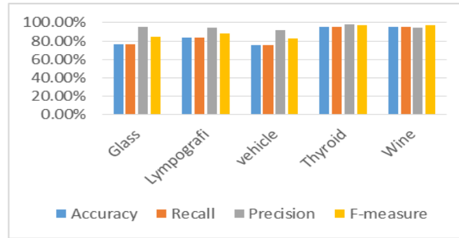
Gambar 5.15 Diagram Hasil Pengujian csDT
