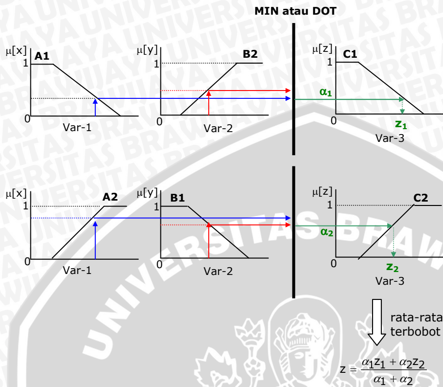
Gambar 7.32 Inferensi dengan menggunakan Metode Tsukamoto.
