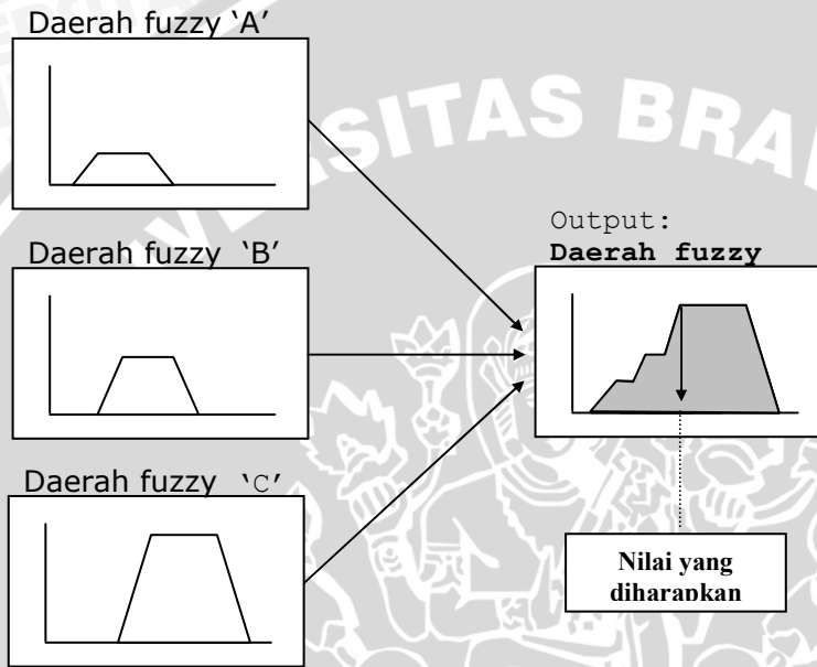
Gambar 7.37 Proses defuzzifikasi.
