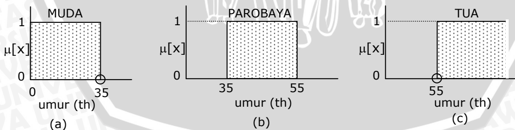
Gambar 7.2 Himpunan: MUDA, PAROBAYA, dan TUA.
