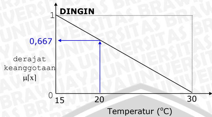
Gambar 7.8 Himpunan fuzzy: DINGIN.
