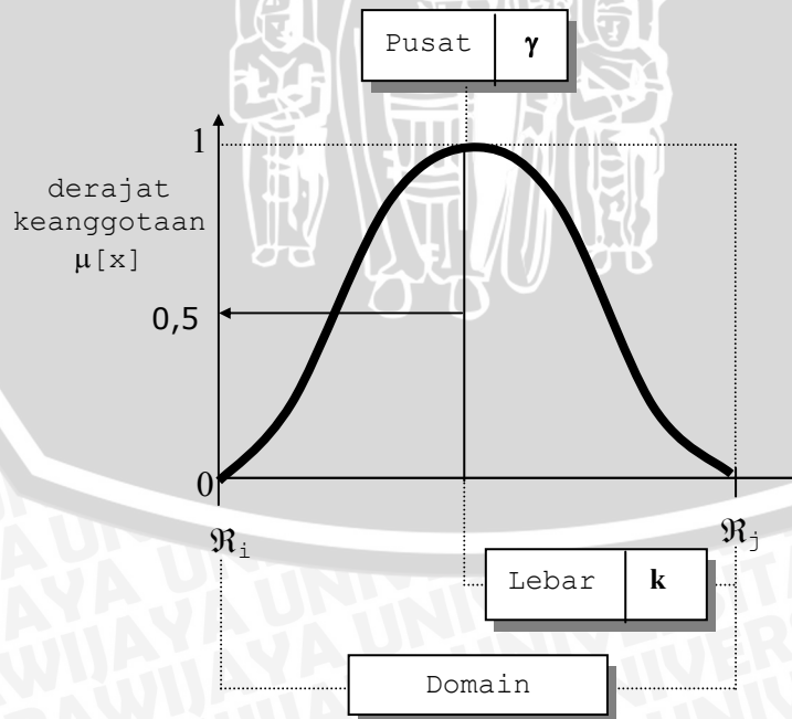
Gambar 7.25 Karakteristik fungsional kurva GAUSS.
