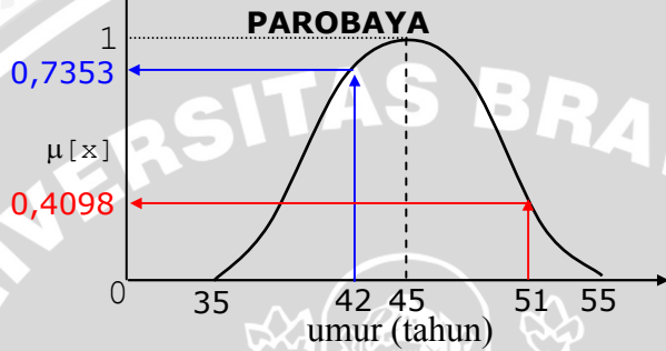
Gambar 7.23 Himpunan Fuzzy: SETENGAH BAYA dengan kurva Beta.
