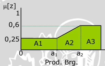
Gambar 7.42 Daerah hasil komposisi.
