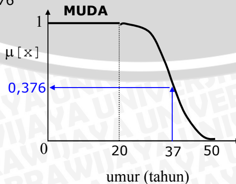
Gambar 7.18 Himpunan Fuzzy: MUDA.
