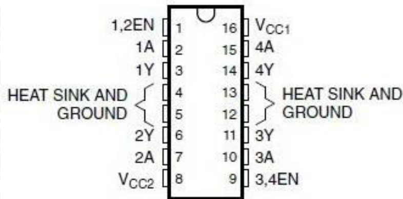
Gambar 2.8 IC L293d
