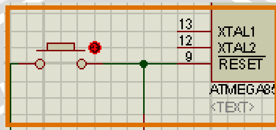
Gambar 4.16 Rangkaian Sistem Reset
