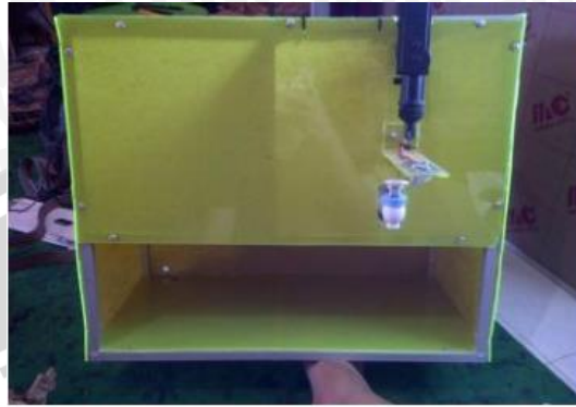
Gambar 2.2 Kran dan Pengering Tangan Otomatis (Fachrul Ramadhan)
