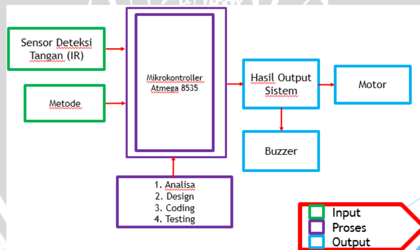
Gambar 4.10 Diagram Blok Sistem
