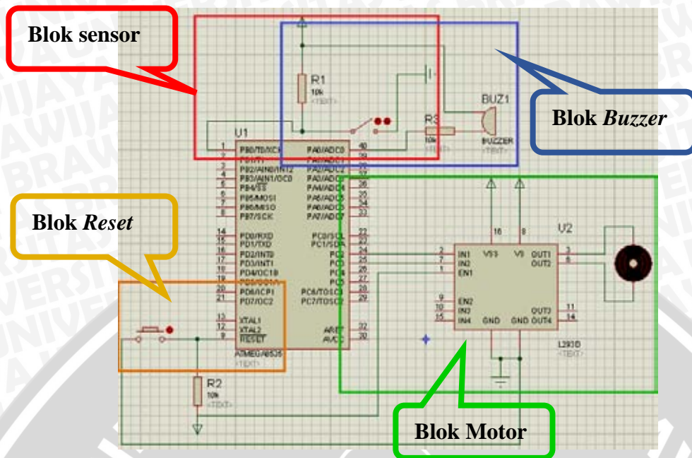
Gambar 4.11 Rangkaian Keseluruhan Kran CTPS
