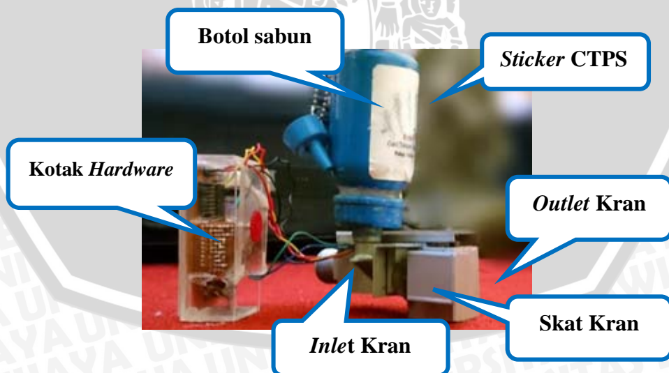
Gambar 5.8 Badan Kran. Tampak: kotak hardware, outlet kran, wadah sabun, sekat
