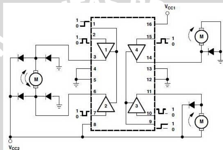
Gambar 2.9 Rangkaian IC L293d
