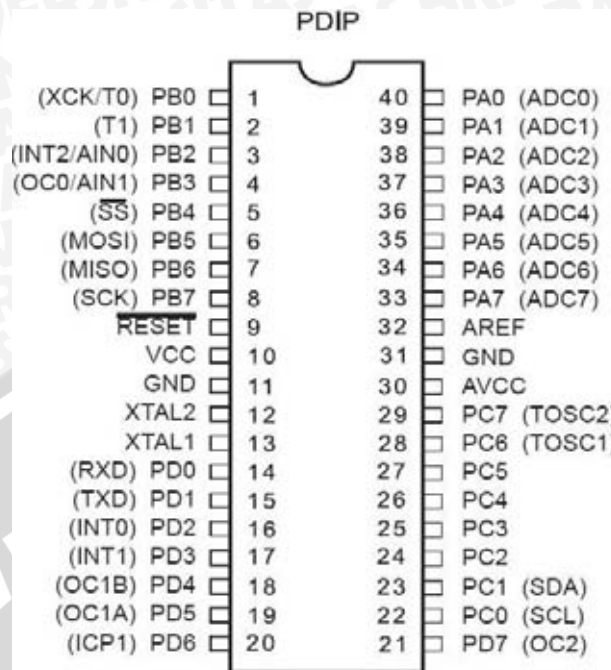
Gambar 2.6 Mikrokontroler ATMEGA 8535
