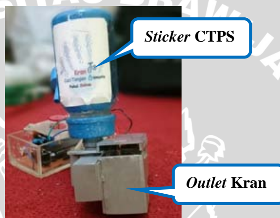
Gambar 5.7 Badan Kran. Tampak: sticker ctps dan outlet kran
