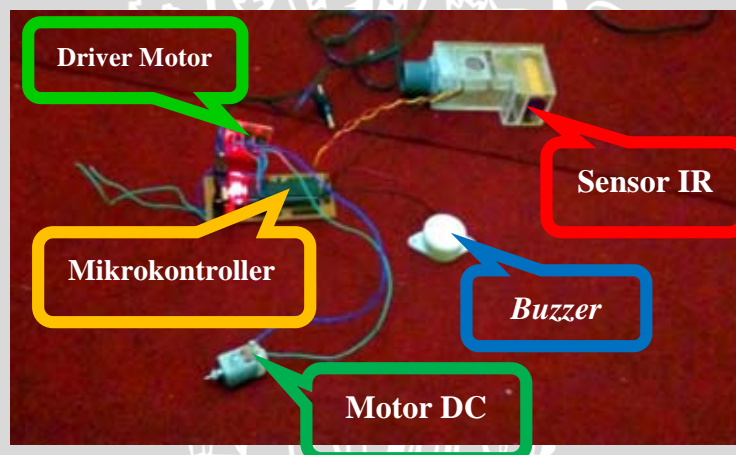
Gambar 5.5 Rangkaian Keseluruhan
