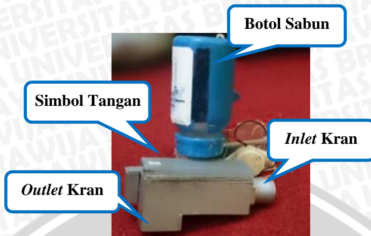
Gambar 5.6 Badan Kran. Tampak: wadah sabun, inlet dan outlet kran
