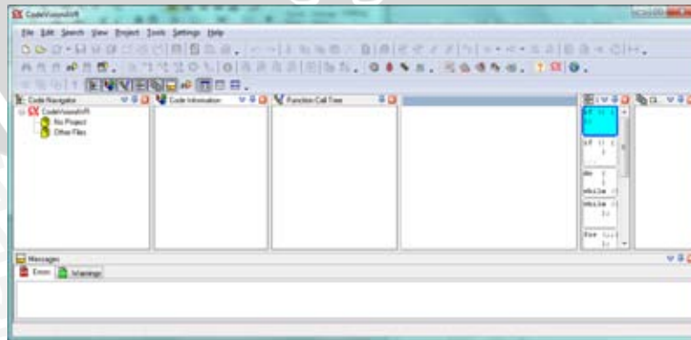
Gambar 2.11 CodeVision AVR
