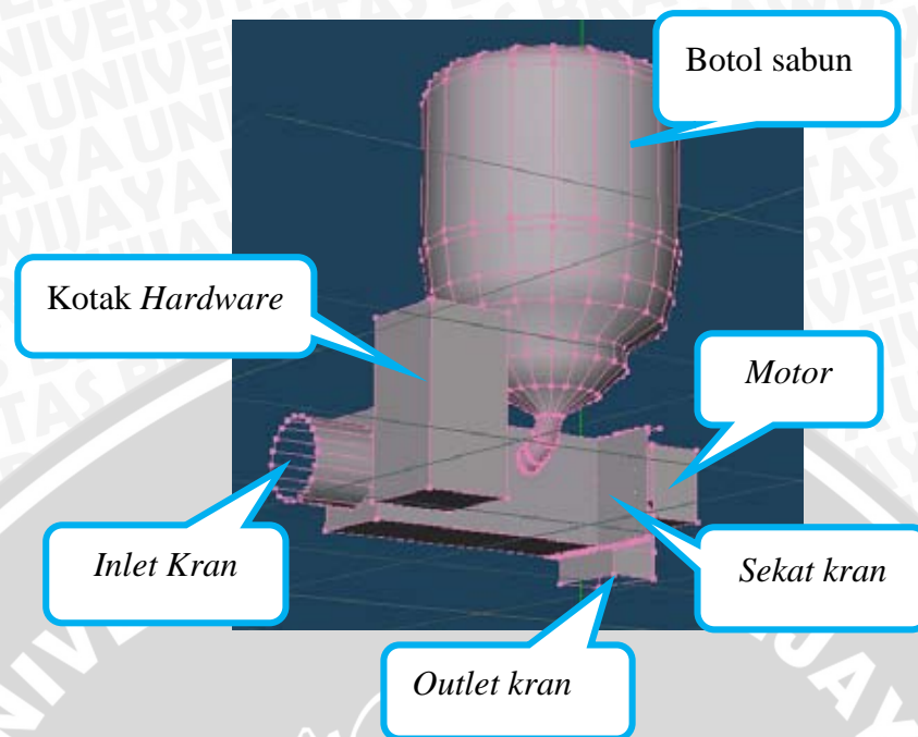
Gambar 4.17 Desain Case Akrilik Kran CTPS
