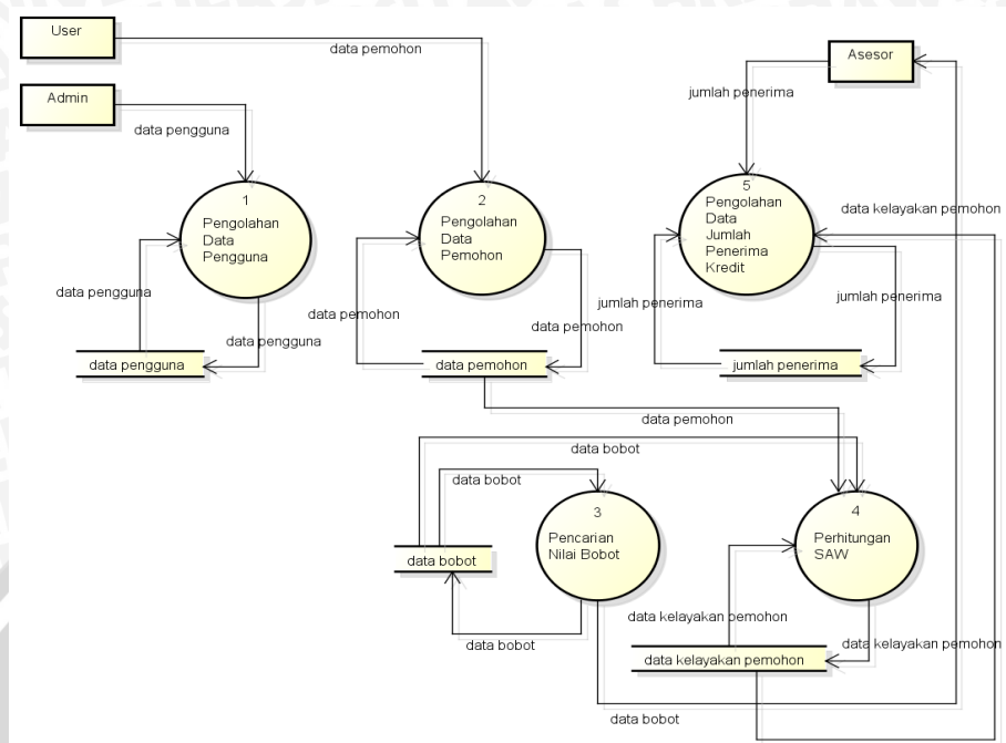
Gambar 3.8 DFD Level 1 untuk Pengolahan Data
