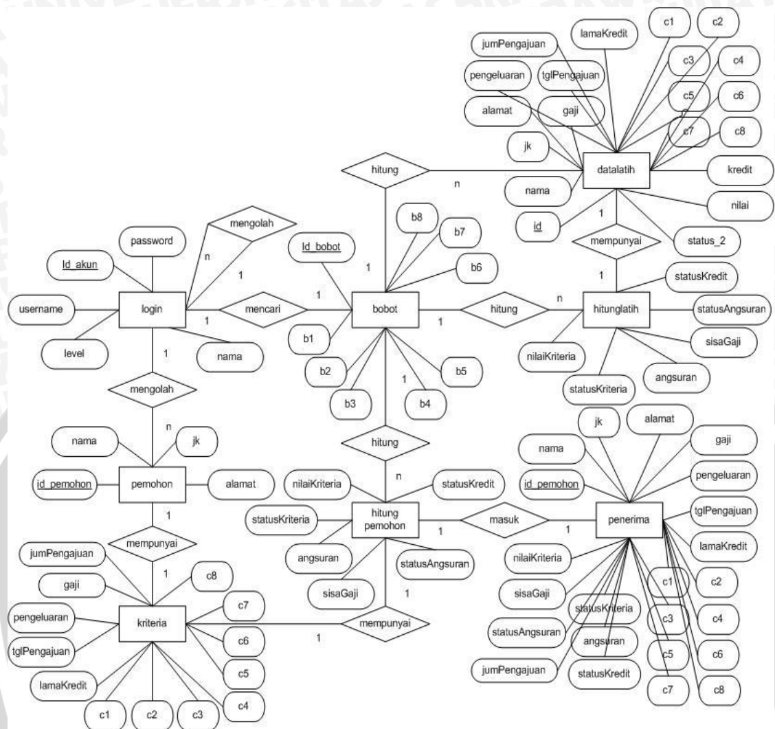
Gambar 3.4 Entity Relationship Diagram SPK Kelayakan Pemohon Kredit Motor
