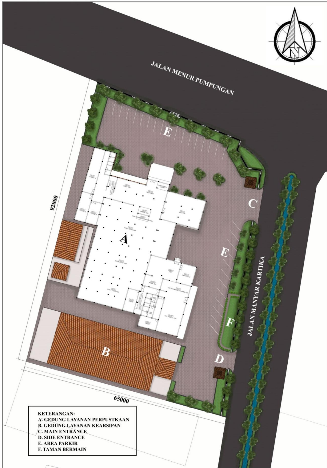
Lampiran 2 Layout Plan Badan Perpustakaan dan Kearsipan Provinsi Jawa Timur (Eksisting)
