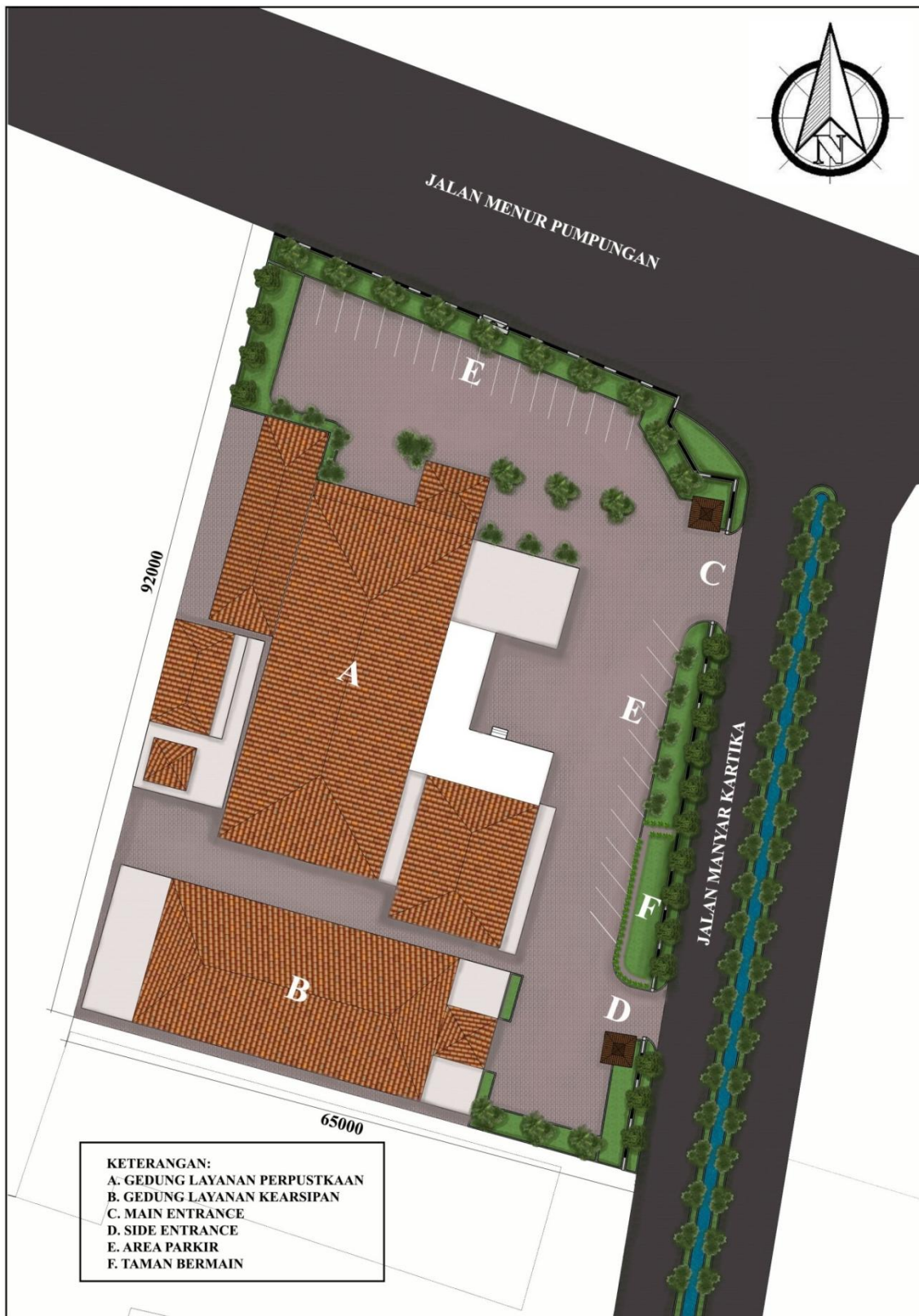
Lampiran 1 Site Plan Badan Perpustakaan dan Kearsipan Provinsi Jawa Timur (Eksisting)
