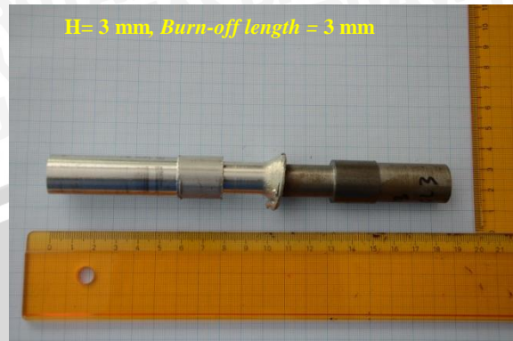
Foto Spesimen Uji Tarik
