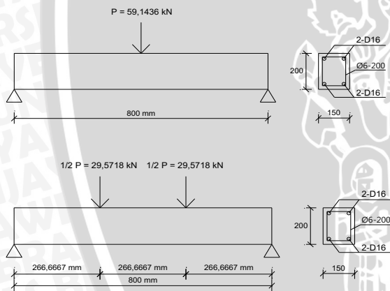
Gambar 2. Benda Uji
