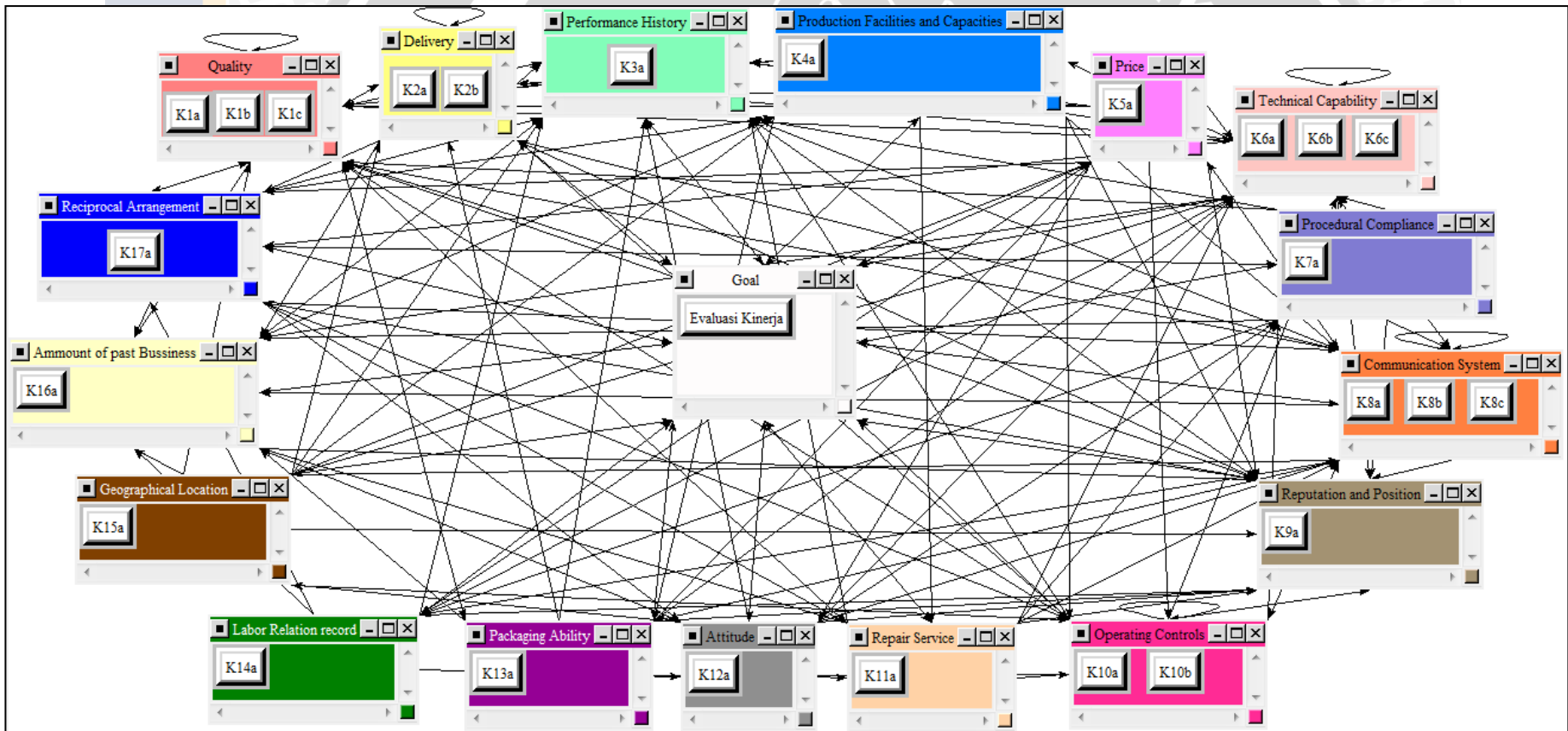
Gambar 4.5 Model jaringan ANP pengukuran kinerja supplier
