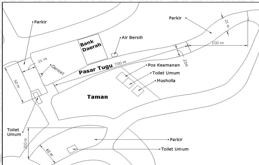
Gambar 4. 3 Site Plan Pasar Tugu Simpang Lima Gumul Kabupaten Kediri
