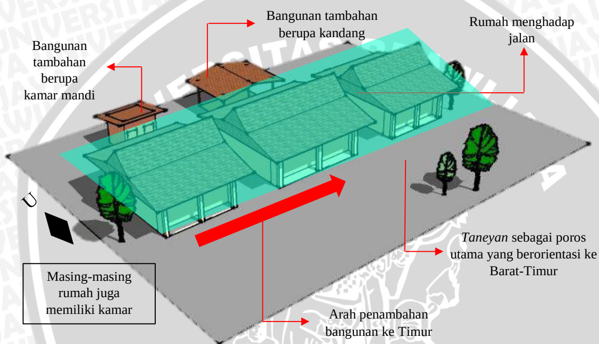
Gambar 4.27 : Perspektif tata letak rumah tradisional Madura X
