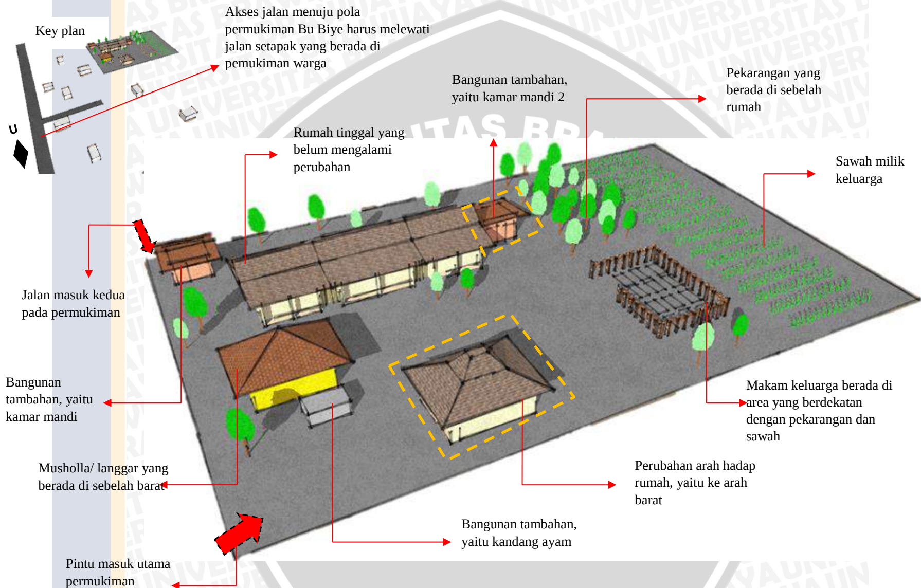
Gambar 4.75: Perspektif perubahan tata letak pada rumah tradisional Madura Bu Biye
