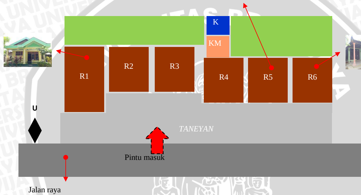
Gambar 4.320: Perubahan bangunan pada rumah tradisional Madura Bu Sumyani
