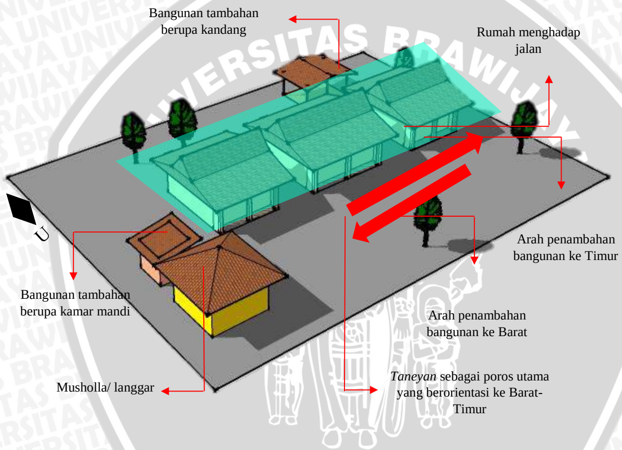
Gambar 4.22 : Perspektif tata letak rumah tradisional Madura V
