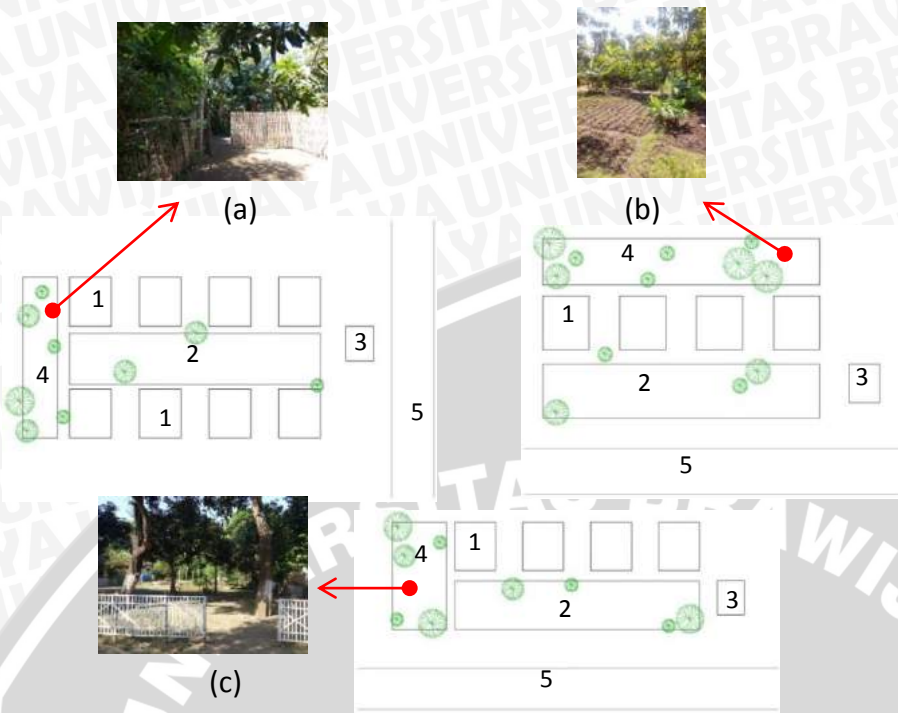
Gambar 4.32 : Letak pekarangan/ tegalan rumah tradisional Madura di Desa Mangaran
