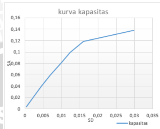
Gambar 9. Kurva Spektrum Kapasitas
