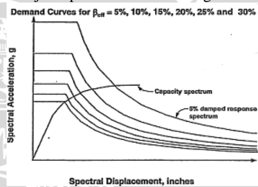
Gambar 2. Spektrum kapasitas Prosedur B
