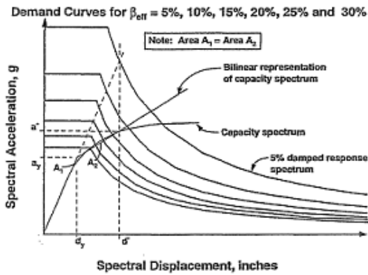
Gambar 3. Spektrum kapasitas Prosedur B setelah step 4.
