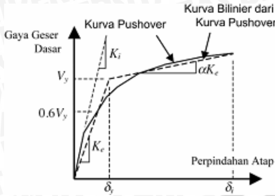
Gambar 4. Waktu getar alami efektif dari kurva pushover .
