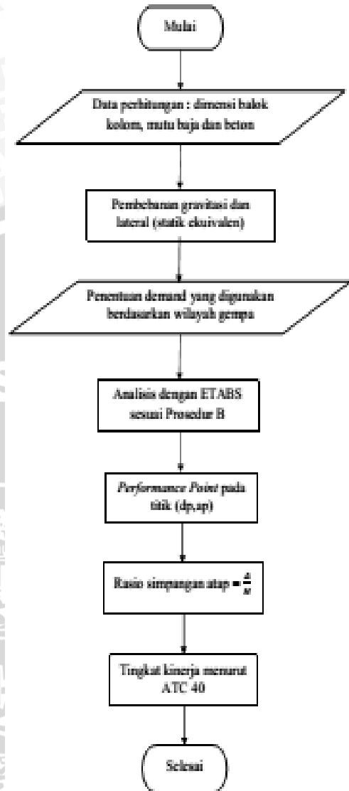
Gambar 5. Flowchart analisis struktur.
