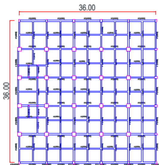
Gambar 7. Denah bangunan.
