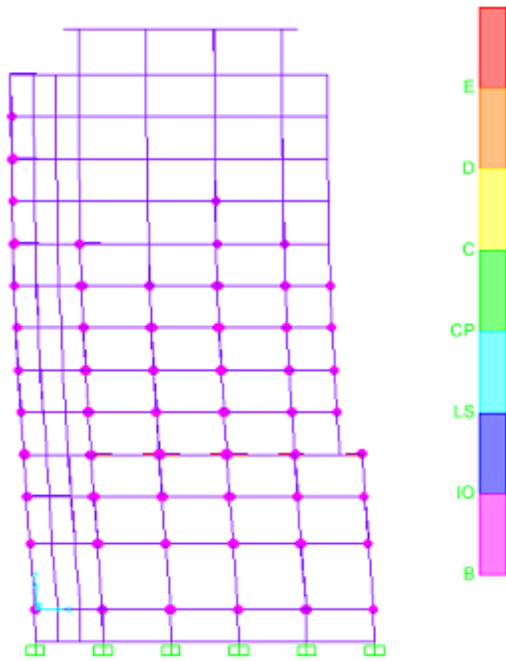
Gambar 12. Letak sendi plastis pada pembebanan step 3
