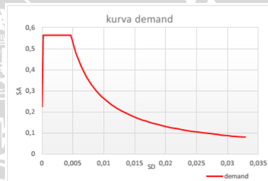
Gambar 10. Kurva Respon Spektrum Format ADRS.
