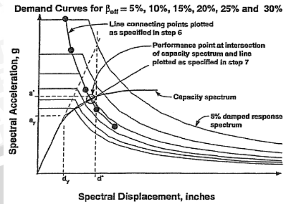
Gambar 4. Spektrum kapasitas Prosedur B setelah step 7.
