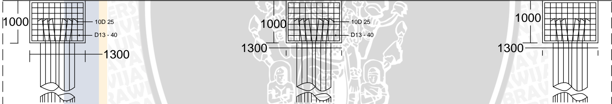
DETAIL PENULANGAN KEPALA TIANG SKALA 1 : 192
