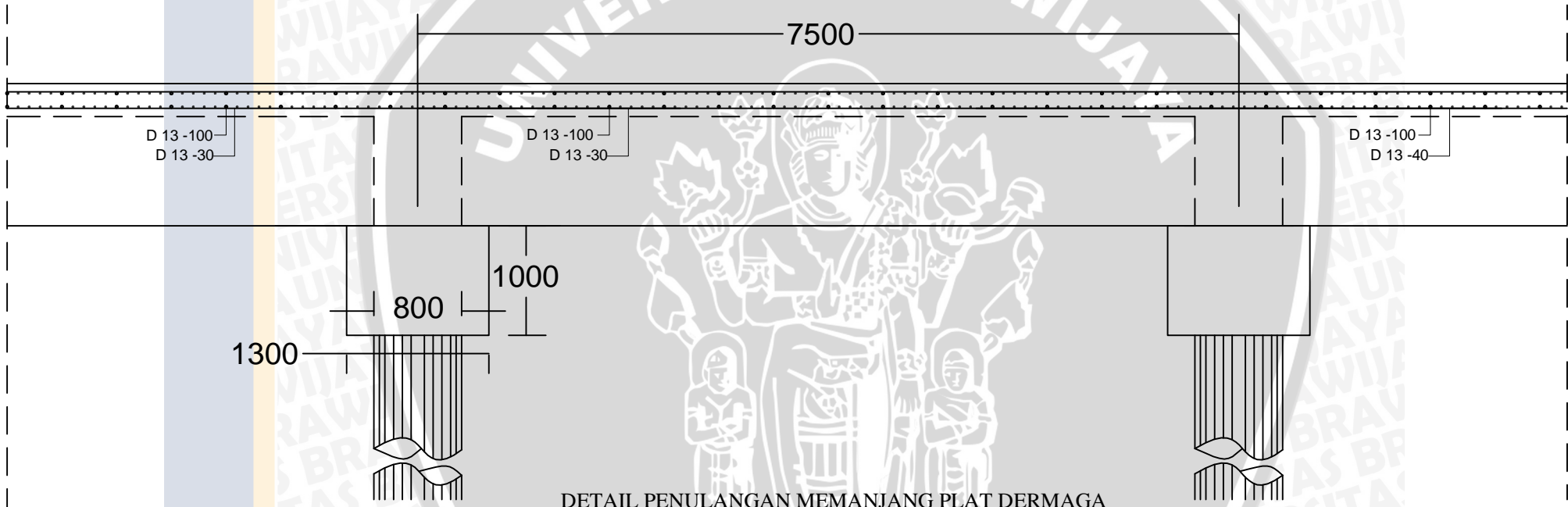
DETAIL PENULANGAN MEMANJANG PLAT DERMAGA SKALA 1 : 192
