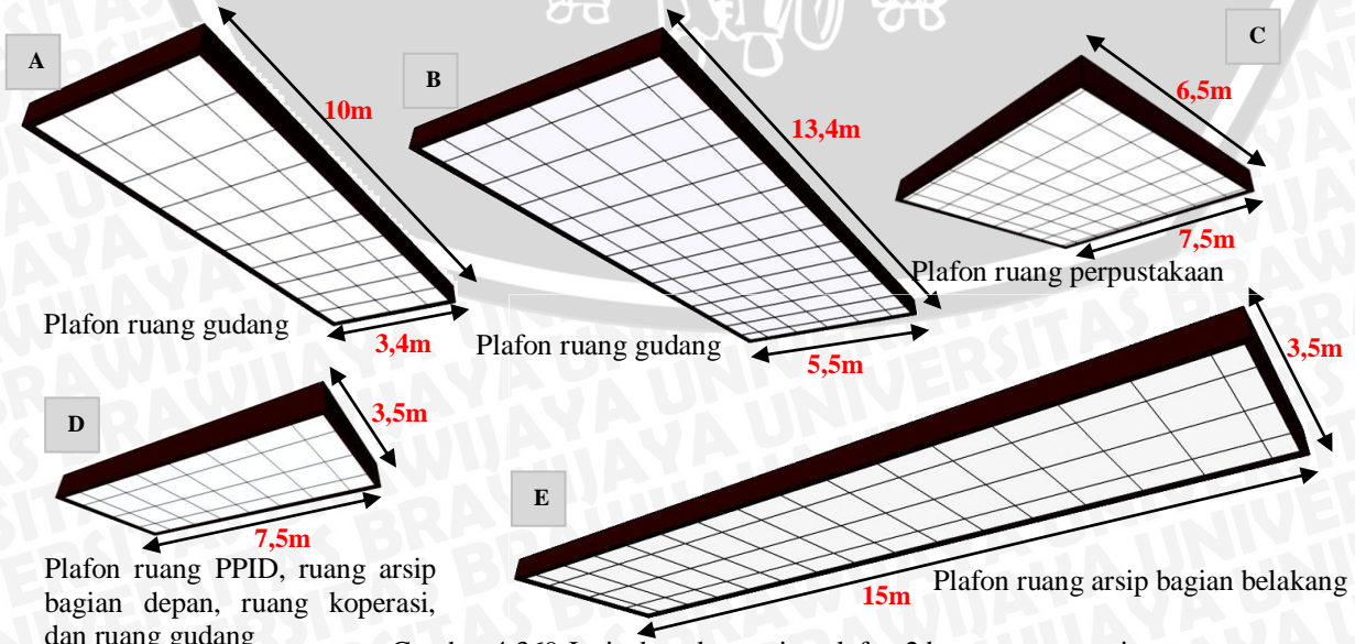
Gambar 4.369 Jenis dan ukuran tipe plafon 2 bangunan penunjang Kantor Bakorwil IV Jatim Pamekasan
