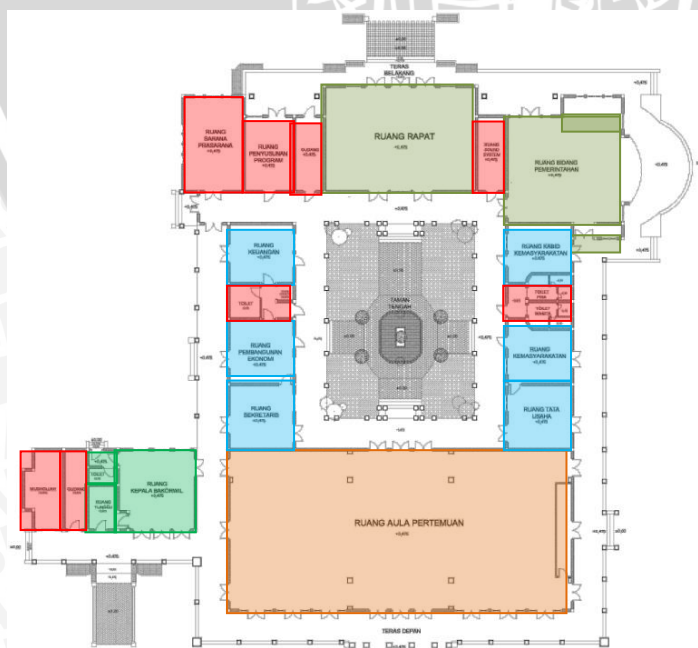
Gambar 4.346 Jenis-jenis dan letak plafon bangunan induk Kantor Bakorwil IV Jatim Pamekasan
