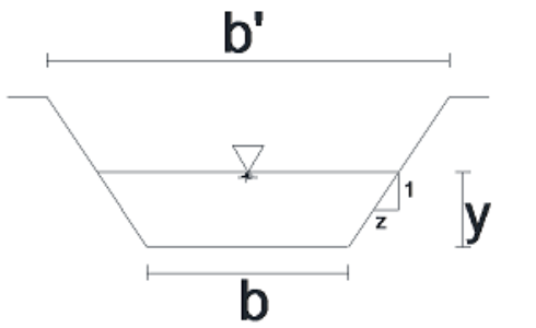
Gambar 1. Penampang saluran trapesium.
