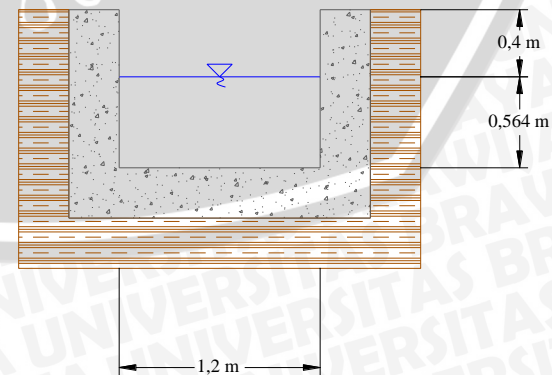
Gambar 6. Dimensi Floodway F2.
