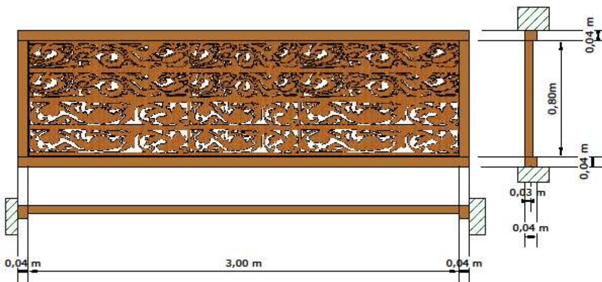
detil v10 front pool villa skala 1:20
