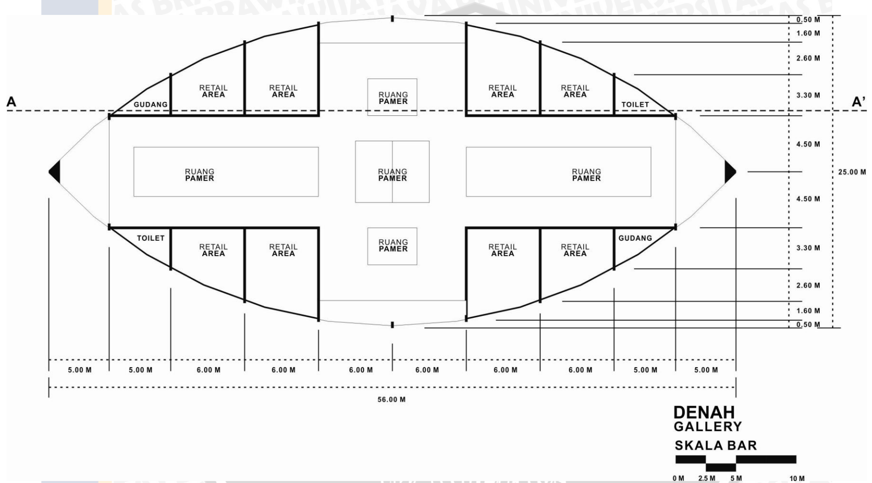
Lampiran 21 Denah bangunan galeri
