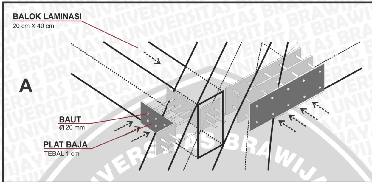
Lampiran 19 Detail A kantor pengelola
