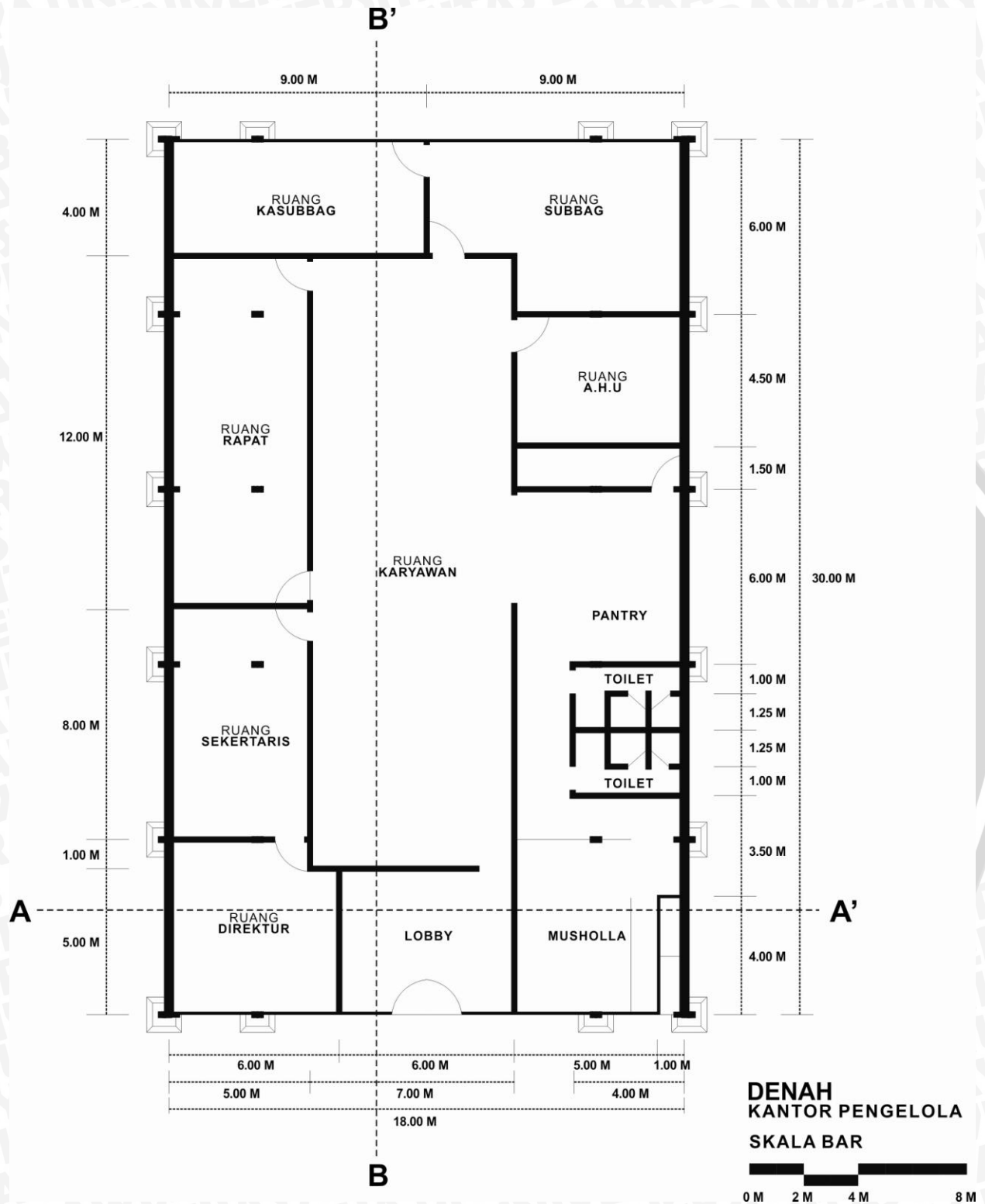
Lampiran 15 Denah Kantor Pengelola
