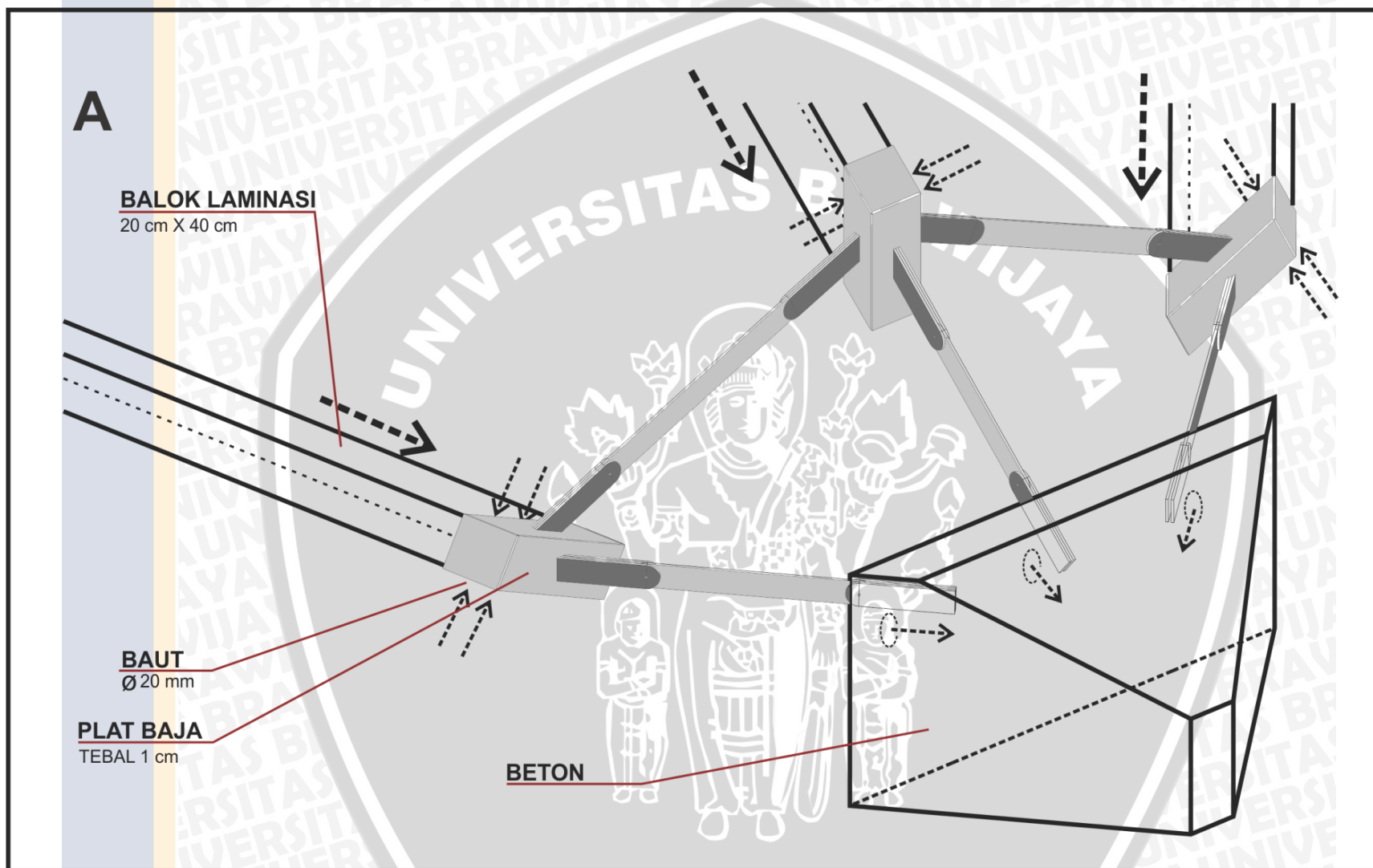
Lampiran 24 Detail A bangunan galeri
