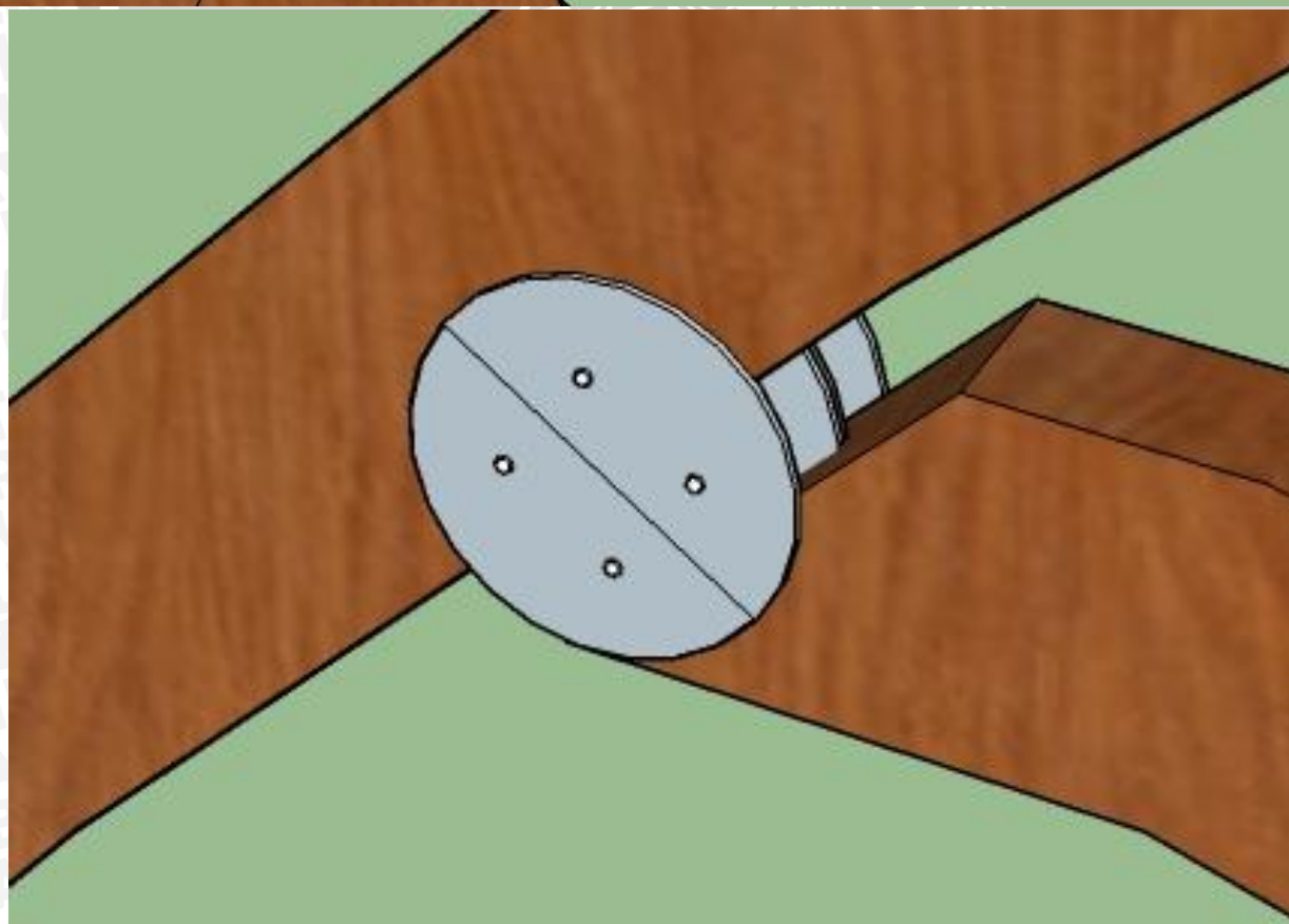
Lampiran 2 Sambungan antar rangka pada bangunan
