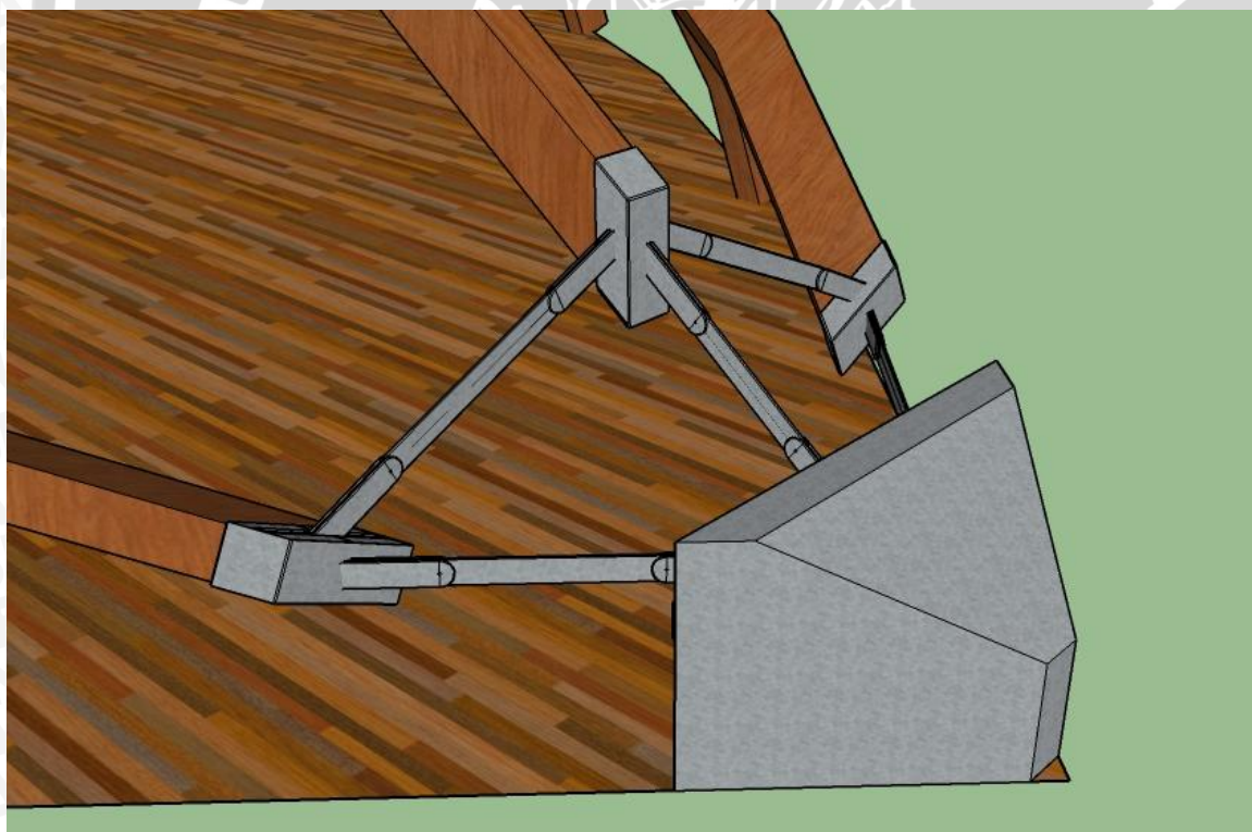
Lampiran 7 Sambungan kolom laminasi dengan balok cor
