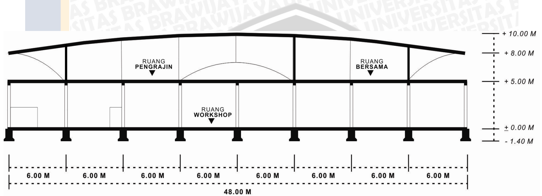
POTONGAN BANGUNAN WORKSHOP
