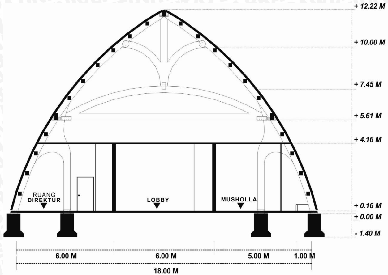
POTONGAN A-A'
