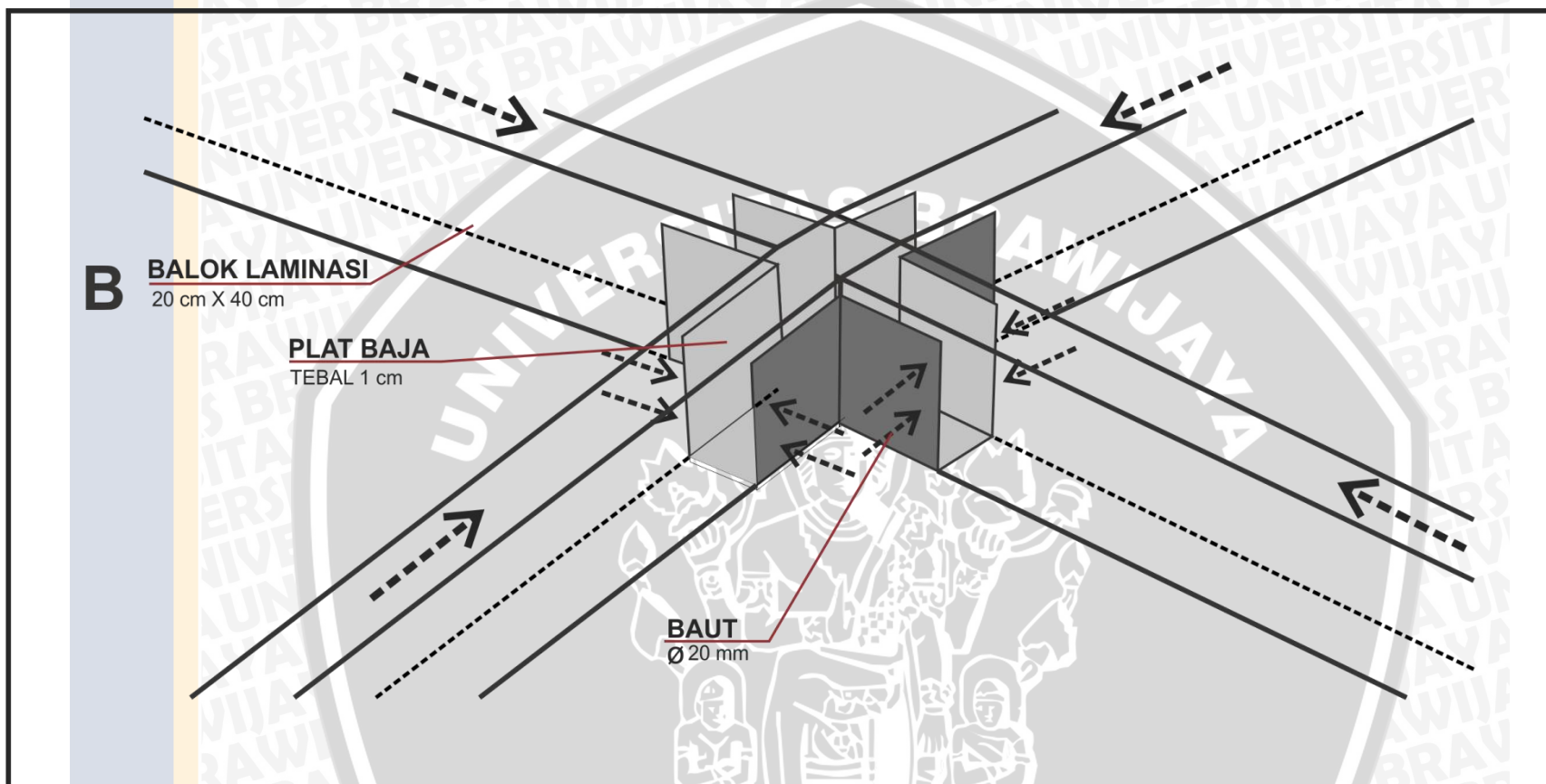
Lampiran 25 Detail B bangunan galer
