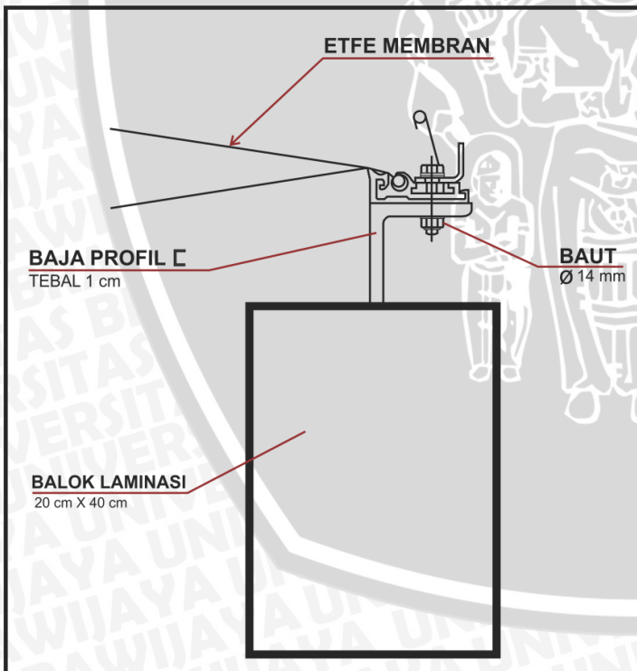
Lampiran 39 Detail Selubung membran
