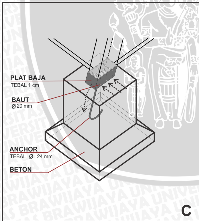
Lampiranrr 46 Detail Sambungan C bangunan Workshop
