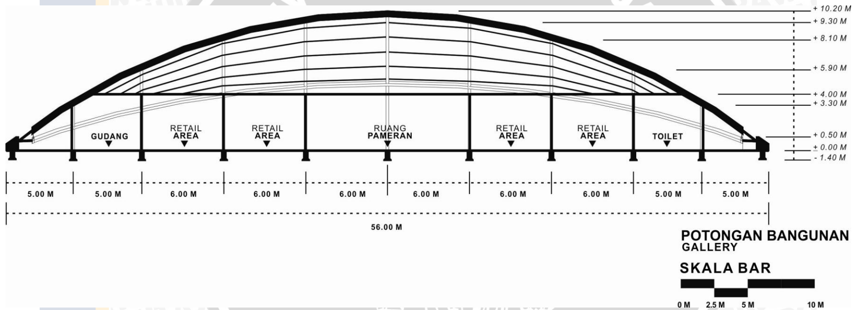
Lampiran 22 Potongan bangunan galeri
