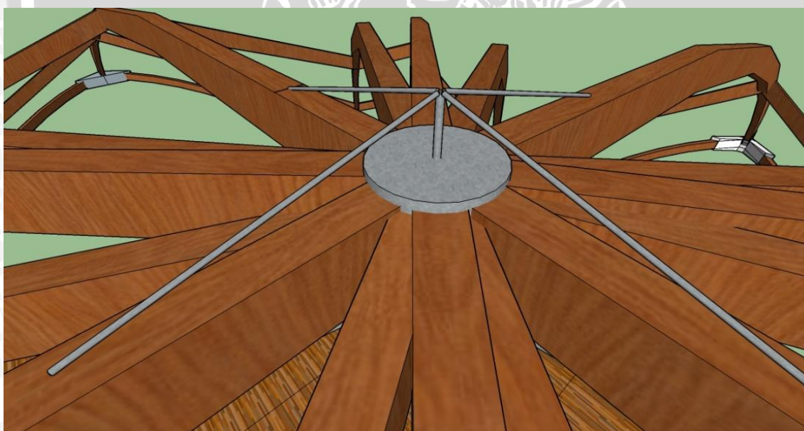
Lampiran 5 Struktur kabel pada rangka atap bangunan penerima
