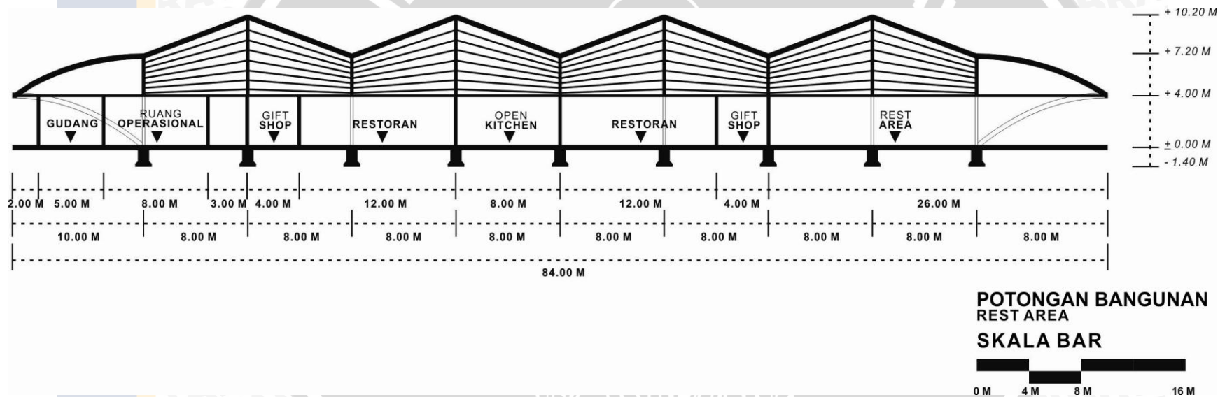
Lampiran 28 Potongan Bangunan Rest Area
