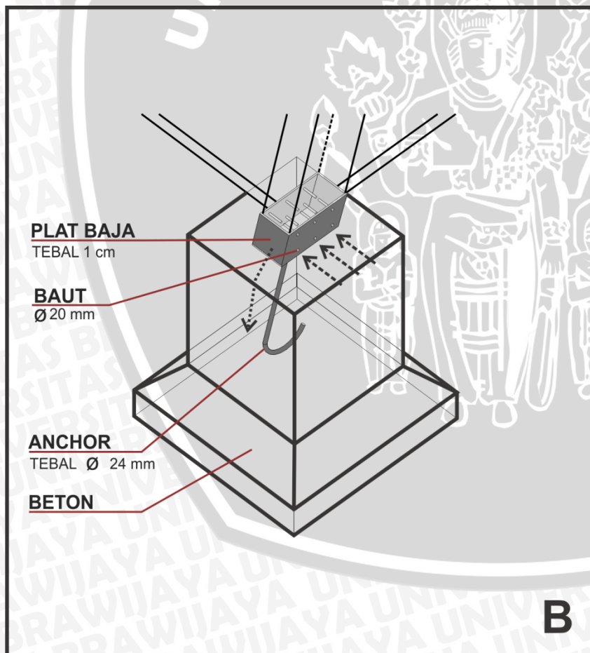
Lampiran 20 Detail B kantor pengelola
