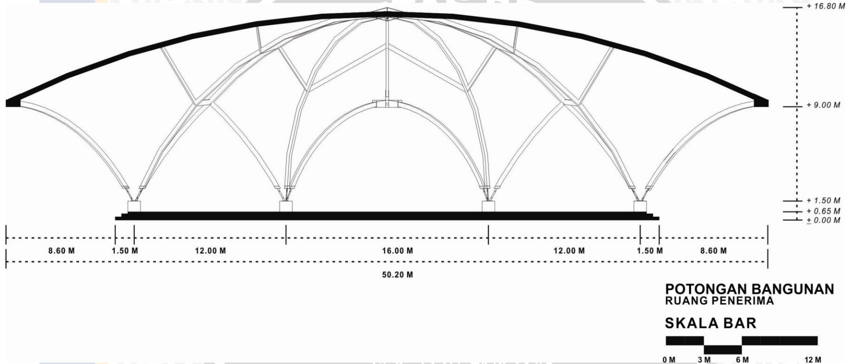
Lampiran 34 Potongan Bangunan ruang penerima
