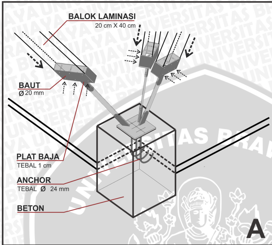
Lampiran 36 Detal Sambungan A Ruang Penerima
