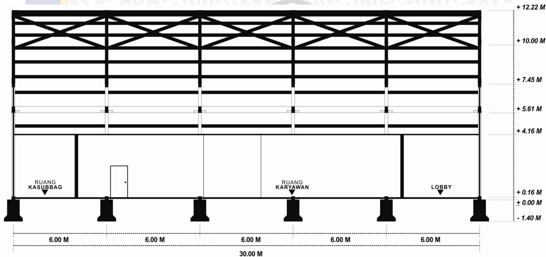
POTONGAN B-B'
