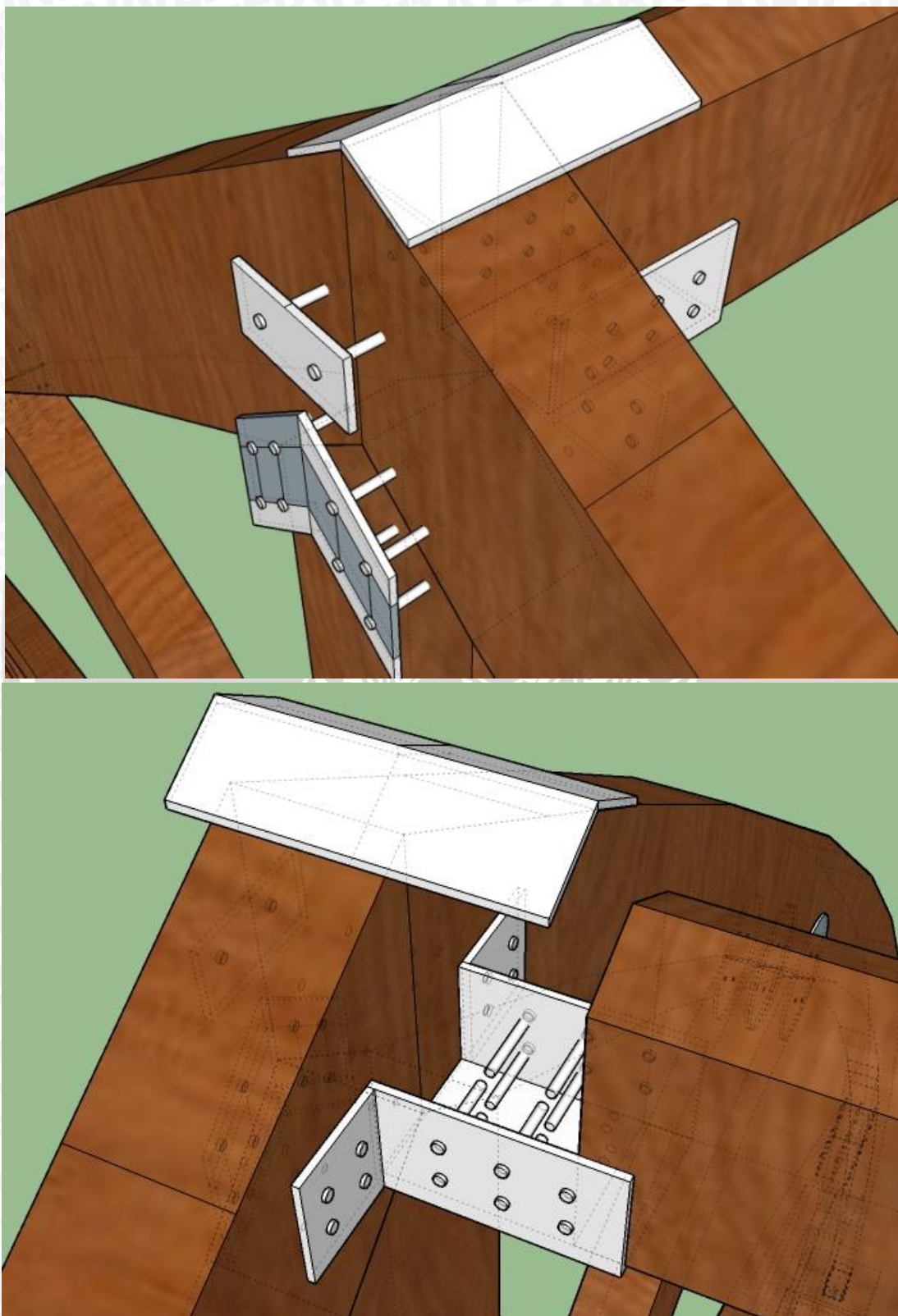
Lampiran 3 Sambungan pada struktur atap
