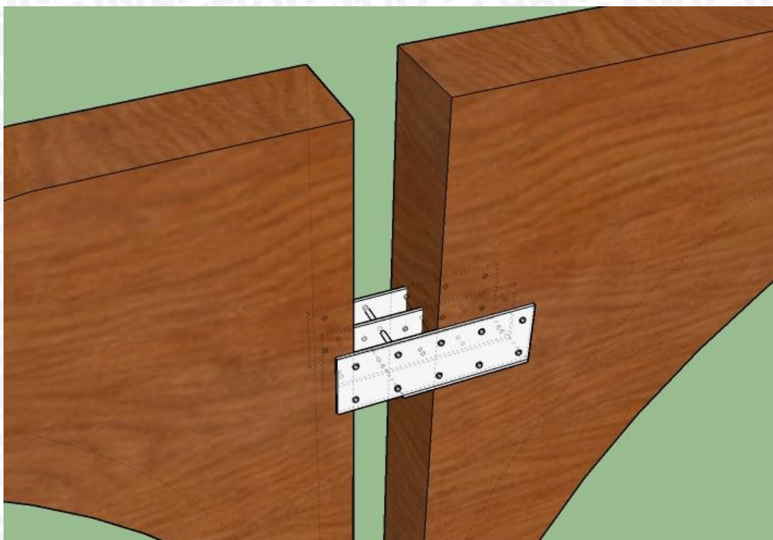
Lampiran 4 Sambungan rangka kolom dengan balok
