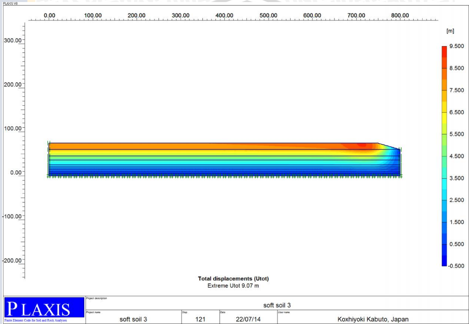
Gambar 4.35 Keluaran total displacements untuk bore hole 3 (Plaxis 8.2 2D) Sumber : Hasil Perhitungan, 2014
