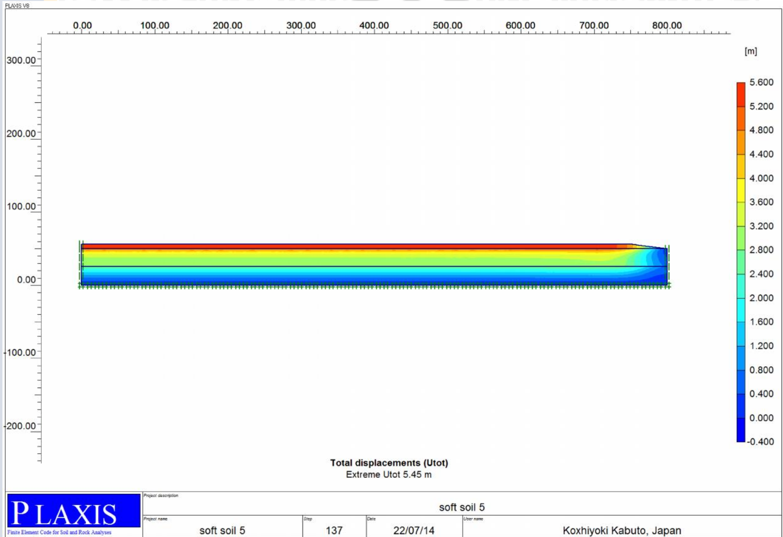
Gambar 4.37 Keluaran total displacements untuk bore hole 5 (Plaxis 8.2 2D) Sumber : Hasil Perhitungan, 2014
