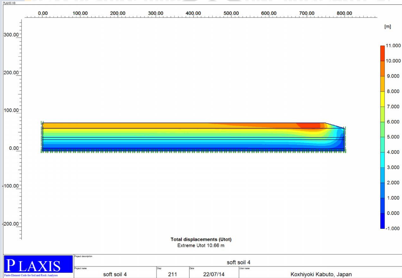
Gambar 4.36 Keluaran total displacements untuk bore hole 4 (Plaxis 8.2 2D)
