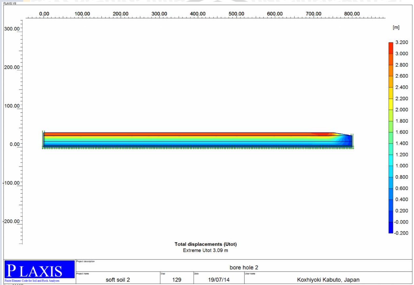
Gambar 4.34 Keluaran total displacements untuk bore hole 2 (Plaxis 8.2 2D) Sumber : Hasil Perhitungan, 2014
