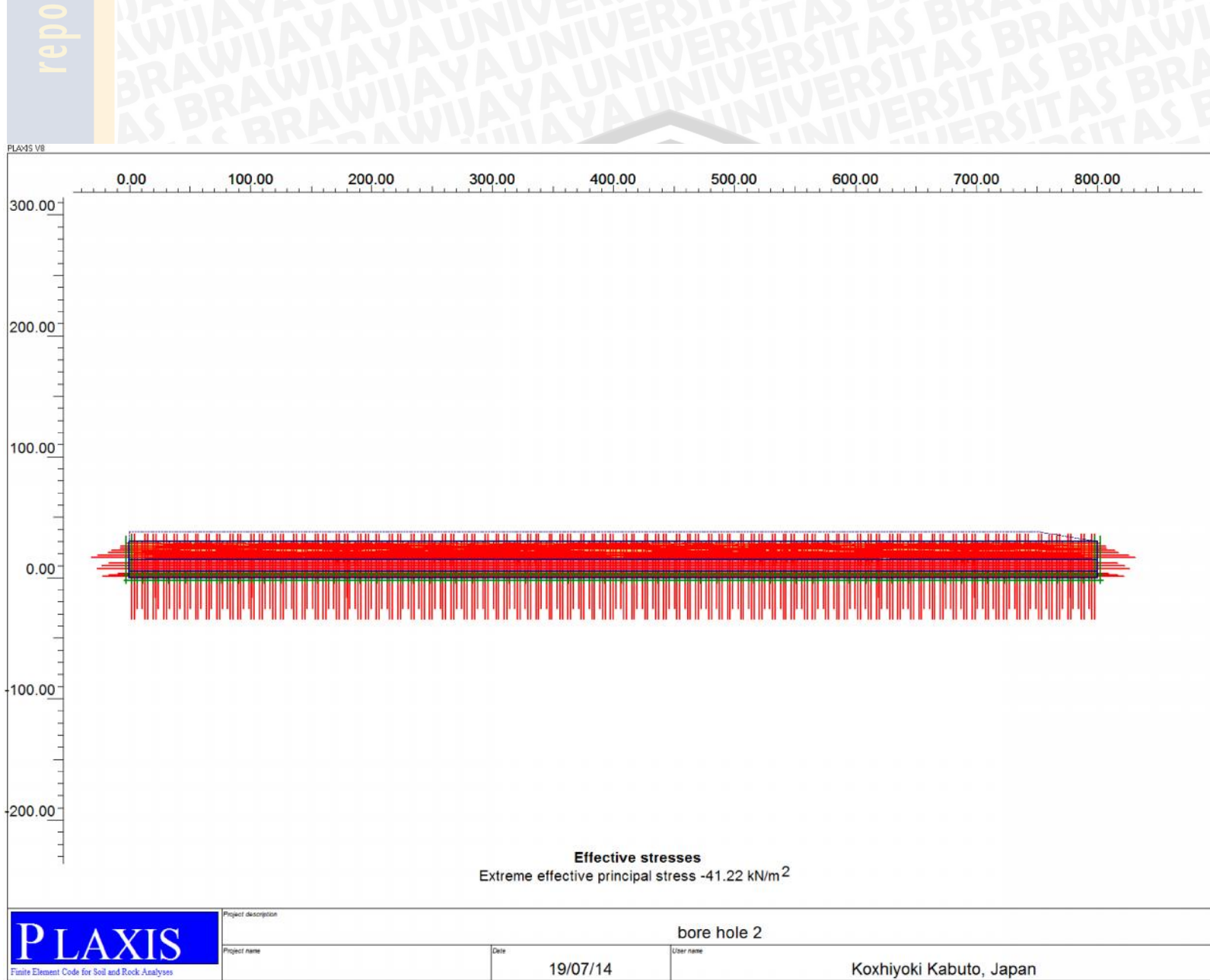
Gambar 4.31 Penggambaran tegangan awal ( Initial Stresses ) untuk bore hole 2 (Plaxis 8.2 2D) Sumber : Hasil Perhitungan, 2014
