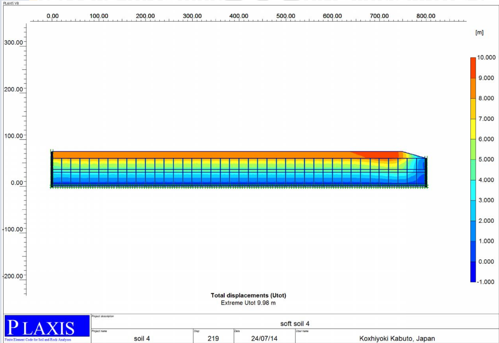
Gambar 4.54 Keluaran total displacements untuk bore hole 4 dengan pemasangan PVD (Plaxis 8.2 2D) Sumber : Hasil Perhitungan, 2014
