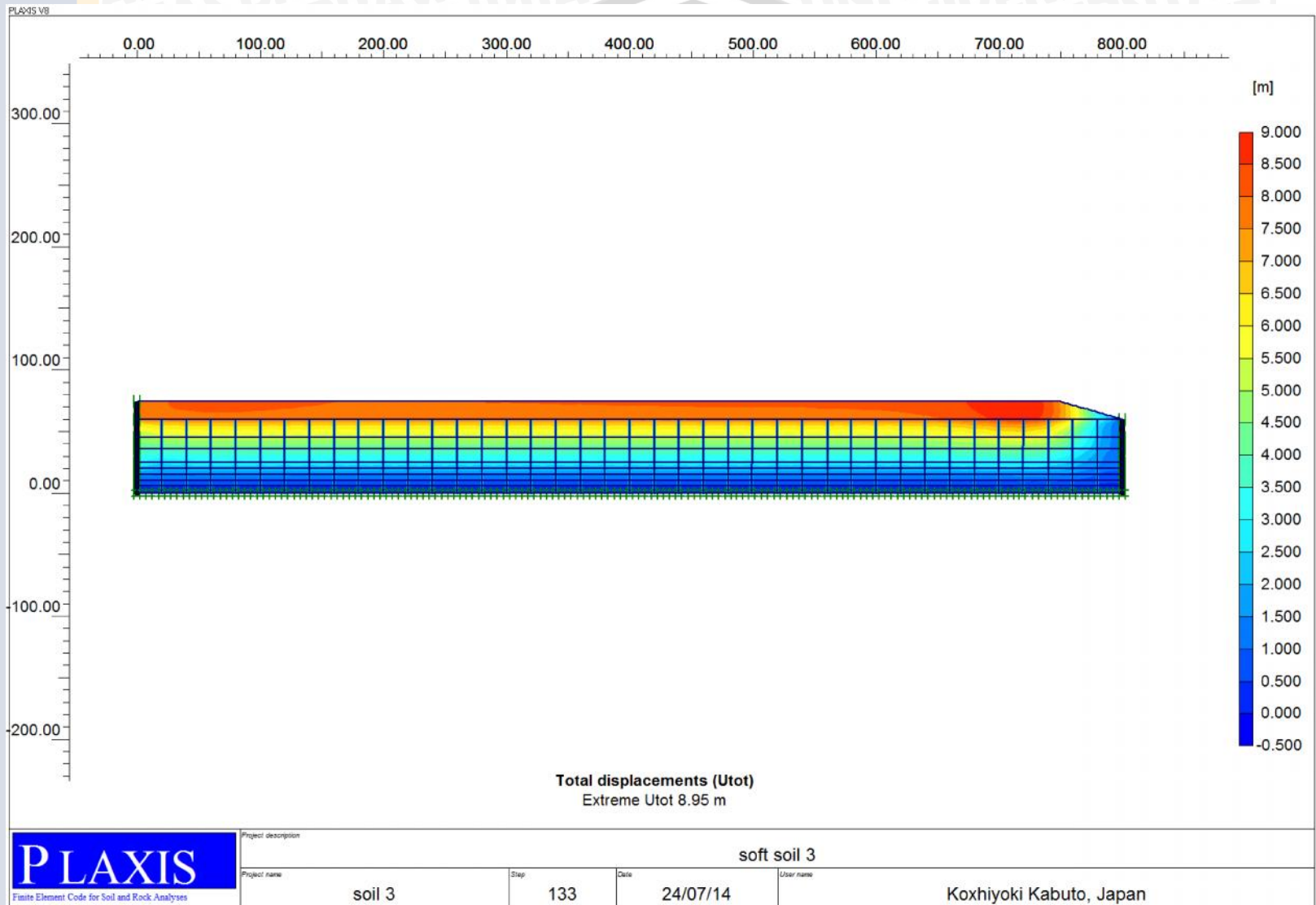
Gambar 4.53 Keluaran total displacements untuk bore hole 3 dengan pemasangan PVD (Plaxis 8.2 2D) Sumber : Hasil Perhitungan, 2014
