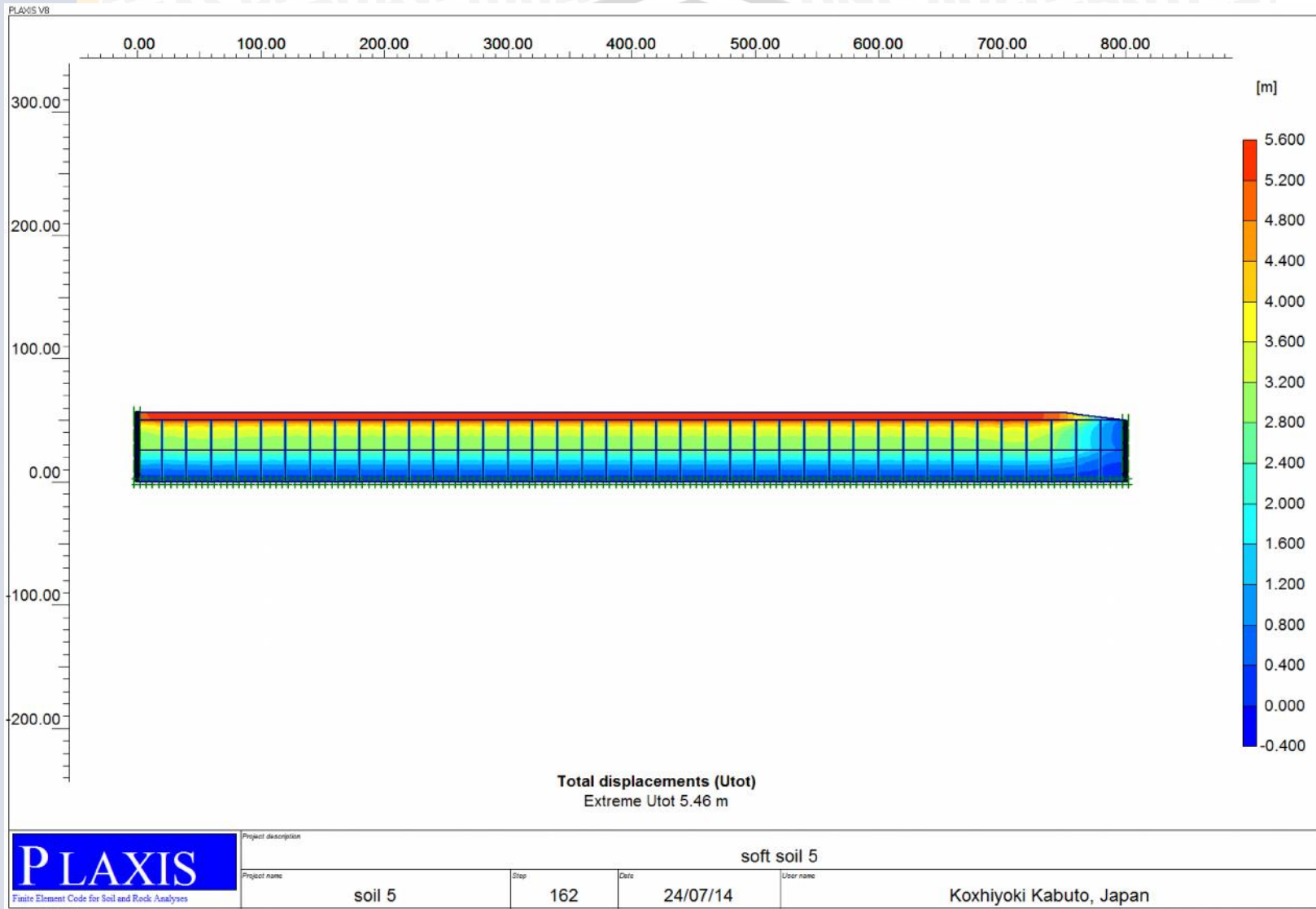
Gambar 4.55 Keluaran total displacements untuk bore hole 5 dengan pemasangan PVD (Plaxis 8.2 2D) Sumber : Hasil Perhitungan, 2014
