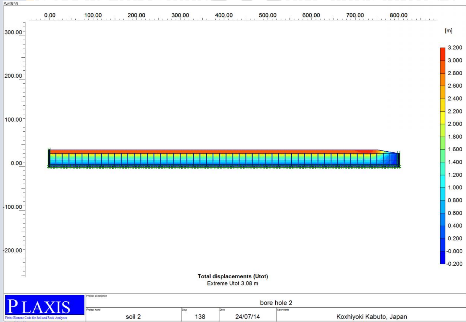
Gambar 4.52 Keluaran total displacements untuk bore hole 2 dengan pemasangan PVD (Plaxis 8.2 2D) Sumber : Hasil Perhitungan, 2014
