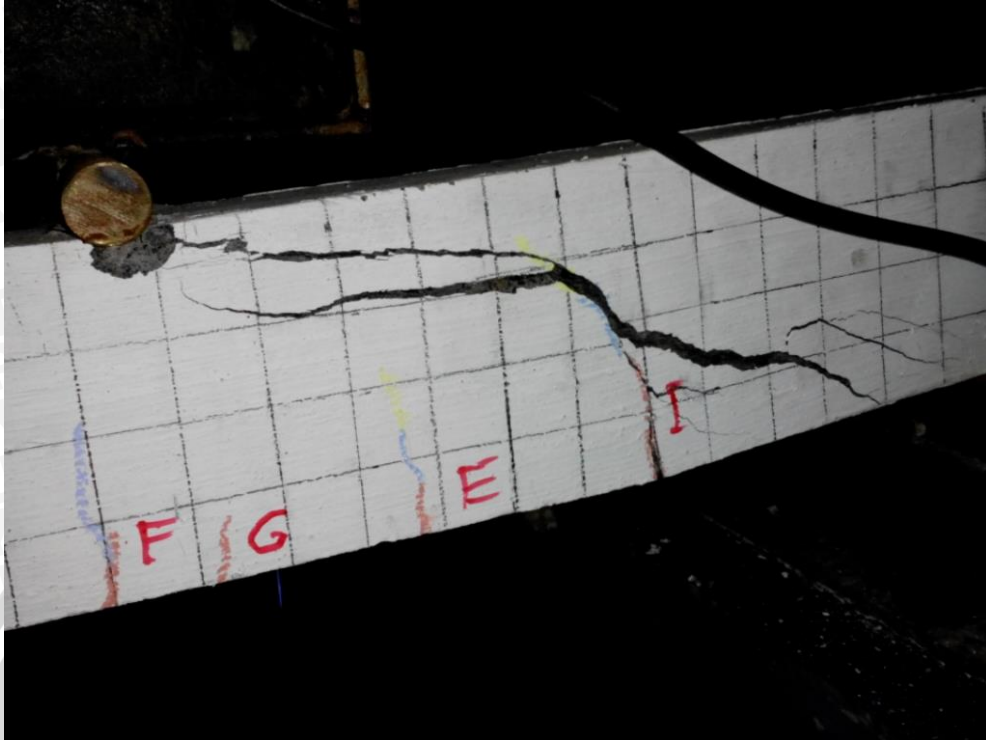
Gambar keruntuhan geser pada balok (20% bottom ash)
