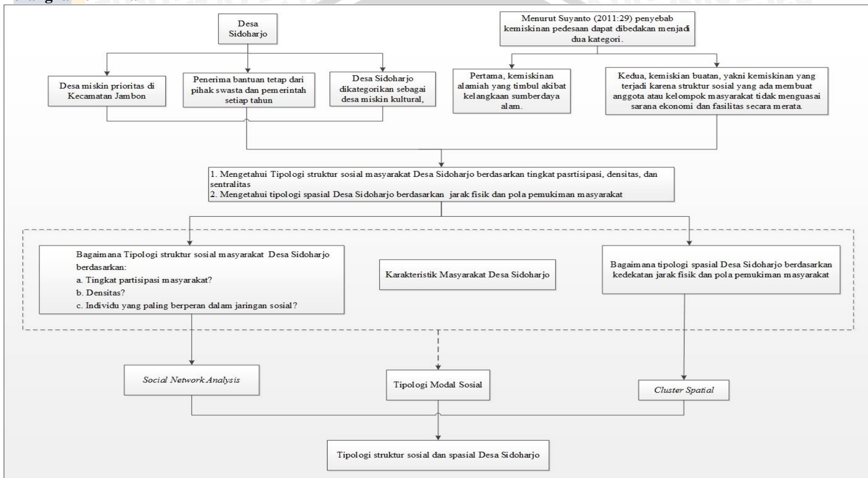
Gambar 1. 3 Diagram Alir
