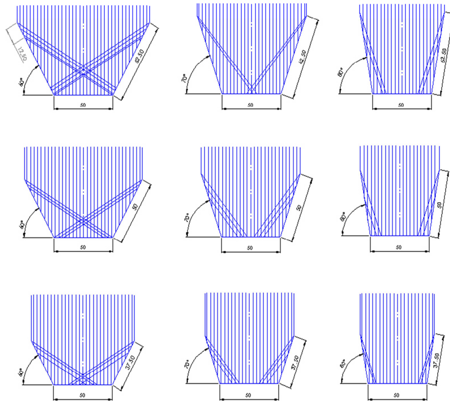
Gambar 3.8 Variasi sudut cermin dan ratio lebar cermin dengan photovoltaic
