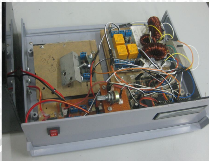
Gambar. 3 Board Keseluruhan
