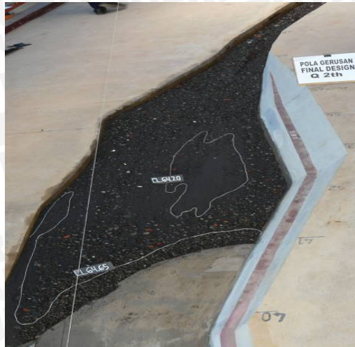
Foto 1. Pola gerusan Q_{2th} tanpa perlindungan sungai
