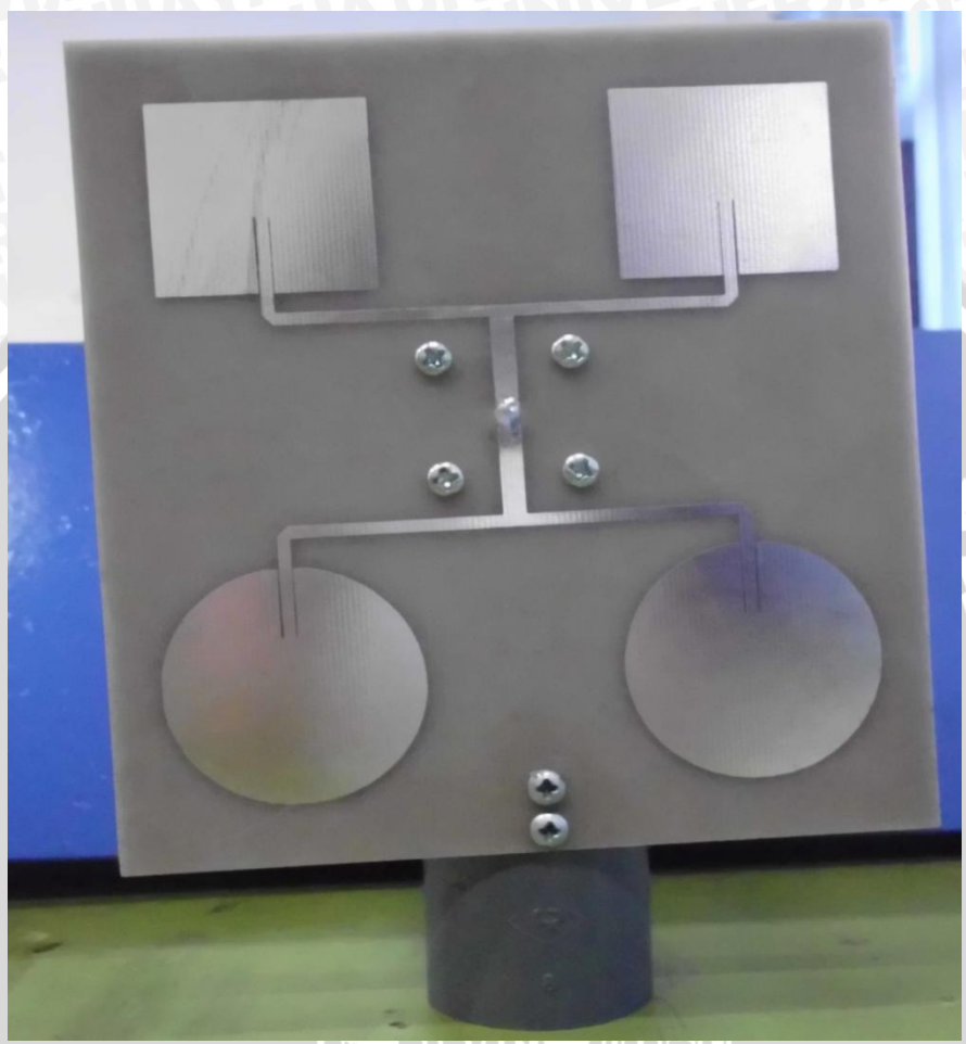
Gambar 1 Antena Mikrostrip Kotak-Lingkar Patch Array Empat Elemen
