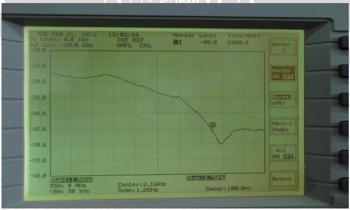
Gambar 5 Hasil Pengukuran Return Loss Antena Uji
