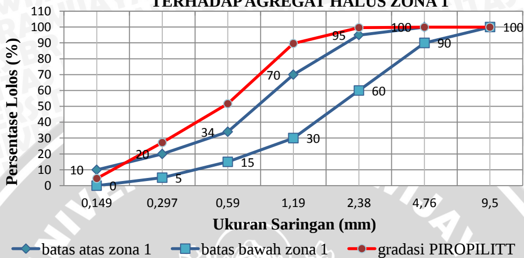
GRAFIK LENGKUNG PIROPILIT TERHADAP AGREGAT HALUS ZONA 1
