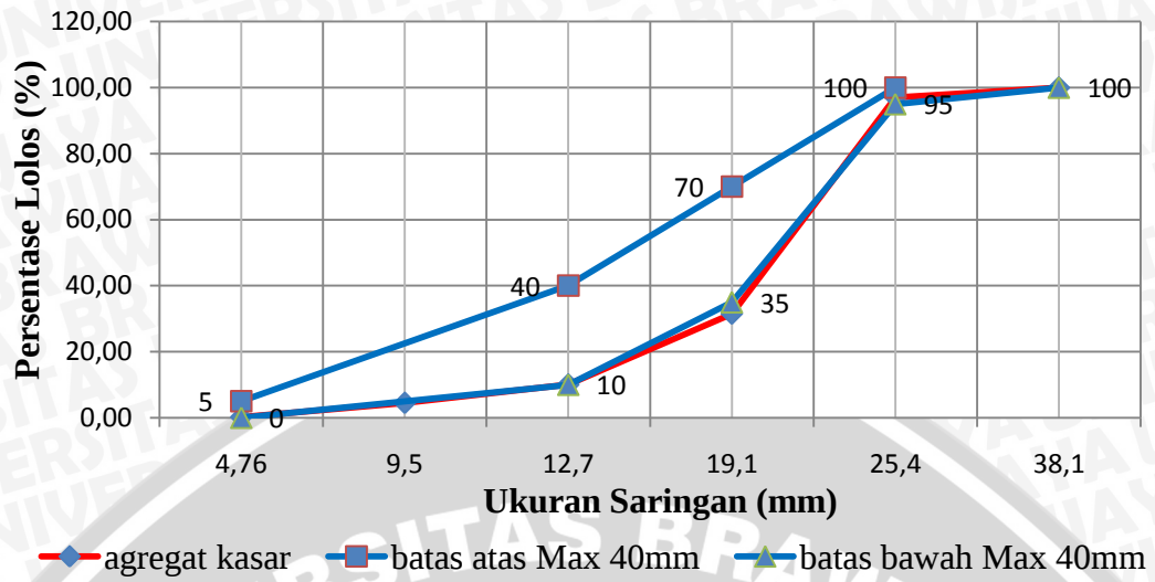
GRAFIK LENGKUNG AGREGAT KASAR Max 40mm
