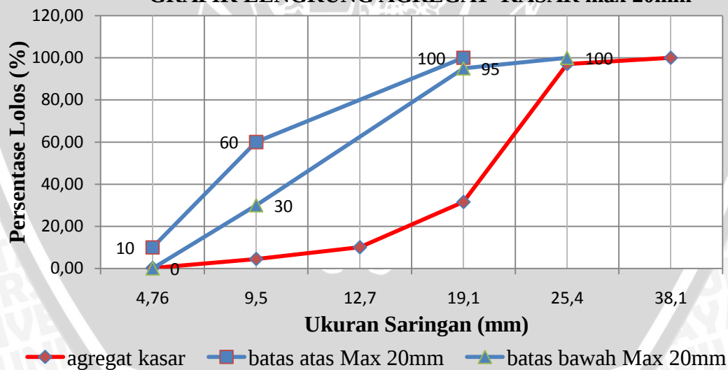
GRAFIK LENGKUNG AGREGAT KASAR max 20mm
