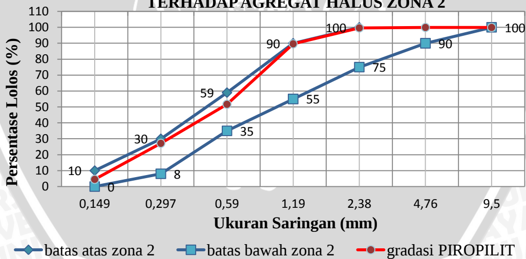
GRAFIK LENGKUNG PIROPILIT TERHADAP AGREGAT HALUS ZONA 2
