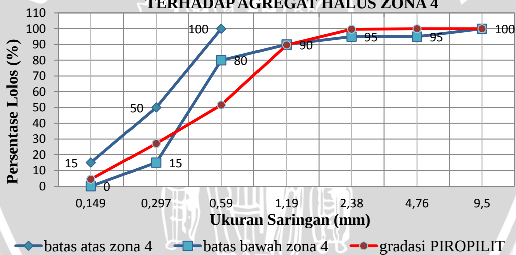
GRAFIK LENGKUNG PIROPILIT TERHADAP AGREGAT HALUS ZONA 4
