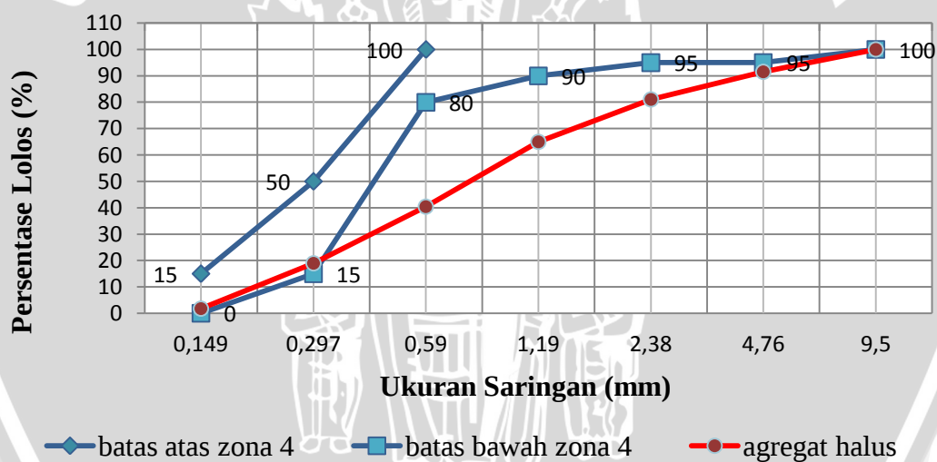
GRAFIK LENGKUNG AGREGAT HALUS ZONA 4
