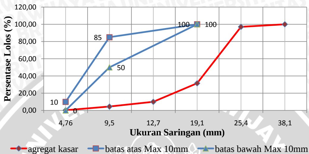
GRAFIK LENGKUNG AGREGAT KASAR Max 10mm
