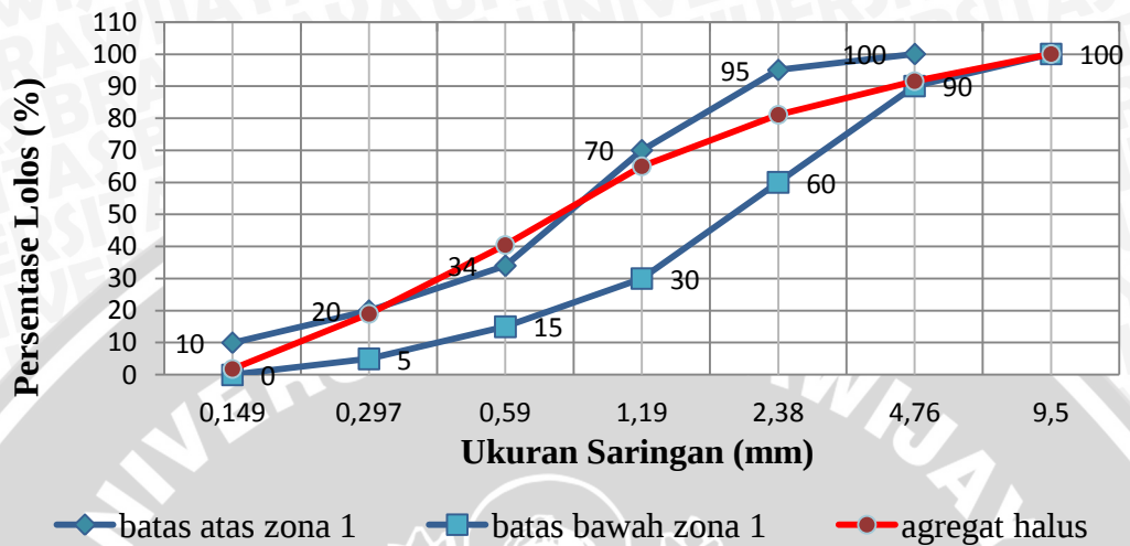
GRAFIK LENGKUNG AGREGAT HALUS ZONA 1
