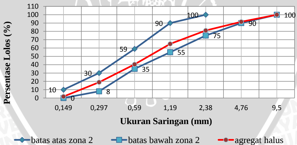
GRAFIK LENGKUNG AGREGAT HALUS ZONA 2
