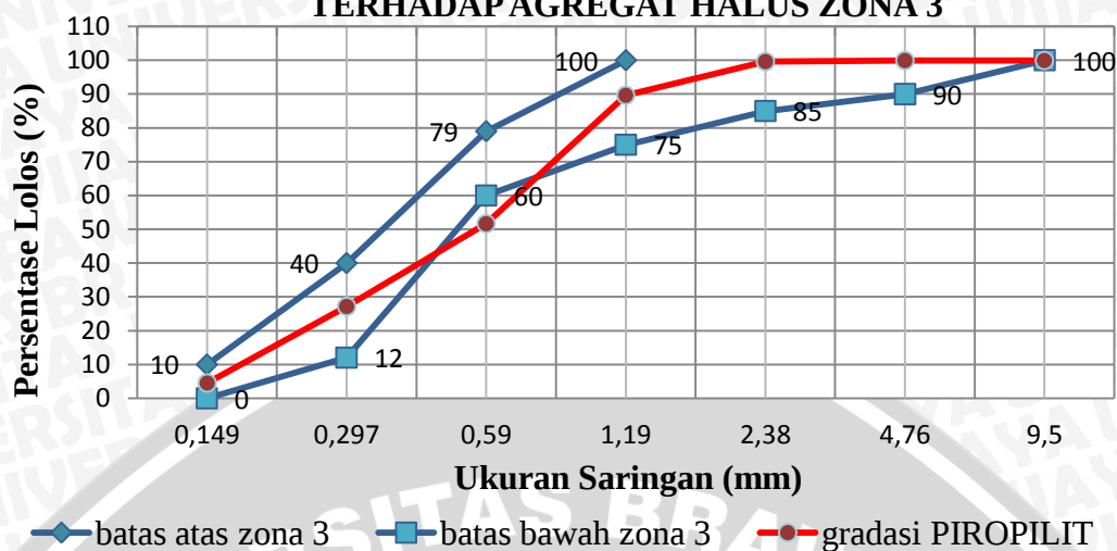
GRAFIK LENGKUNG PIROPILIT TERHADAP AGREGAT HALUS ZONA 3
